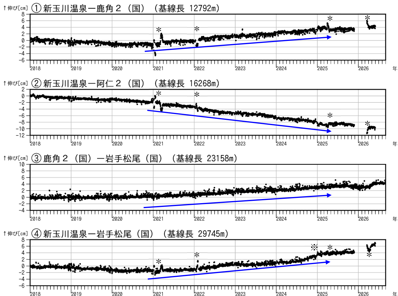
図4 秋田焼山 GNSS 基線長変化図（2018年1月～2026年8月）
