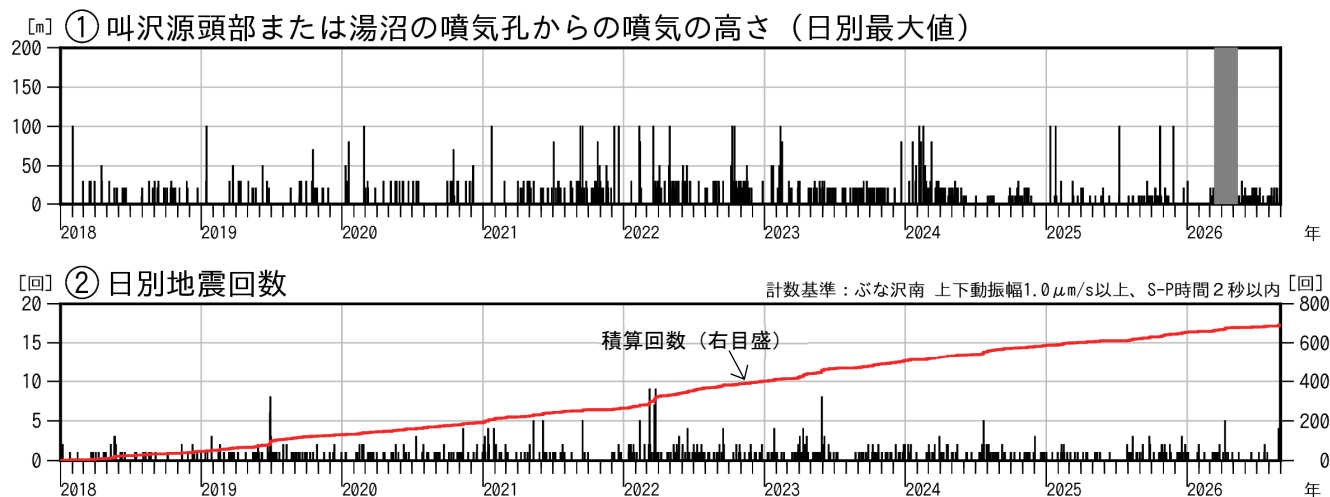
図3 秋田焼山 火山活動経過図（2018年1月～2026年8月）
