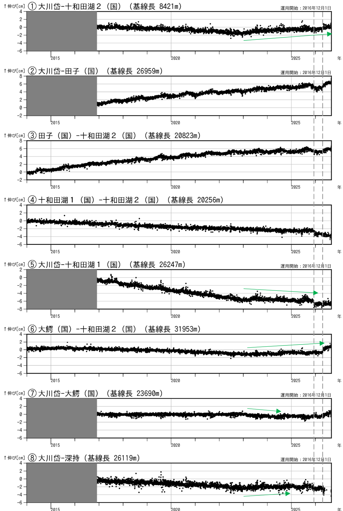
図 4 十和田 GNSS 基線長変化図（2014 年 1 月～2026 年 8 月）
