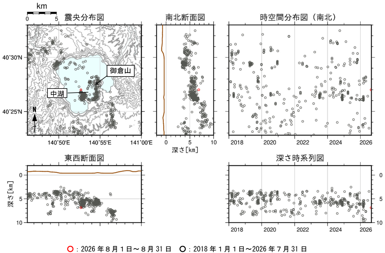
図3 十和田 地震活動（2018年1月～2026年8月）
