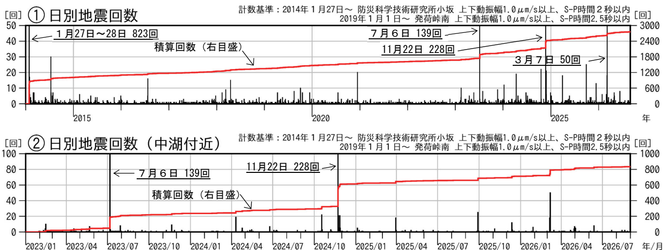
図2 十和田 活動経過図（2014年1月～2026年8月）
