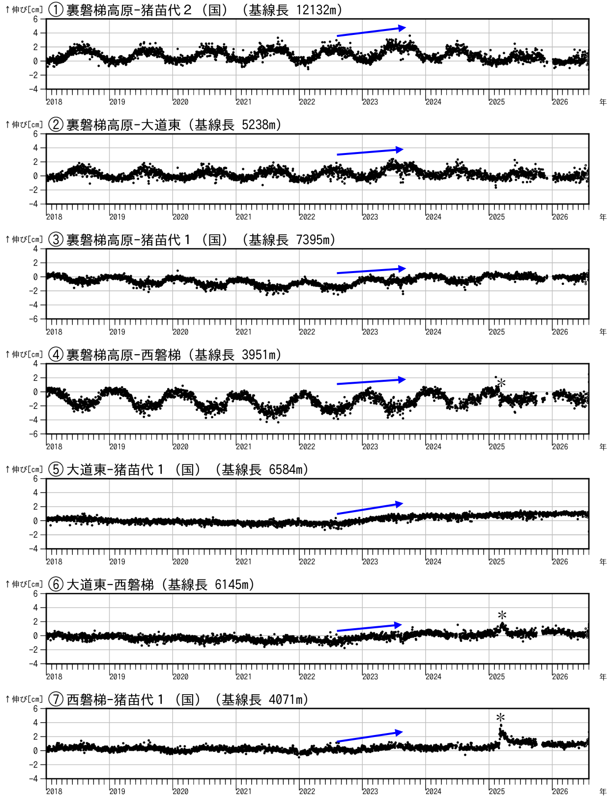
図6 磐梯山 GNSS基線長変化図（2018年1月～2026年7月）
