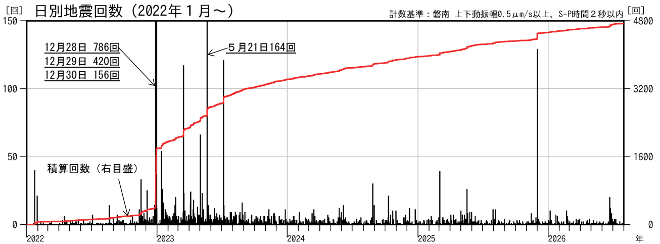
図4 磐梯山 地震回数（2022年1月～2026年7月）
