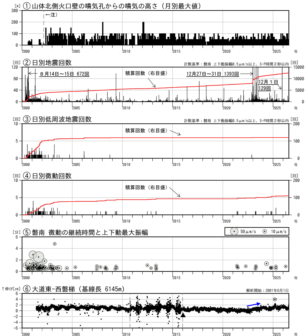
図3 磐梯山 火山活動経過図（2000年1月～2026年7月）
