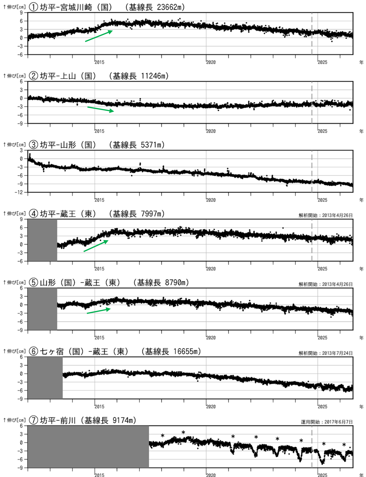
図3 蔵王山 GNSS 基線長変化図（2012年1月～2026年7月）
