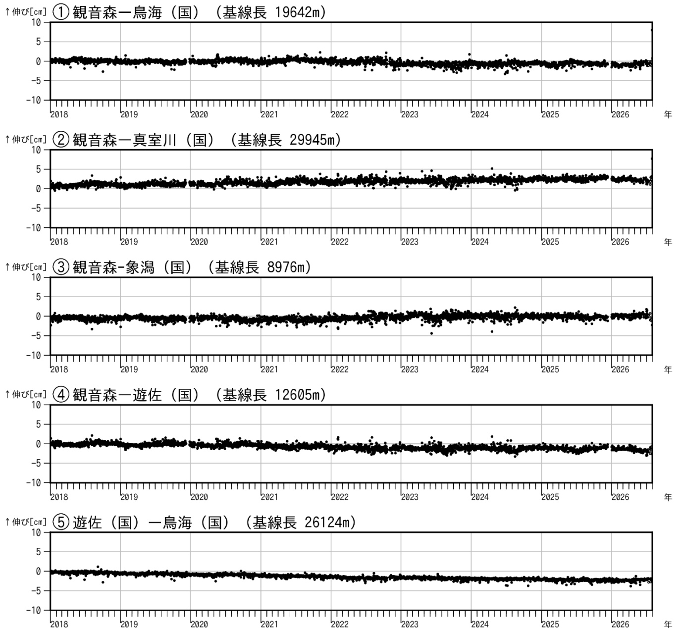
図4 鳥海山 GNSS 基線長変化図（2018年1月～2026年7月）
