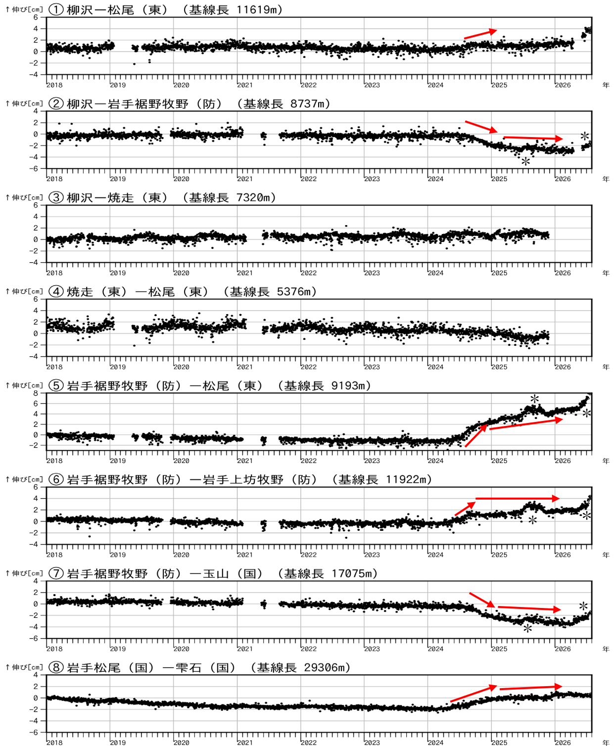
図7 岩手山 GNSS 基線長変化図（2018年1月～2026年7月）
