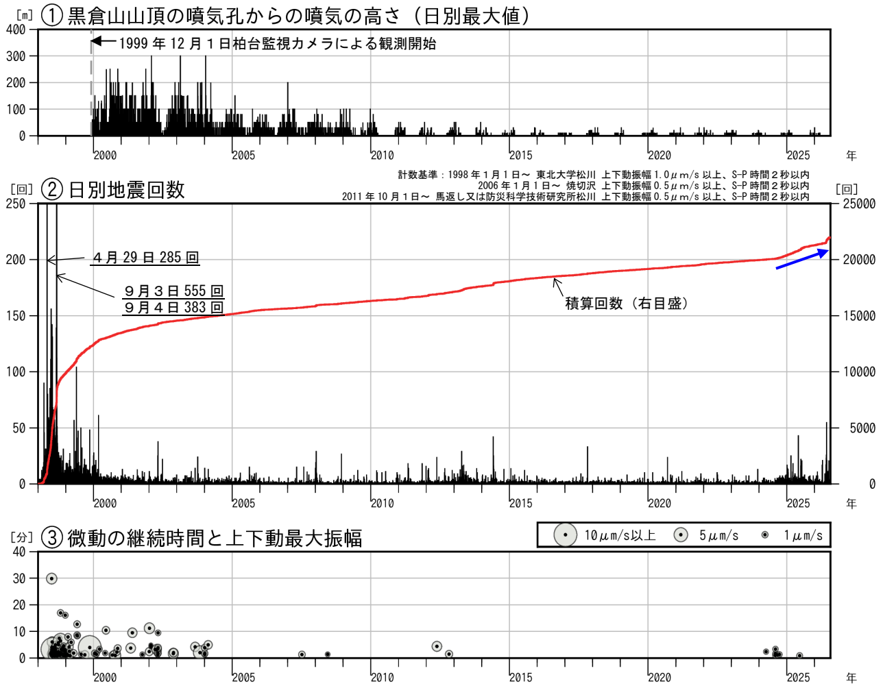
図1 岩手山 火山活動経過図（1998年1月～2026年7月）
