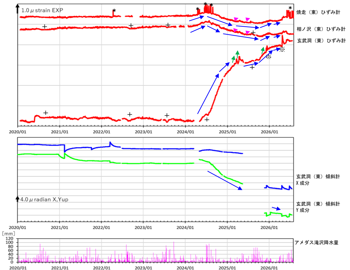
図8 岩手山 ひずみ計・傾斜計（日値・トレンド補正済み）による地殻変動の状況 （2020年1月～2026年7月）
