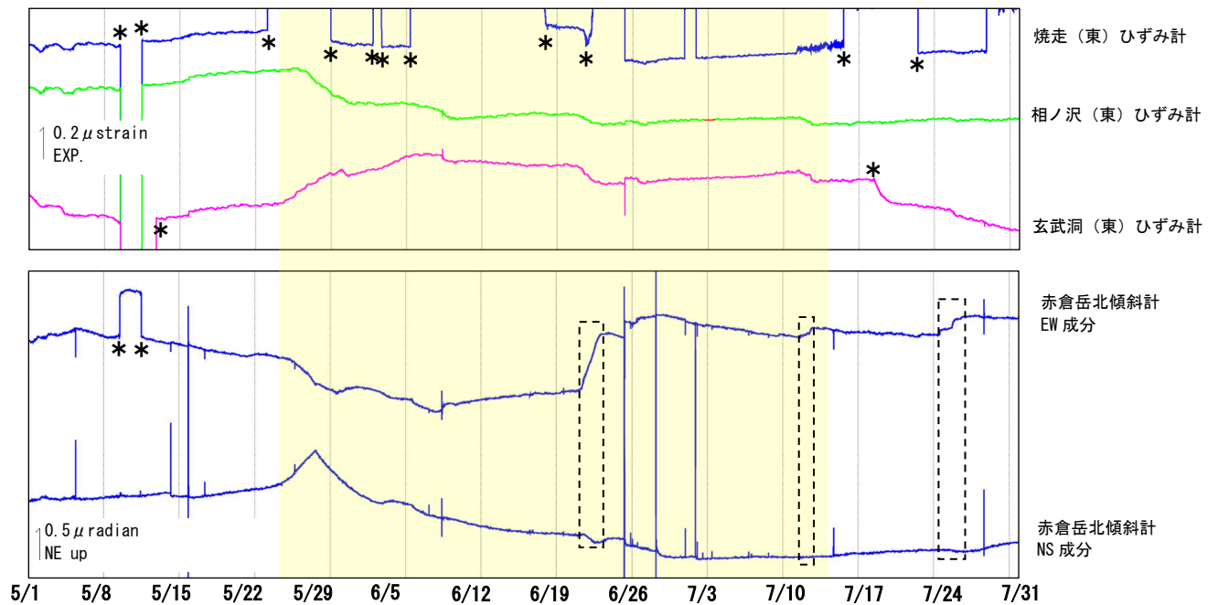
図9 岩手山 ひずみ計・傾斜計（分値・トレンド補正済み）による地殻変動の状況 （2026年5月1日～7月31日）
