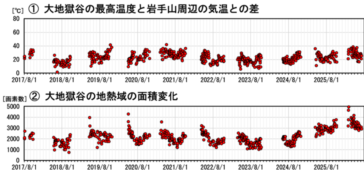
図 5－2 岩手山 黒倉山監視カメラによる大地獄谷の地熱域の経過（2017 年 8 月～2026 年 7 月）
