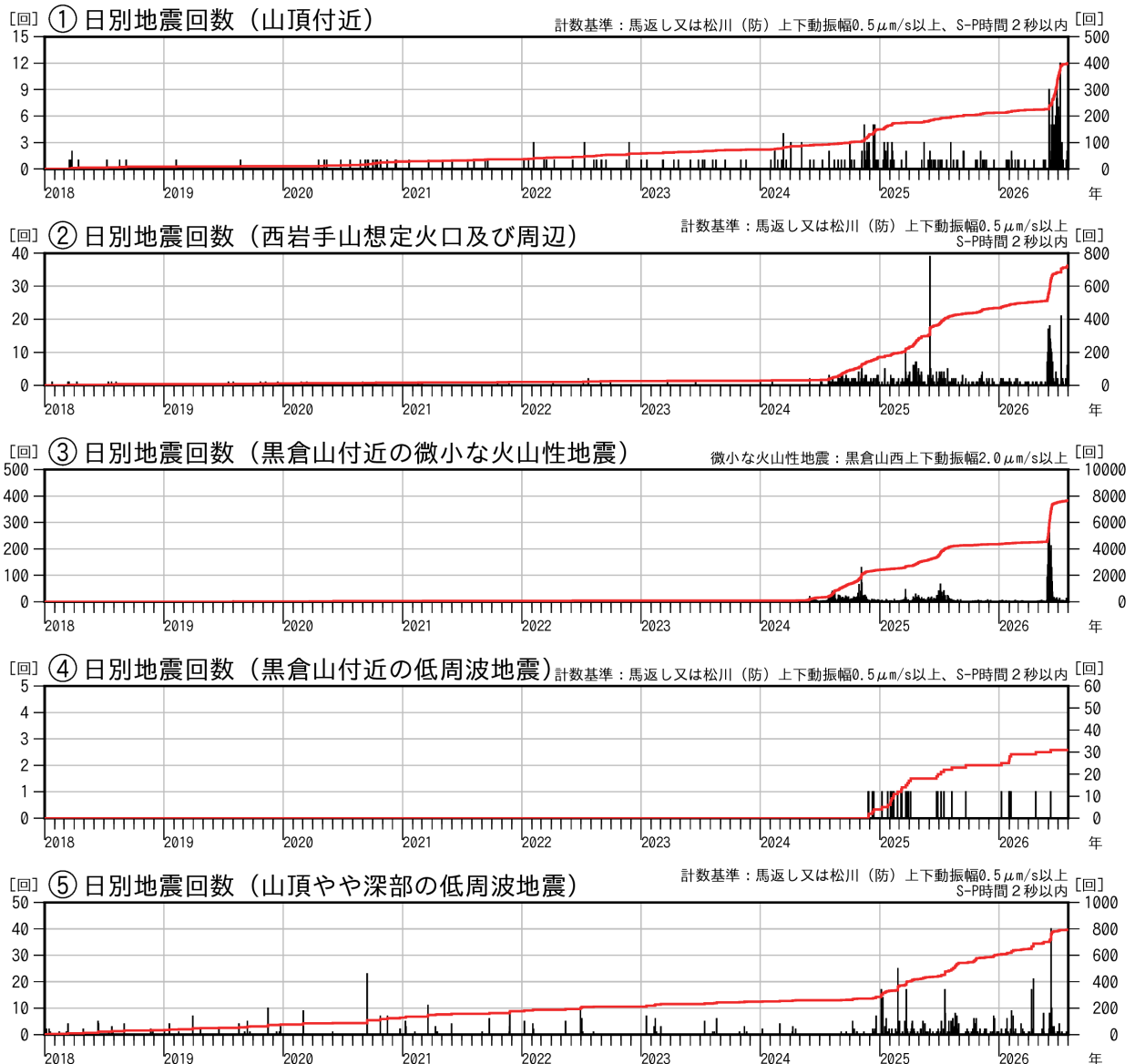
図2 岩手山 日別地震回数（2018年1月～2026年7月）
