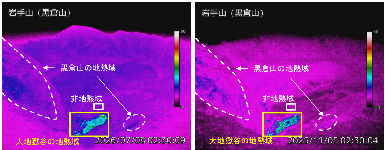
図 5－1 岩手山 黒倉山監視カメラからの地表面温度分布
