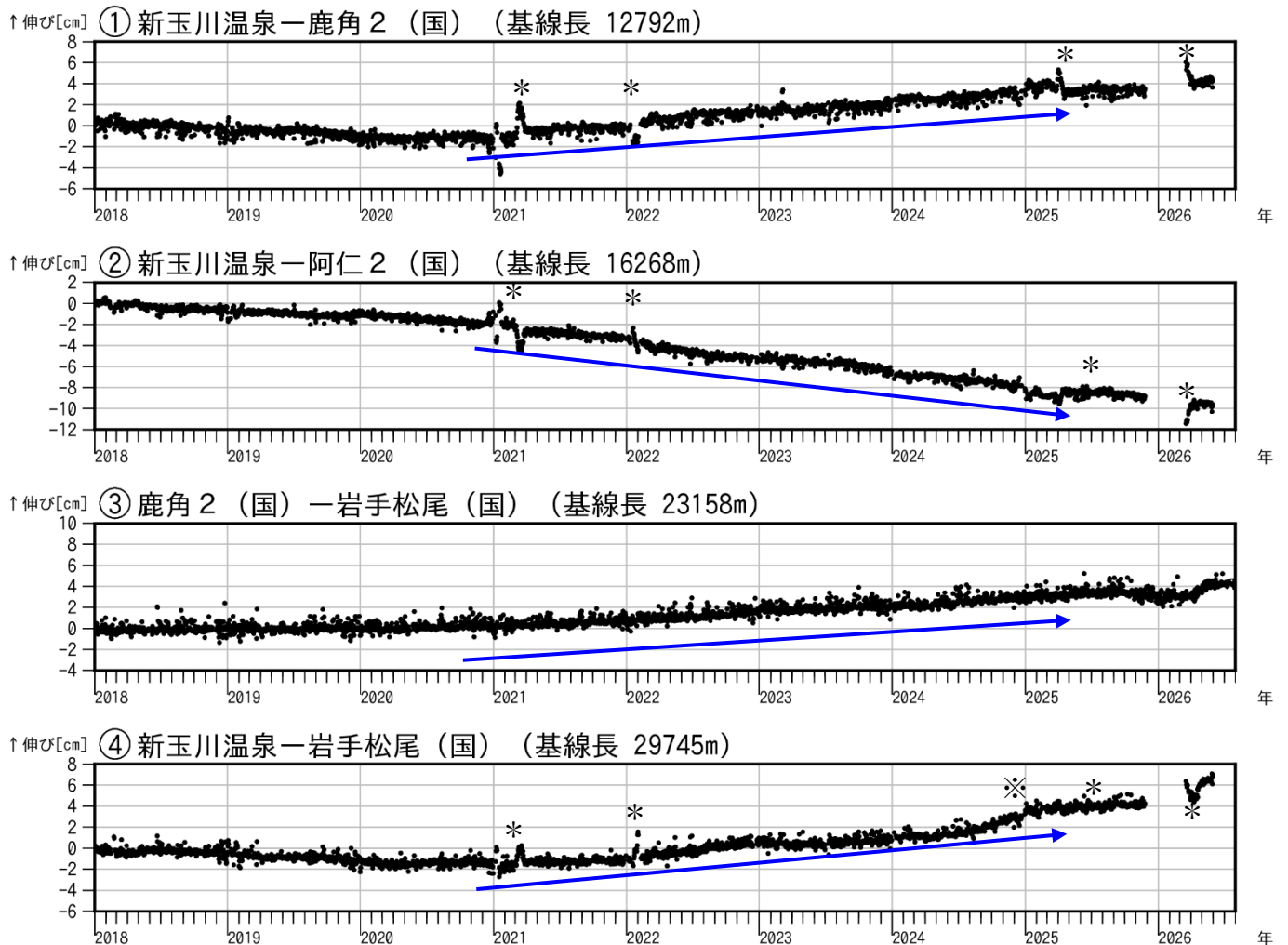
図 4 秋田焼山 GNSS 基線長変化図（2018 年 1 月～2026 年 7 月）
