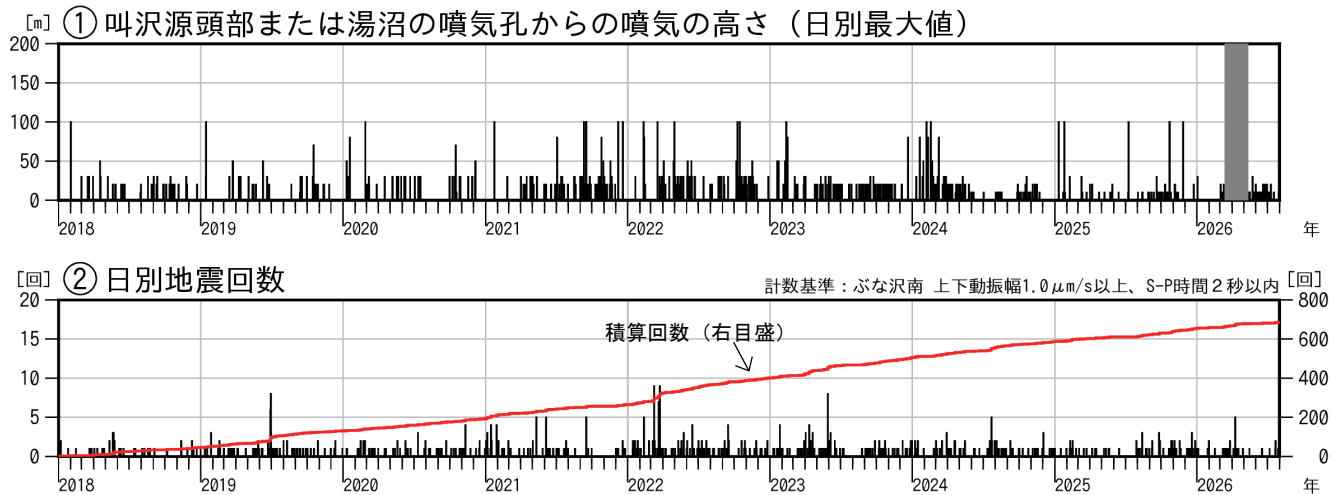
図 3 秋田焼山 火山活動経過図（2018 年 1 月～2026 年 7 月）
