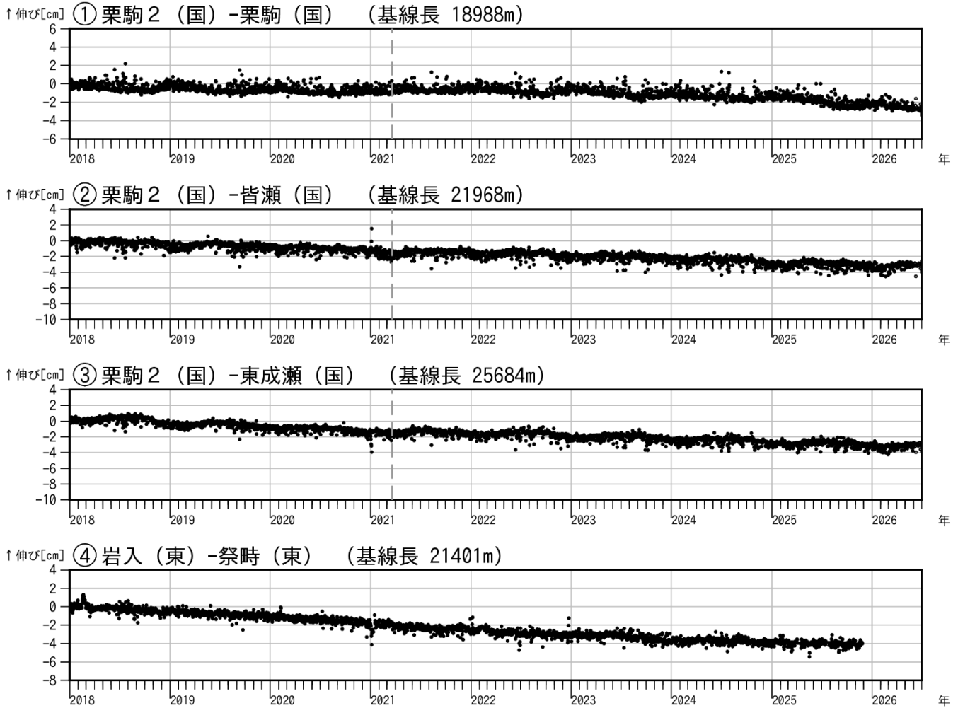
図7 栗駒山 GNSS 基線長変化図（2018年1月～2026年6月）
