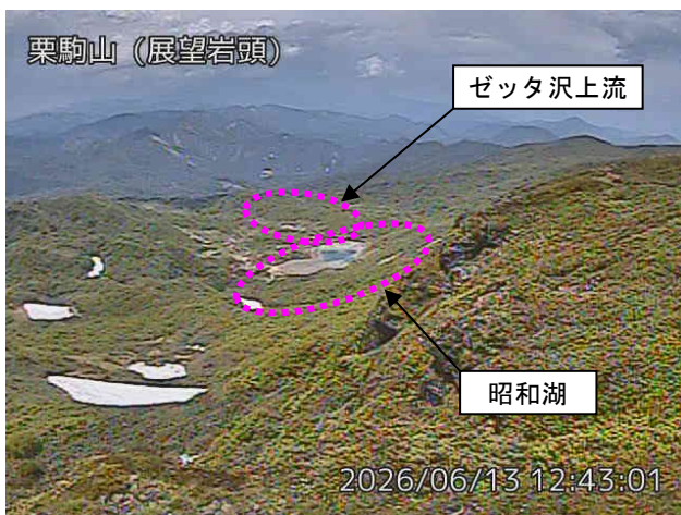
図2 栗駒山 昭和湖及びゼッタ沢上流周辺の状況（6月13日）と地表面温度分布（6月30日） ・展望岩頭監視カメラ（昭和湖の南南西約900m）の可視及び赤外熱画像です。
