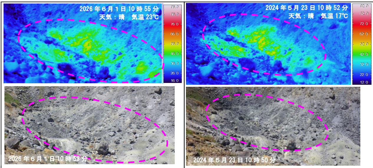
図4 栗駒山 北東から撮影したゼッタ沢上流の状況と地表面温度分布
