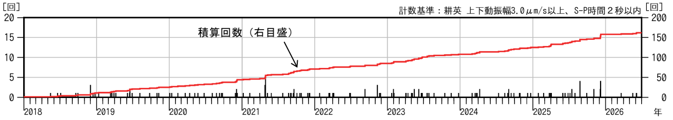
図6 栗駒山 日別地震回数（2018年1月～2026年6月）
