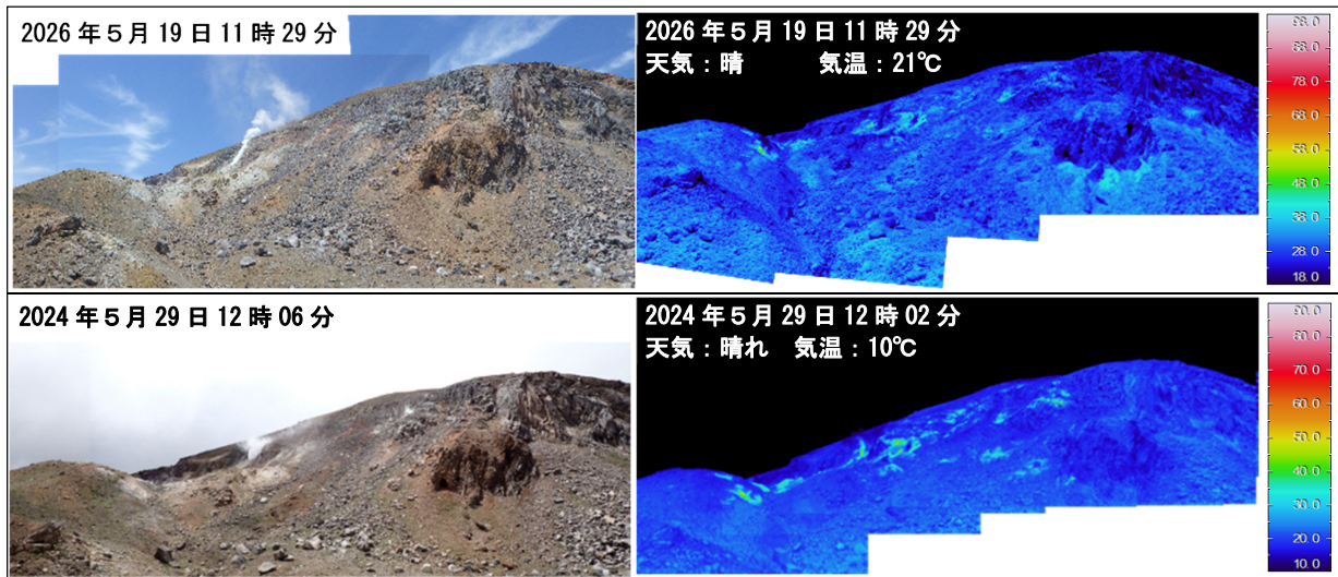
図4 吾妻山 大穴火口東及びその周辺の状況と地表面温度分布図
