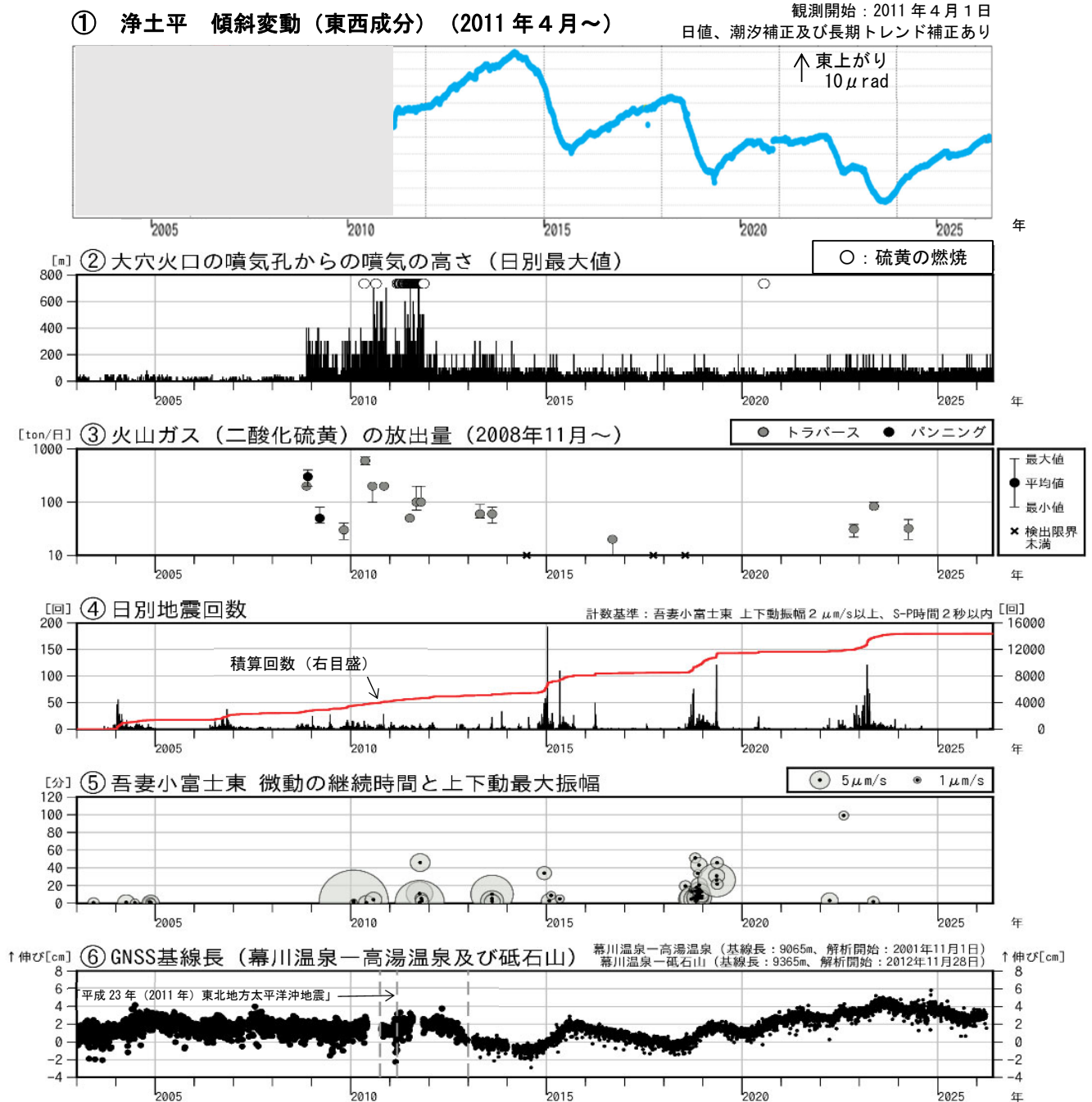
図6 吾妻山 中期的な火山活動の経過（2003年1月～2026年5月）
