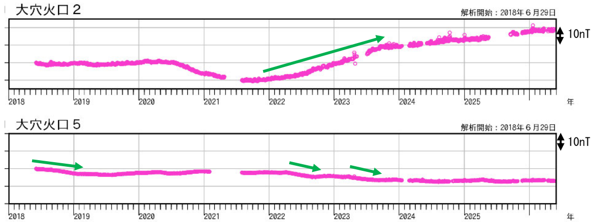
図8 吾妻山 全磁力連続観測点の全磁力値変化（2018年1月～2026年5月）
