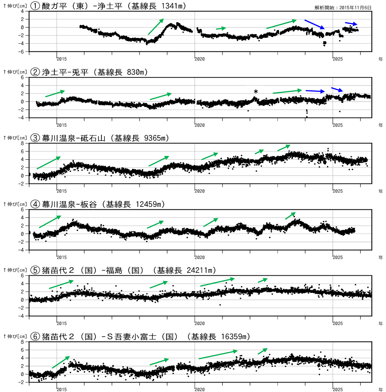
図7 吾妻山 吾妻山浅部・深部の地殻変動（2014年1月～2026年5月）
