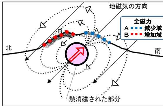
図9 熱消磁に伴う全磁力変化のモデル
