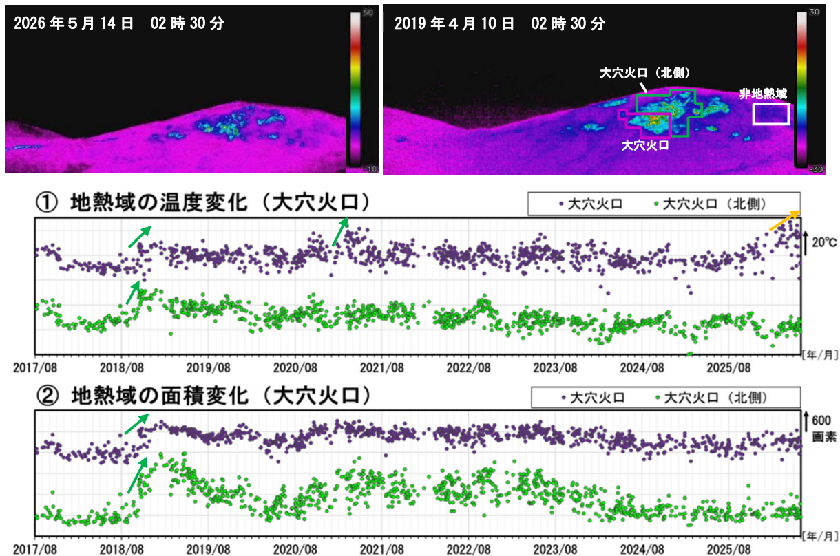
図2 吾妻山 監視カメラによる大穴火口周辺の地熱域の経過（2017年8月～2026年5月）
