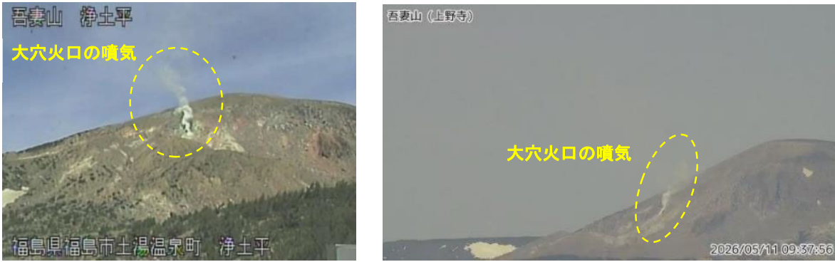
図1 吾妻山 大穴火口周辺の噴気の状態（5月11日）
