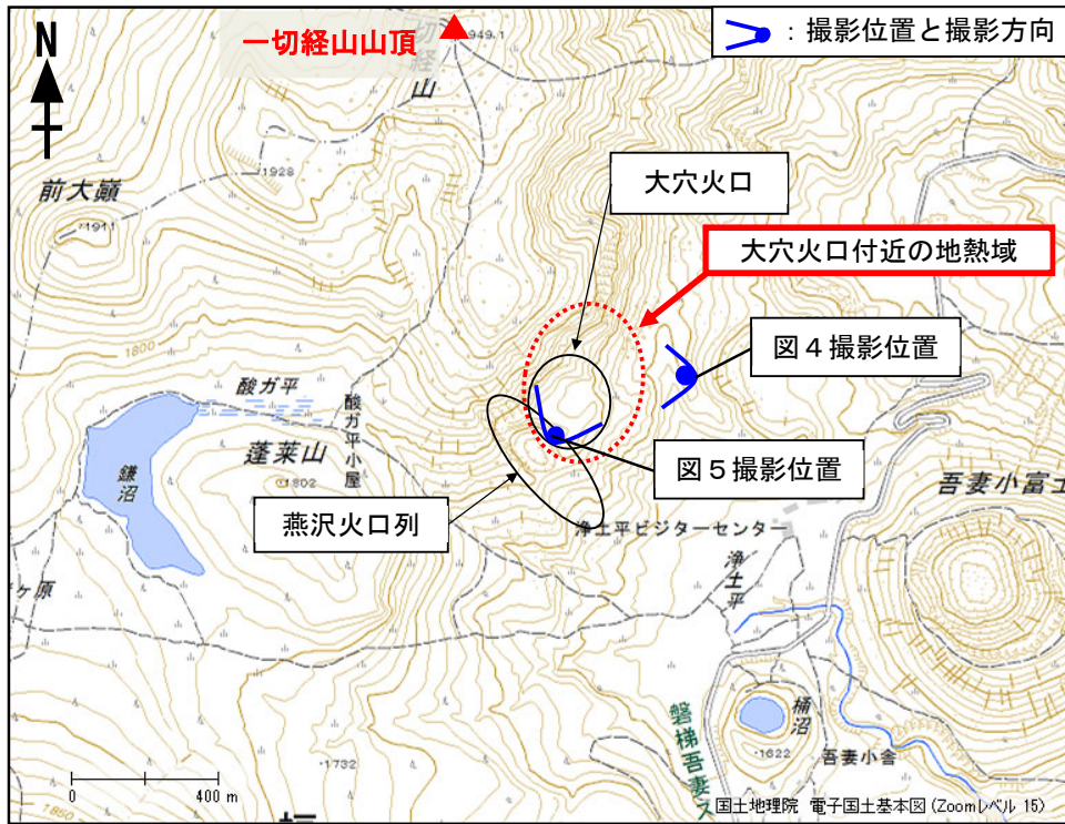
図3 吾妻山 大穴火口周辺の噴気と地熱域の分布及び写真と地表面温度分布撮影位置、撮影方向
