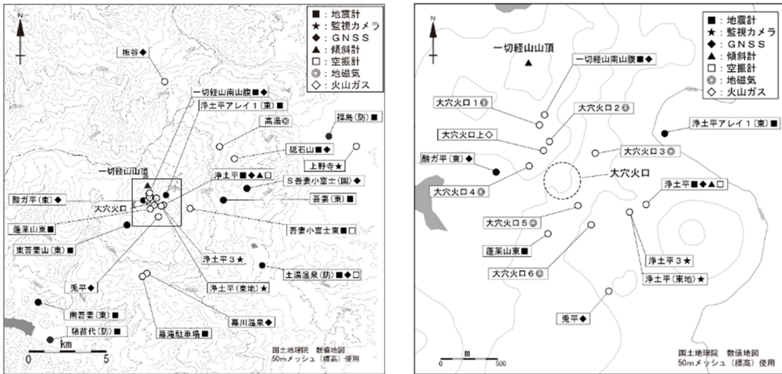
図10 吾妻山 観測点配置図
