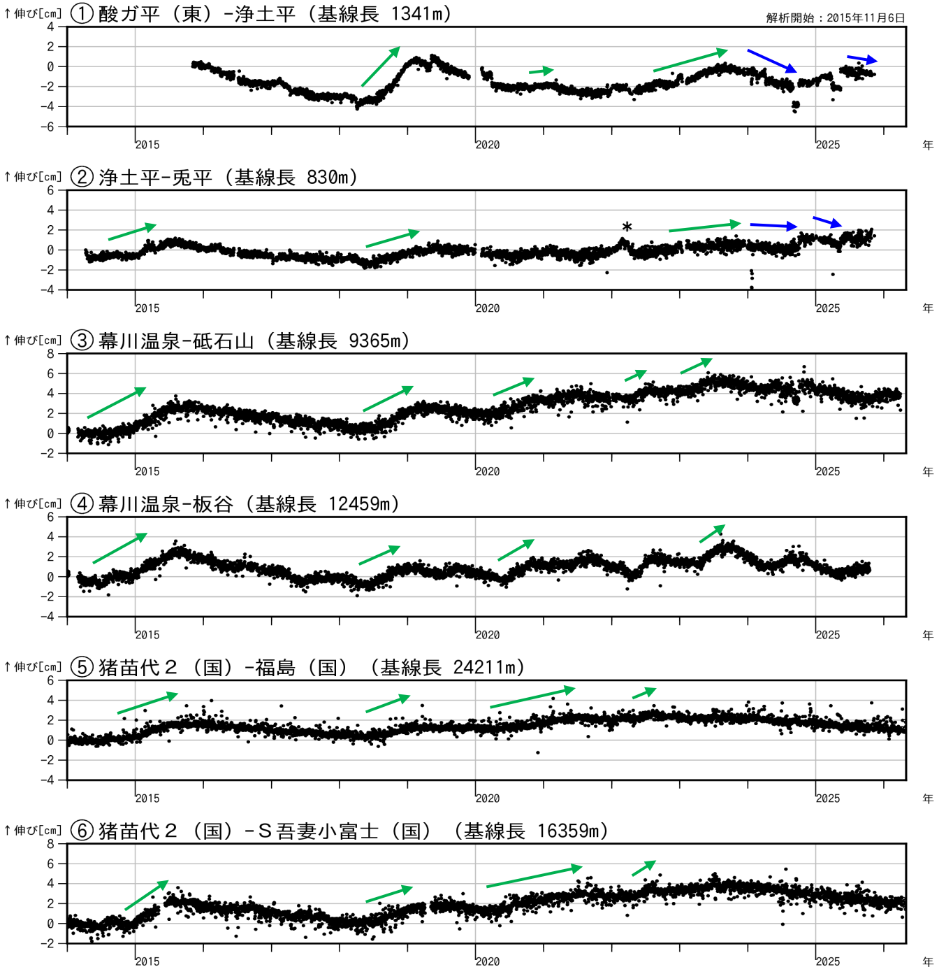
図4 吾妻山 吾妻山浅部・深部の地殻変動（2014年1月～2026年4月）
