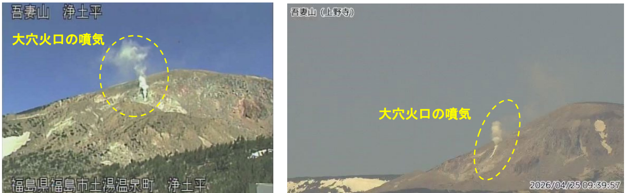
図1 吾妻山 大穴火口周辺の噴気の状態（4月25日）
