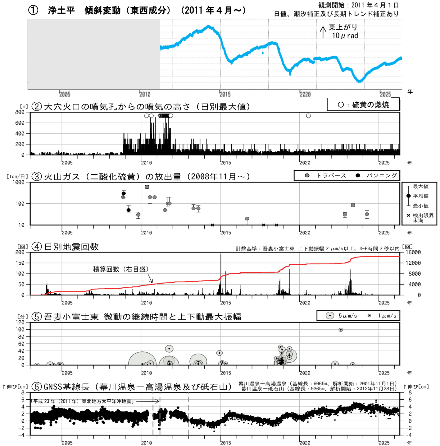
図3 吾妻山 中期的な火山活動の経過（2003年1月～2026年4月）
