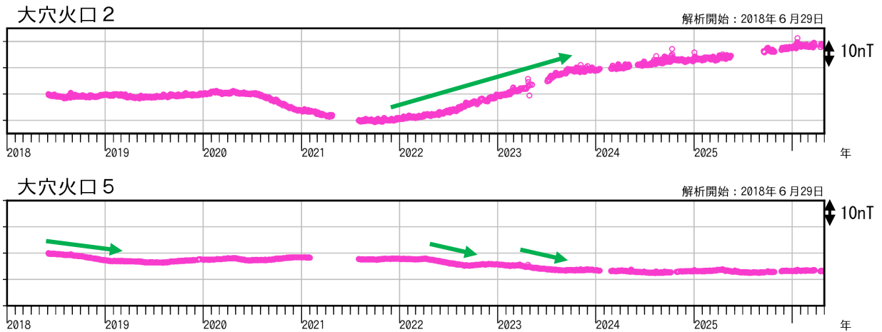
図5 吾妻山 全磁力連続観測点の全磁力値変化（2018年1月～2026年4月）
