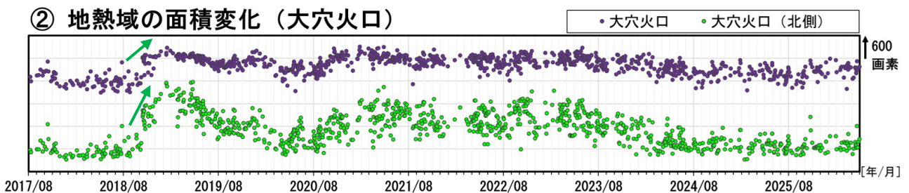
図2 吾妻山 監視カメラによる大穴火口周辺の地熱域の経過（2017年8月～2026年4月）
