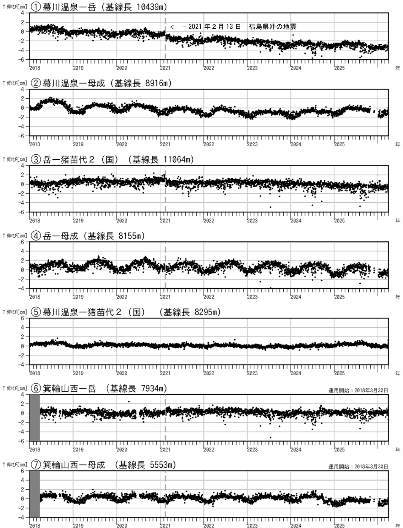
図4 安達太良山 GNSS 基線長変化図（2018年1月～2026年3月）
