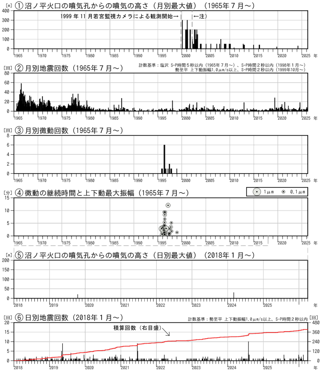
図3 安達太良山 火山活動経過図（1965年7月～2026年3月）
