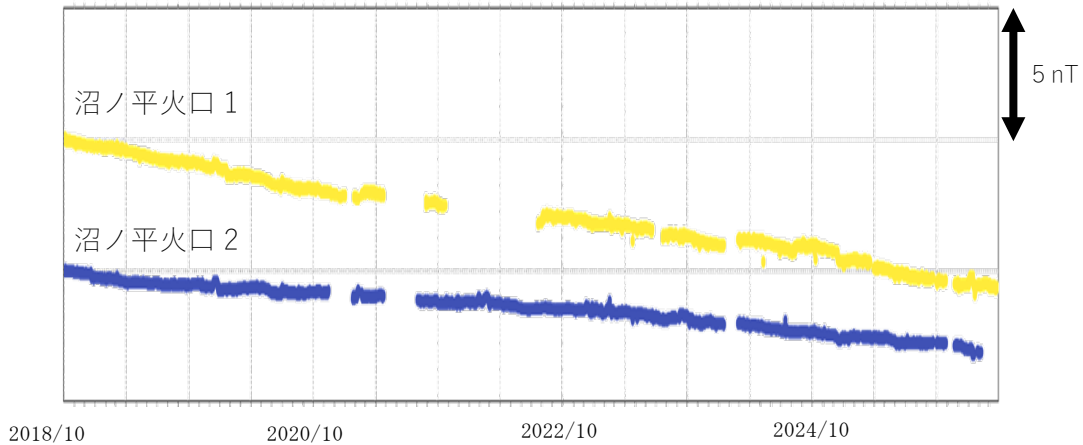
図5 安達太良山 全磁力連続観測結果（2018年10月～2026年3月）
