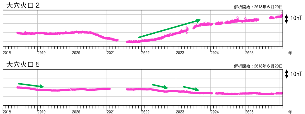
図6 吾妻山 全磁力連続観測点の全磁力値変化（2018年1月～2026年1月）
