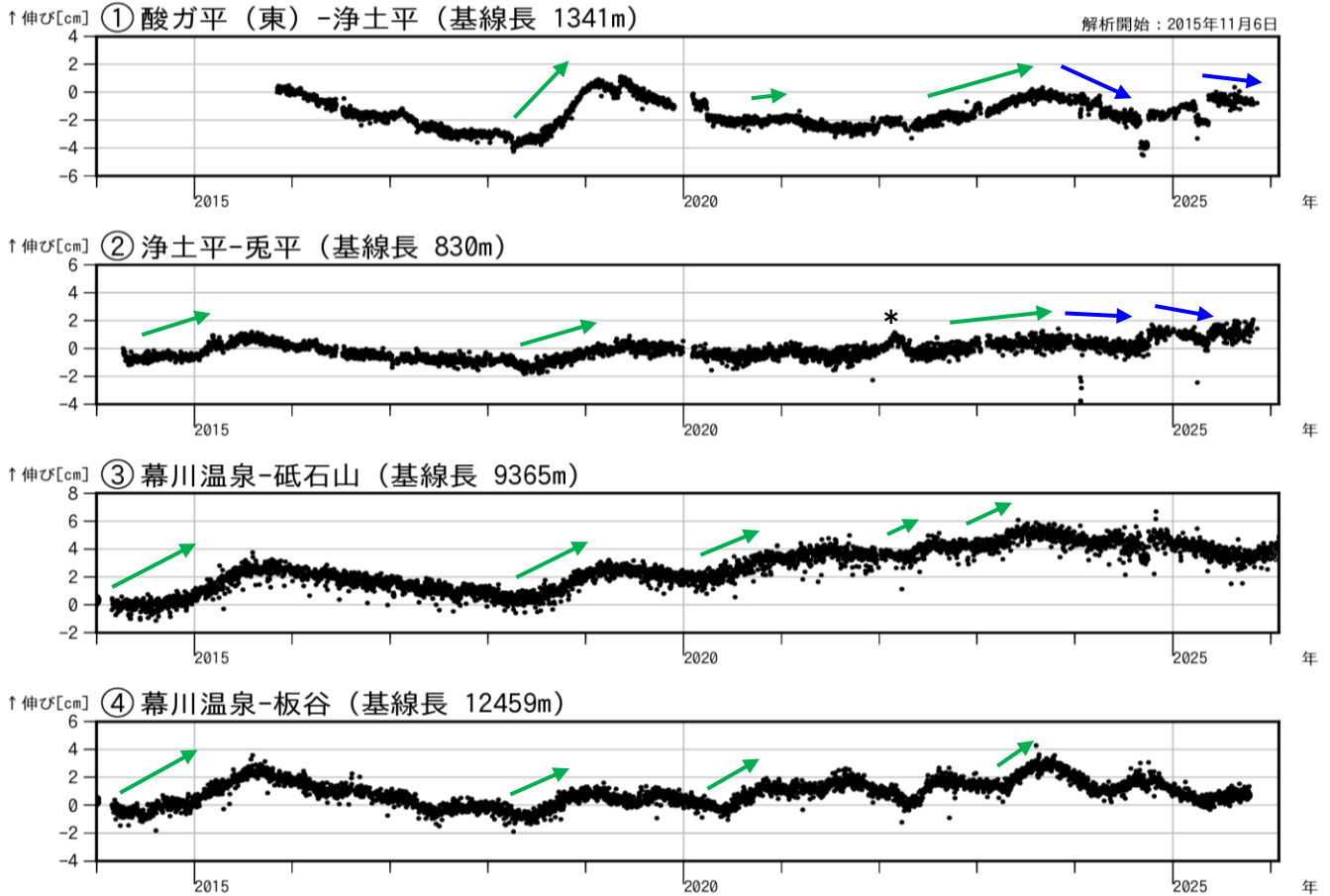
図 4 吾妻山 吾妻山浅部・深部の地殻変動（2014 年 1 月～2026 年 1 月）
