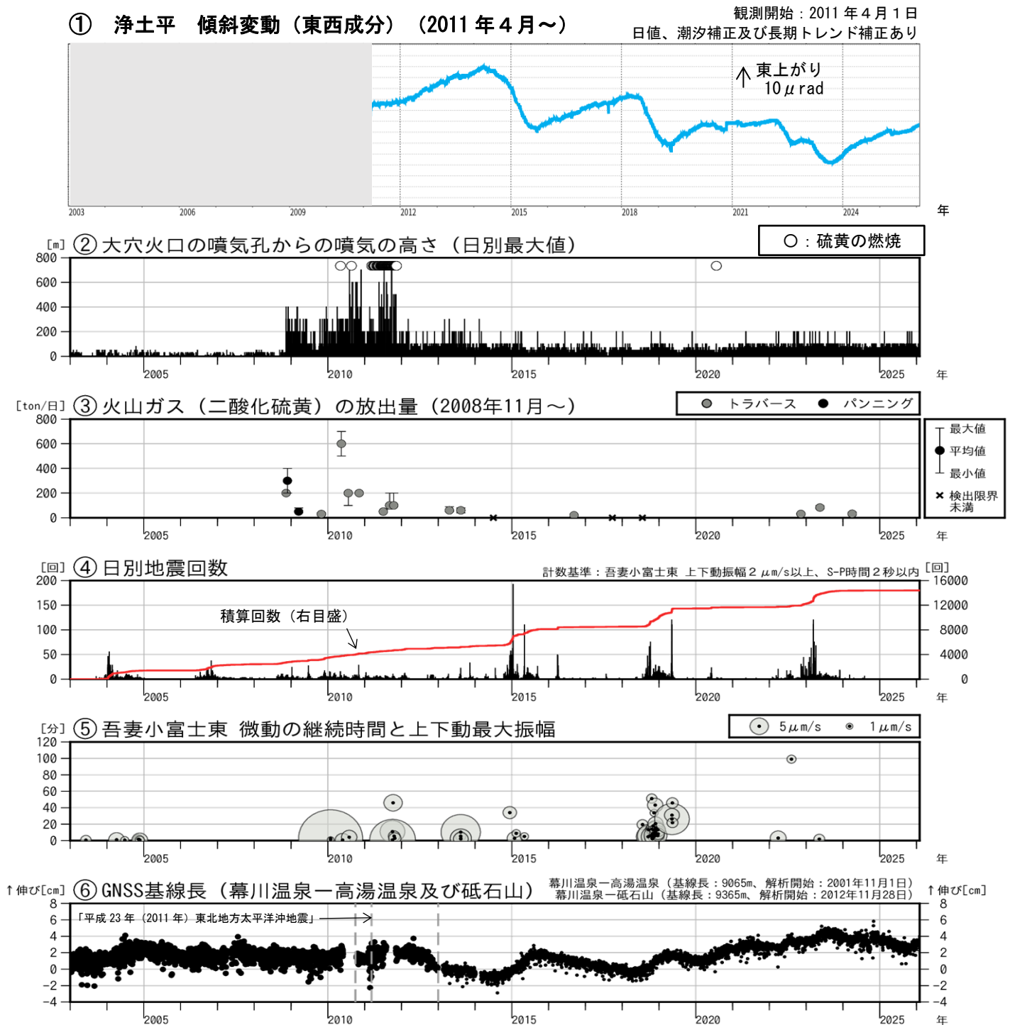
図3 吾妻山 中期的な火山活動の経過（2003年1月～2026年1月）
