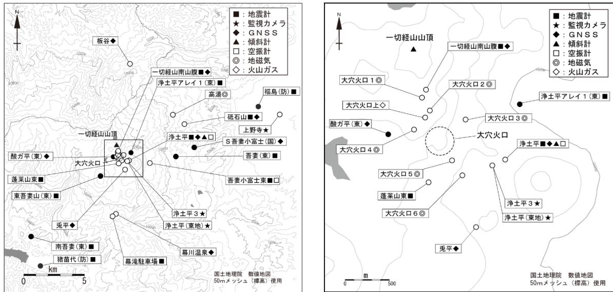
図8 吾妻山 観測点配置図
