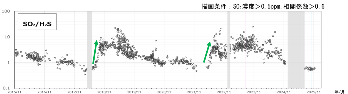
図 5 吾妻山 火山ガス観測装置による観測（2015 年 11 月～2026 年 1 月）
