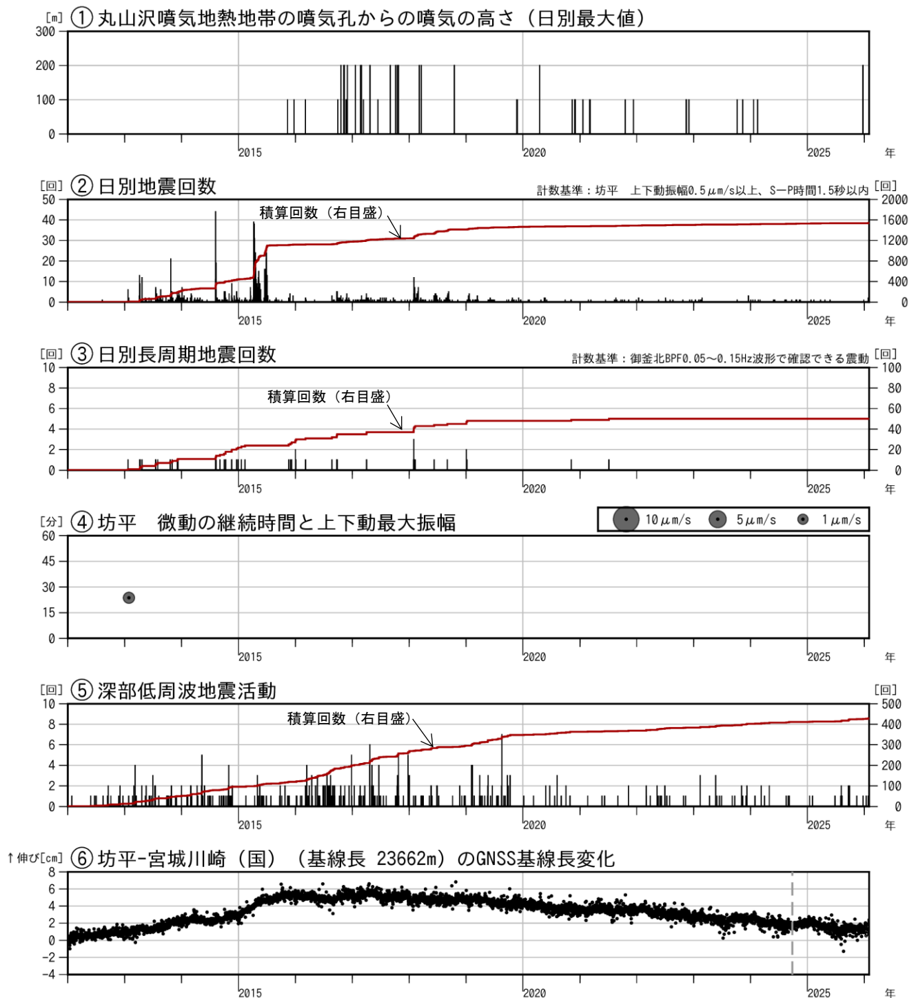
図2 蔵王山 火山活動経過図（2012年1月～2026年1月）
