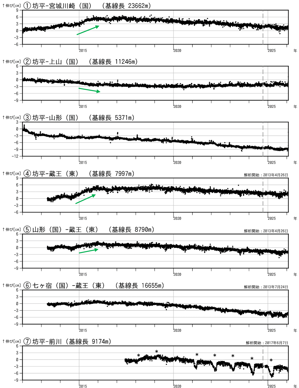
図3 蔵王山 GNSS 基線長変化図（2012年1月～2026年1月）
