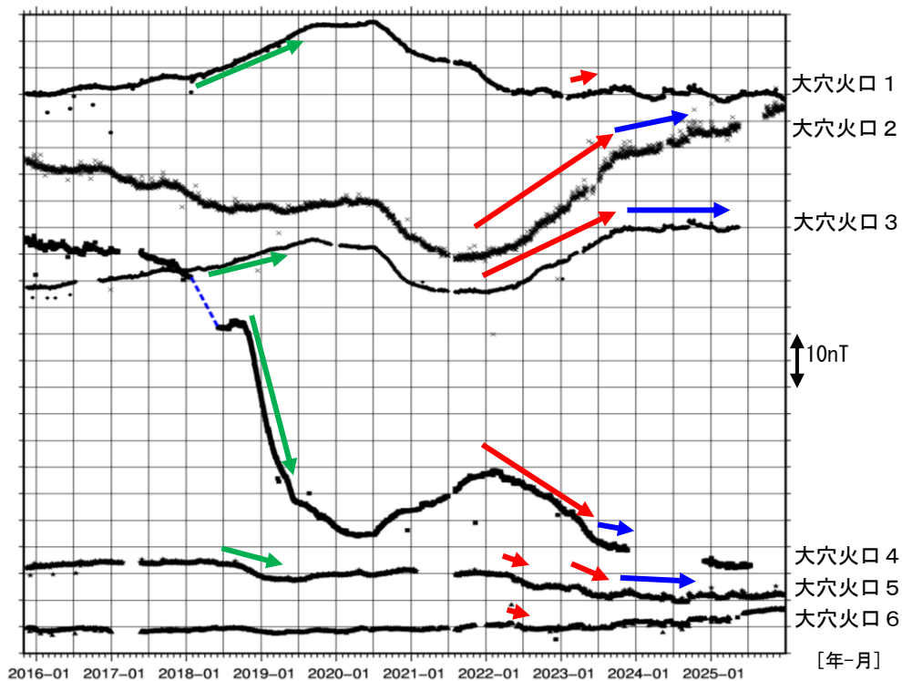
図7 吾妻山 全磁力連続観測点の全磁力値変化（2015 年 11 月～2025 年 12 月）
