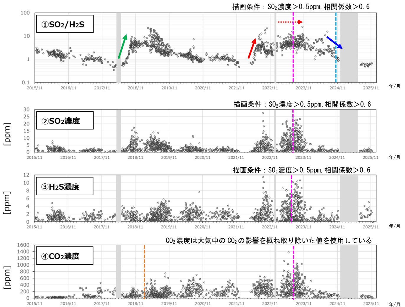
図6 吾妻山 火山ガス観測装置による観測（2015年11月～2025年12月）
