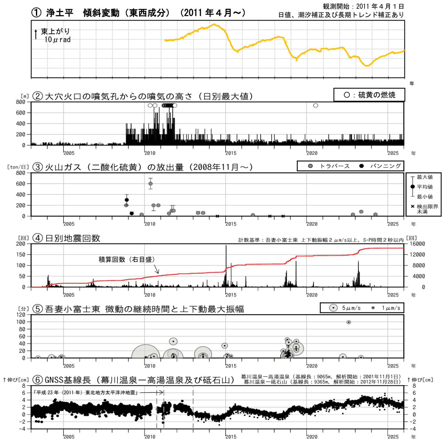
図2 吾妻山 中期的な火山活動の経過（2003年1月～2025年12月）
