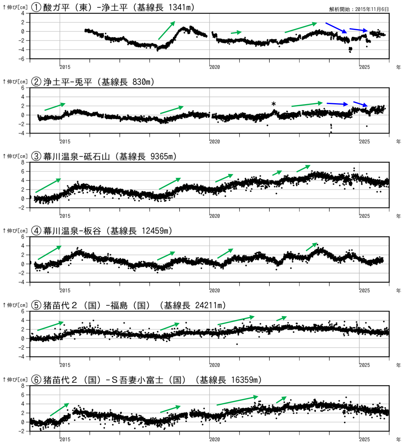
図4 吾妻山 吾妻山浅部・深部の地殻変動（2014年1月～2025年12月）
