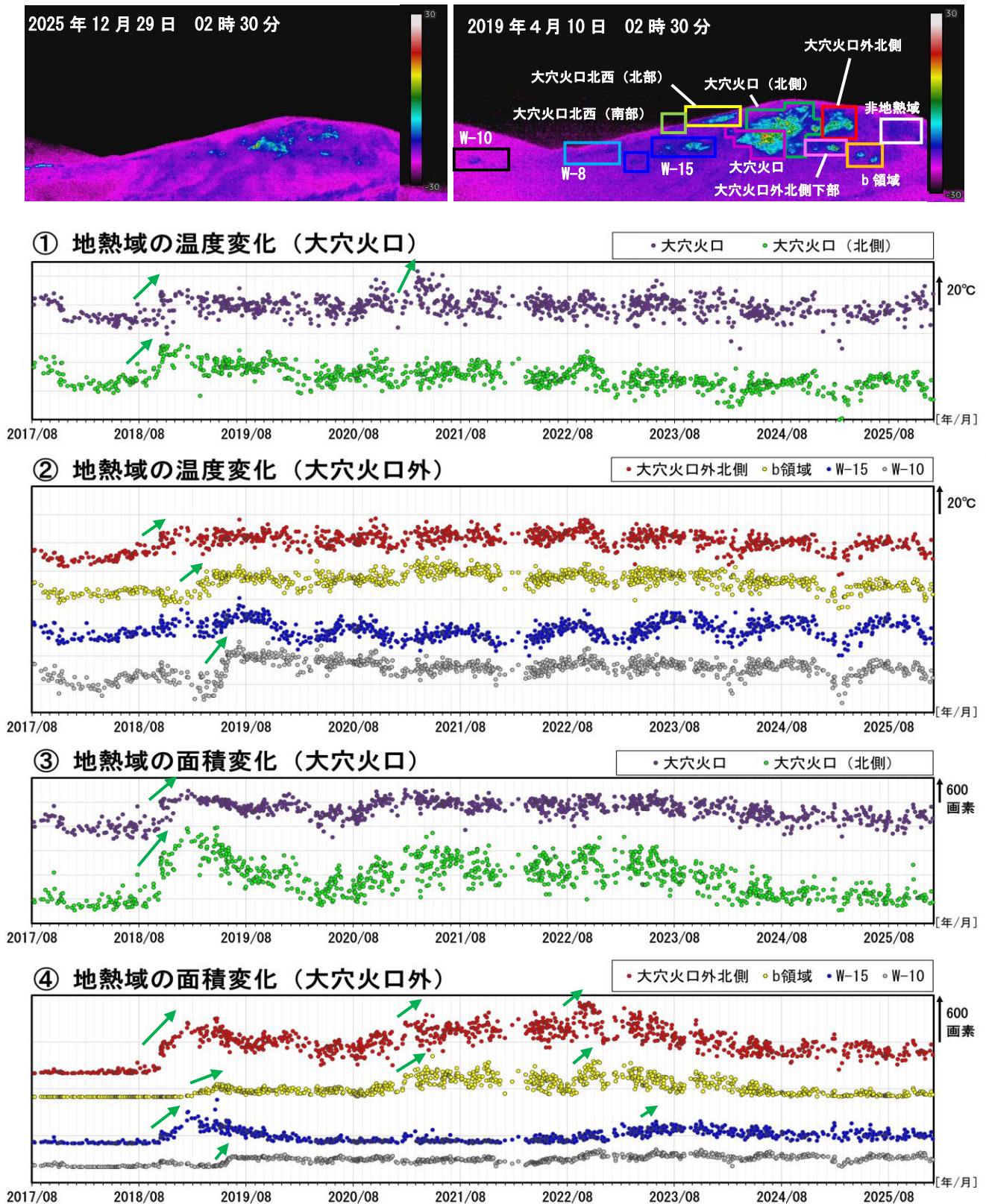
図5 吾妻山 監視カメラによる大穴火口周辺の地熱域の経過（2017 年 8 月～2025 年 12 月）
