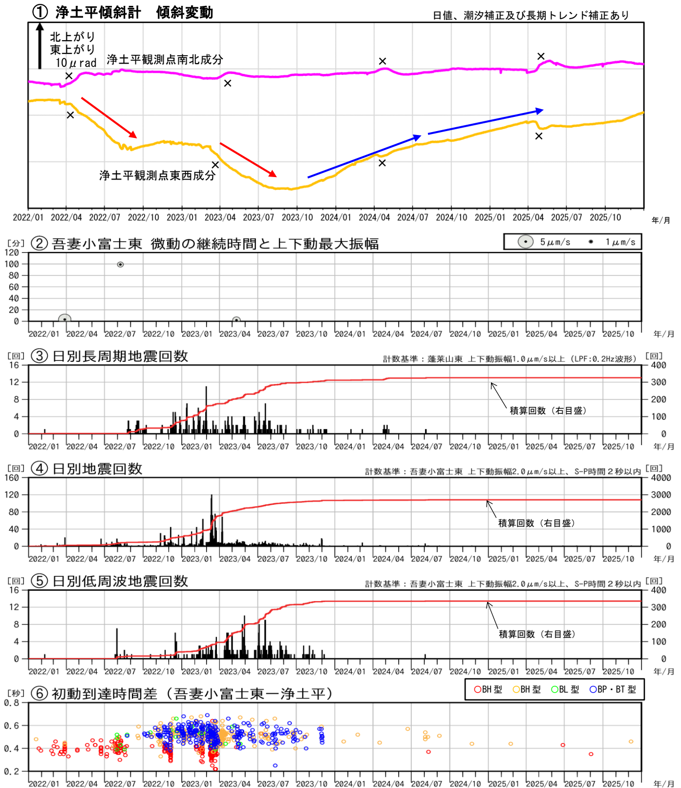
図3 吾妻山 火山活動経過図（2022年1月～2025年12月）
