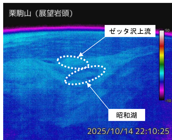
図 2 栗駒山 昭和湖及びゼッタ沢上流周辺の状況（10 月 9 日）と地表面温度分布（10 月 14 日） ・展望岩頭監視カメラ（昭和湖の南南西約 900m）の映像です。
