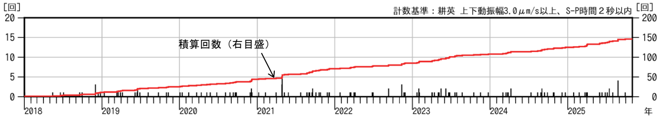
図3 栗駒山 日別地震回数 (2018 年 1 月～2025 年 10 月)
