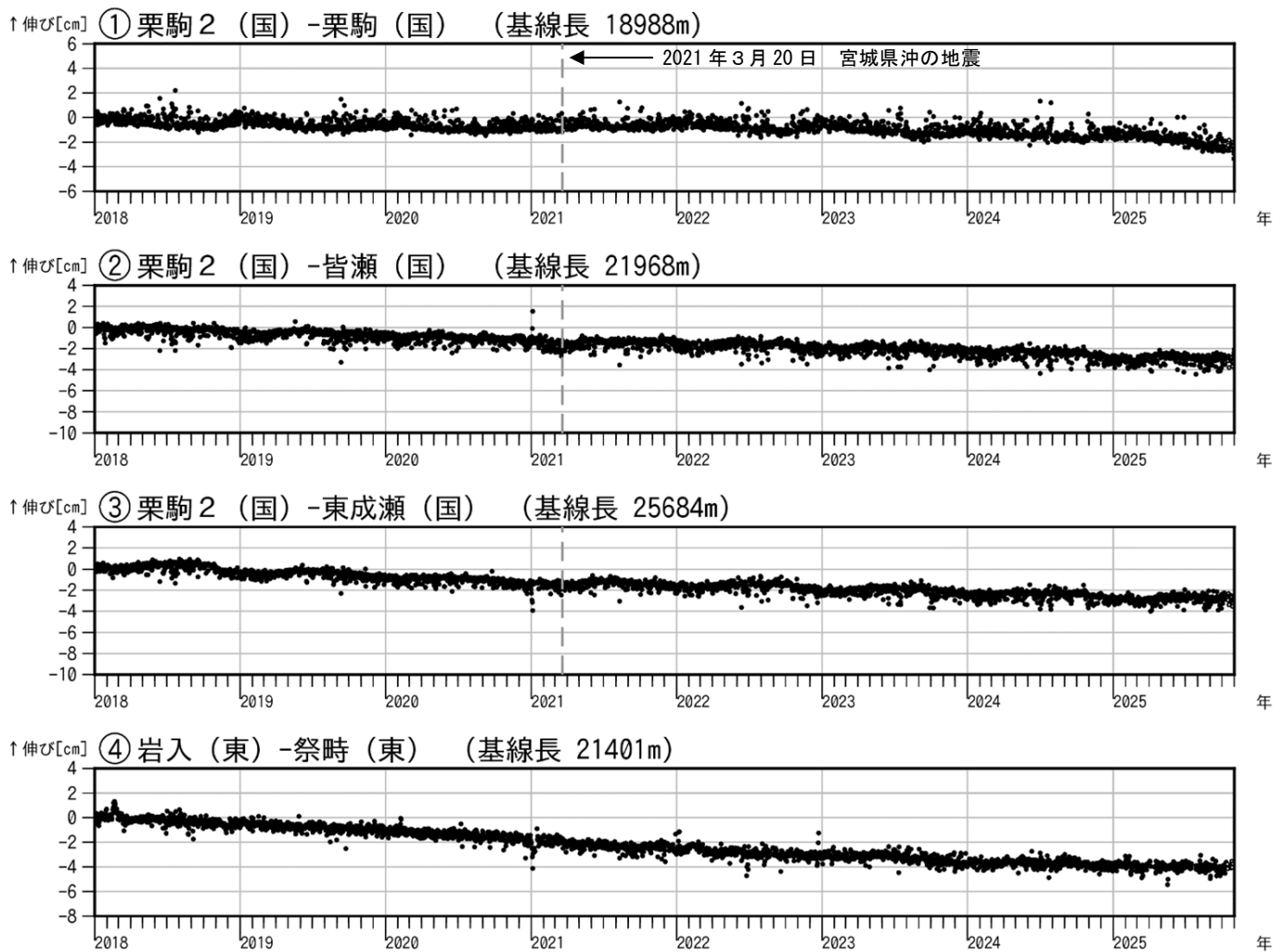
図4 栗駒山 GNSS 基線長変化図 (2018 年 1 月～2025 年 10 月)
