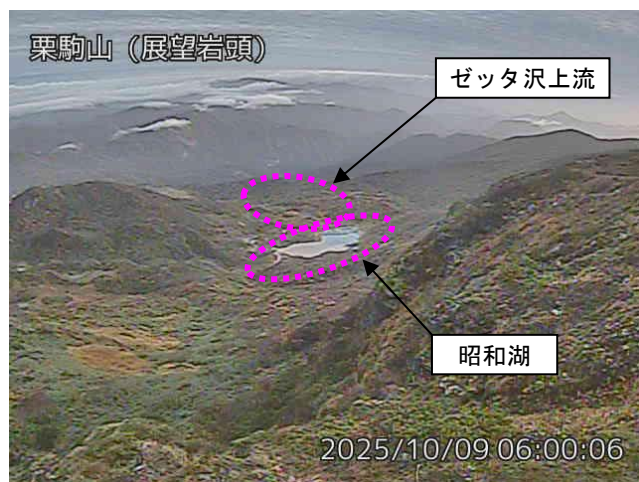
図 2 栗駒山 昭和湖及びゼッタ沢上流周辺の状況（10 月 9 日）と地表面温度分布（10 月 14 日） ・展望岩頭監視カメラ（昭和湖の南南西約 900m）の映像です。
