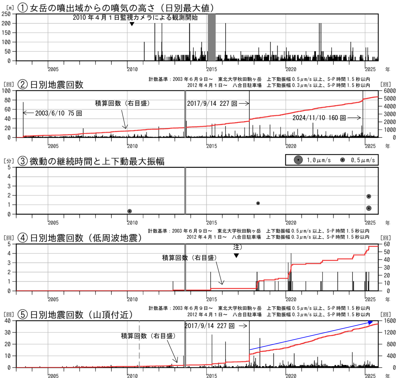
図2 秋田駒ヶ岳 火山活動経過図（2003年6月～2025年10月）
