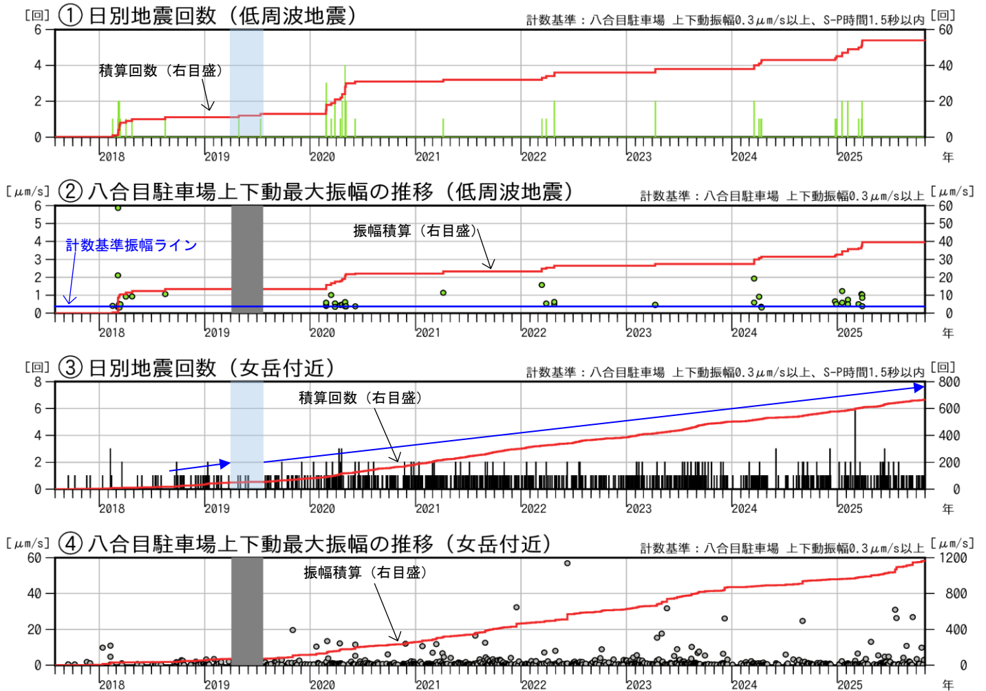
図3 秋田駒ヶ岳 低周波地震及び女岳付近の日別回数と最大振幅（2017年8月～2025年10月）
