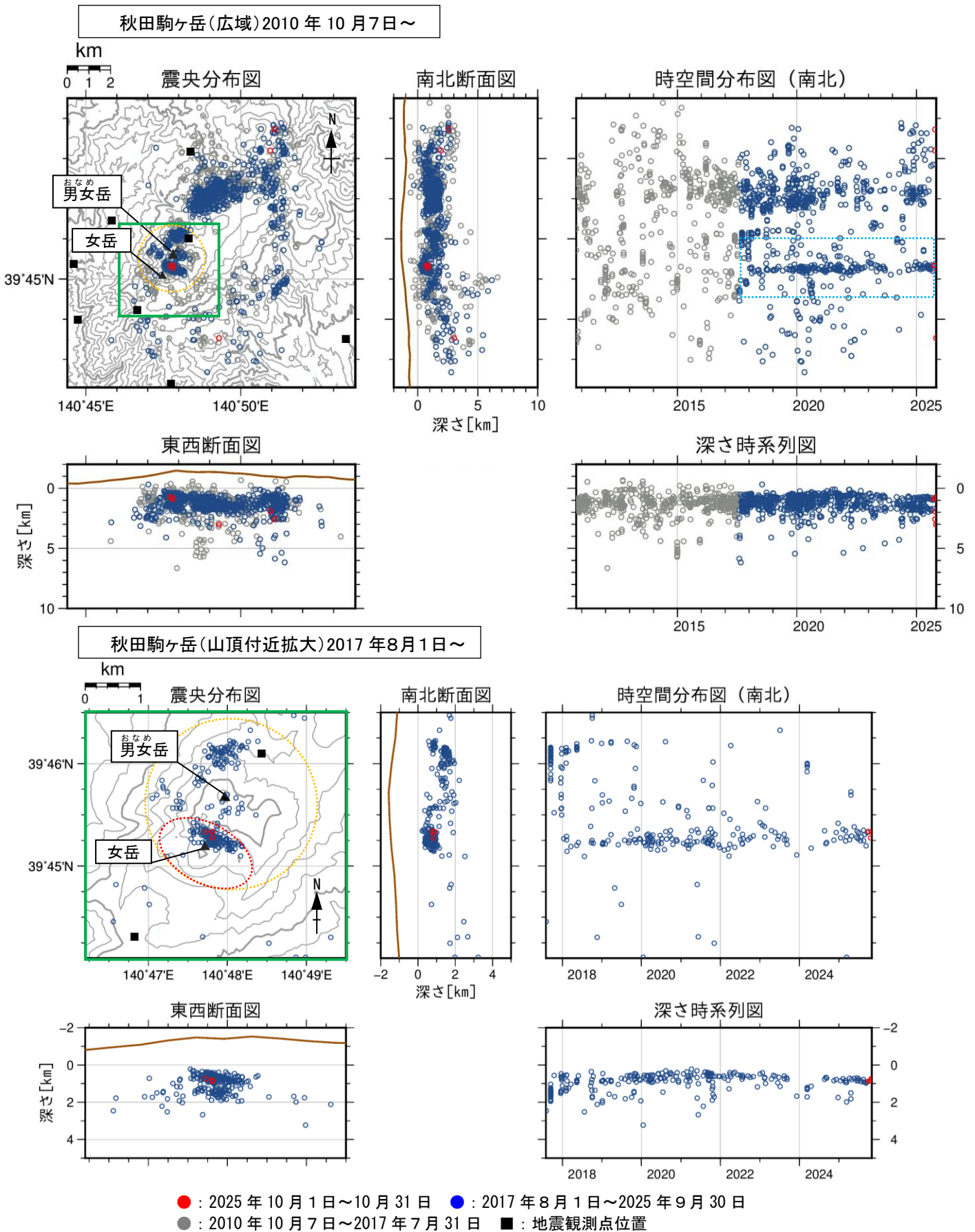
図4 秋田駒ヶ岳 地震活動（2010年10月7日～2025年10月）
