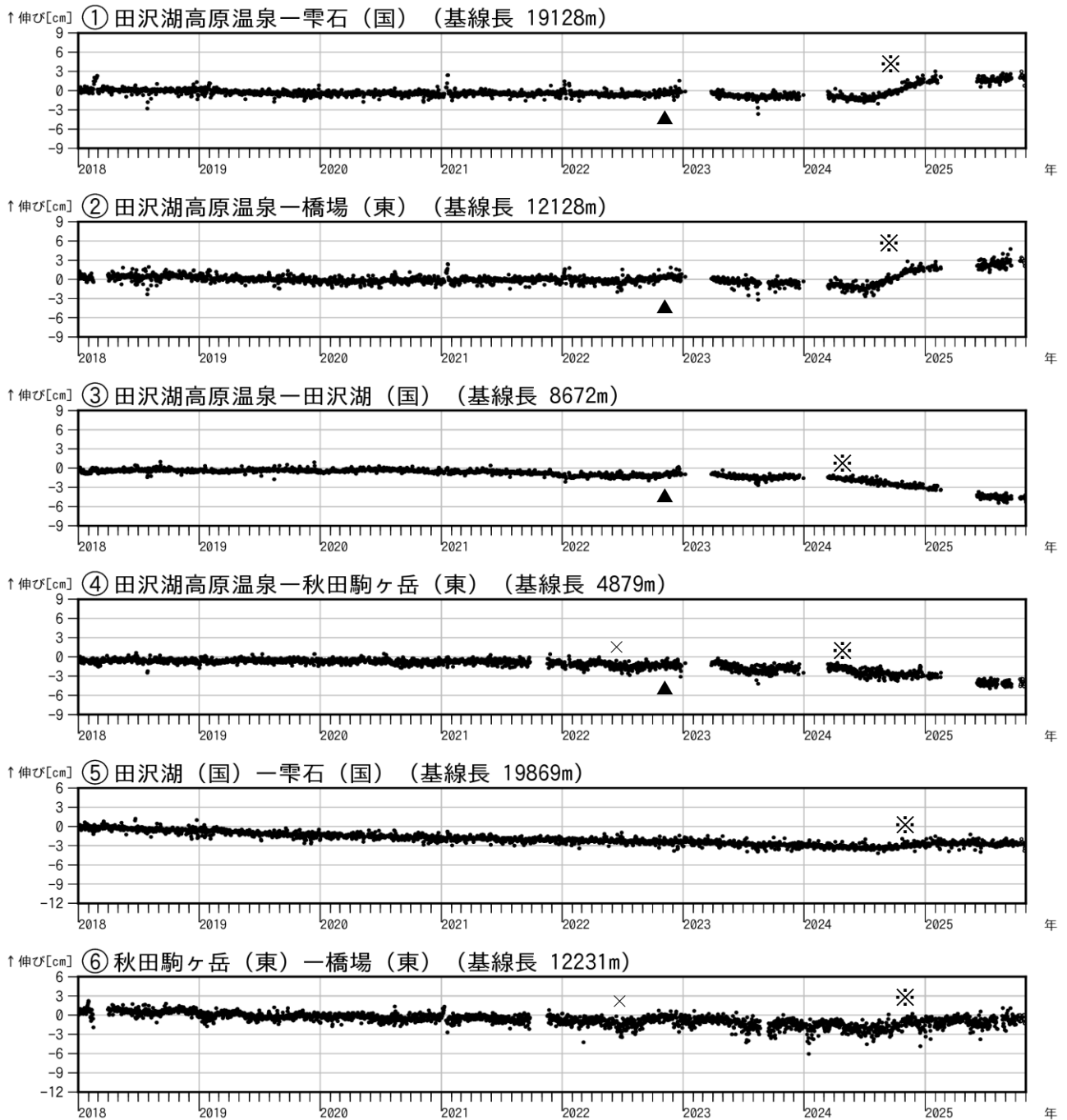
図5 秋田駒ヶ岳 GNSS 基線長変化図（2018年1月～2025年10月）
