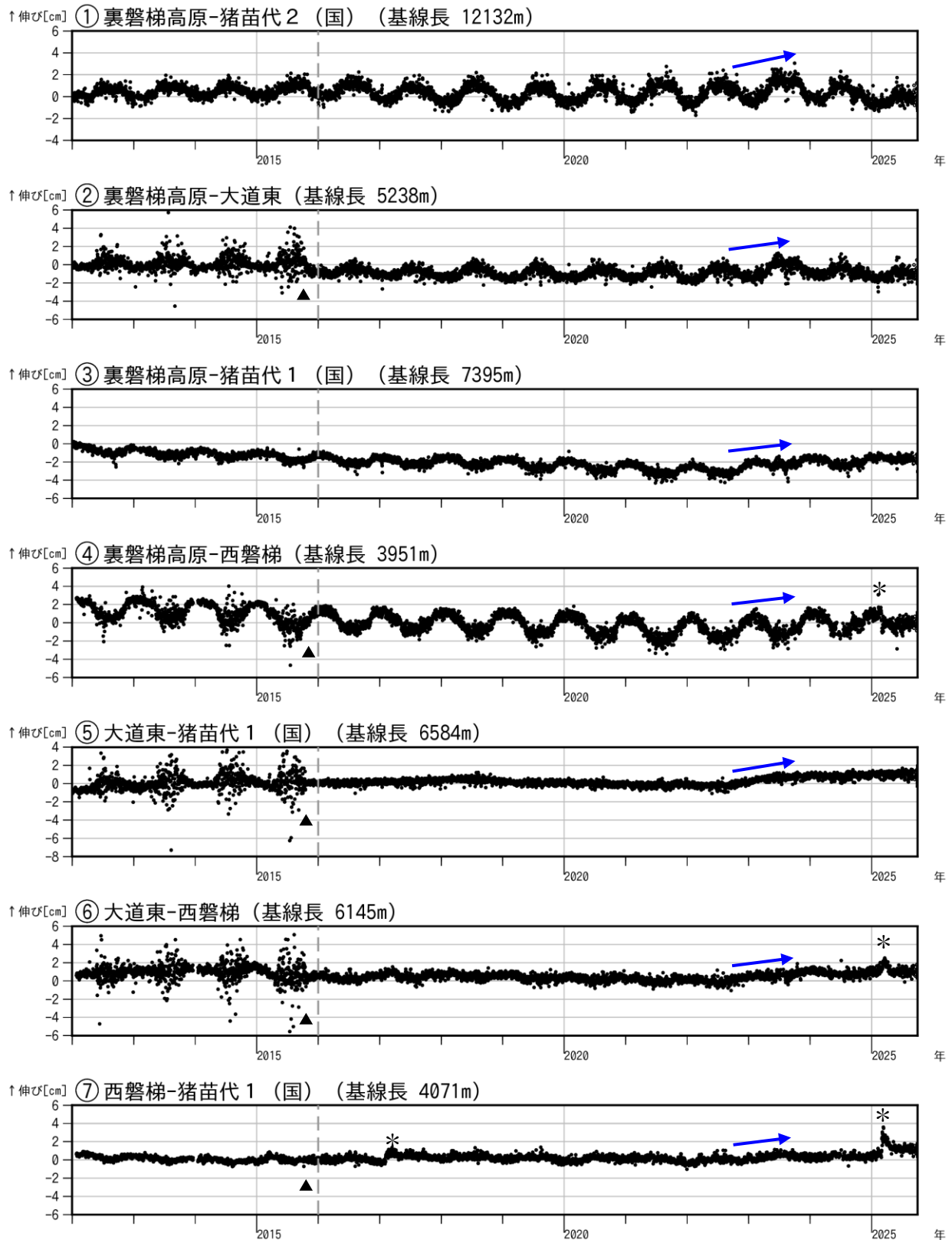
図6 磐梯山 GNSS 基線長変化図（2012年1月～2025年9月）
