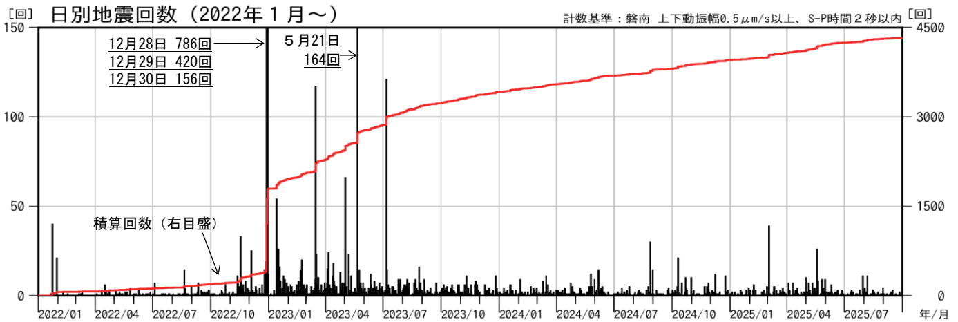
図 4 磐梯山 地震回数（2022 年 1 月～2025 年 9 月）
