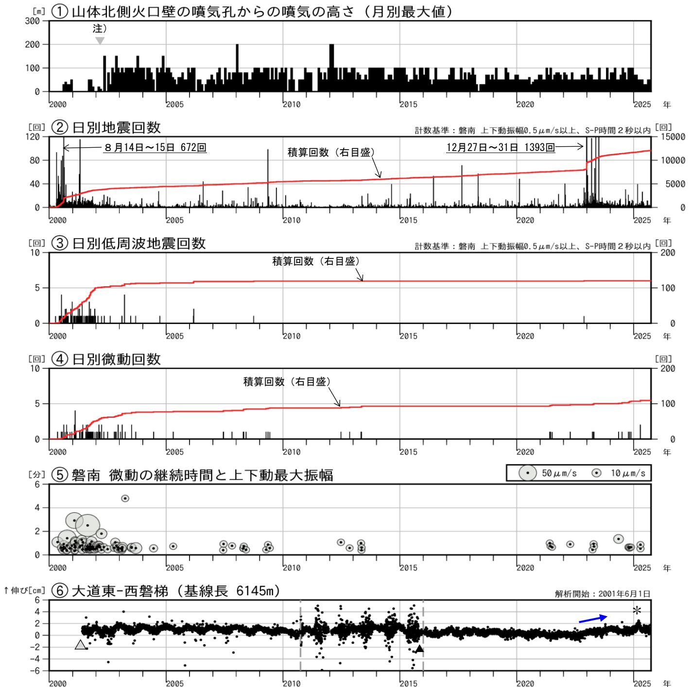
図3 磐梯山 火山活動経過図（2000年1月～2025年9月）
