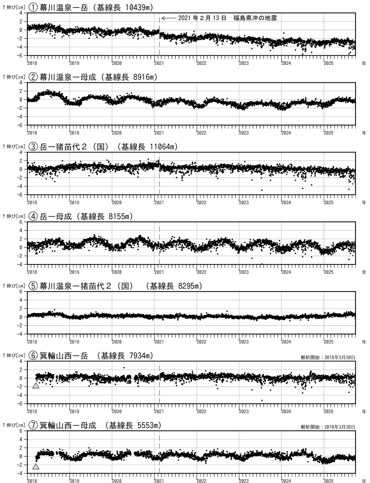
図4 安達太良山 GNSS 基線長変化図（2018年1月～2025年9月）
