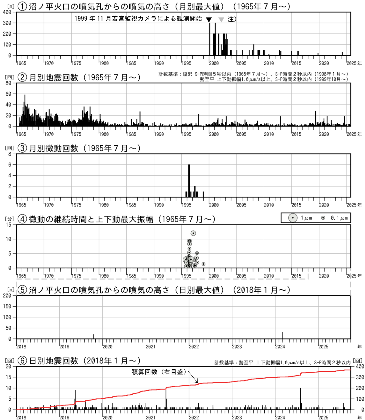
図3 安達太良山 火山活動経過図（1965年7月～2025年9月）
