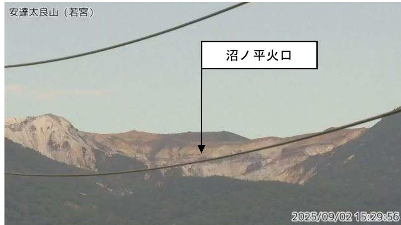
図1 安達太良山 沼ノ平火口周辺の状況（9月2日） ・若宮監視カメラ（沼ノ平火口の西北西約8km）の映像です。
