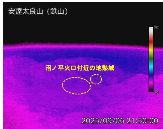
図2 安達太良山 沼ノ平火口周辺の状況（9月1日）と地表面温度分布の状況（9月6日） ・鉄山監視カメラ（沼ノ平火口の北東約700m）の映像です。
