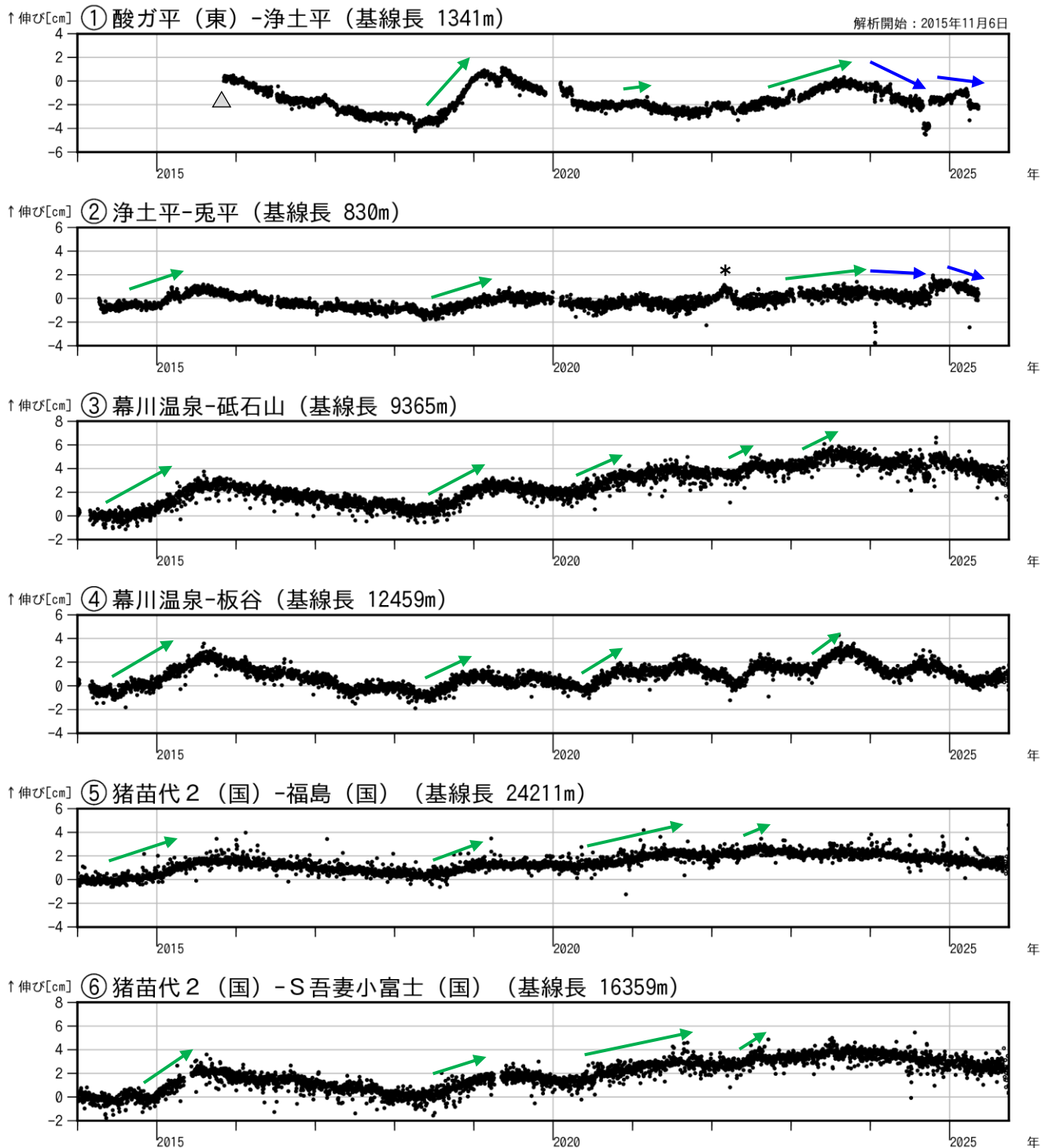
図4 吾妻山 吾妻山浅部・深部の地殻変動（2014年1月～2025年9月）
