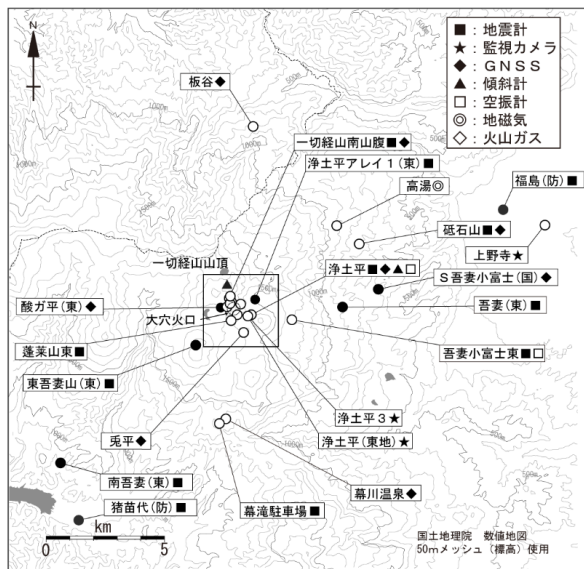
図8 吾妻山 観測点配置図
