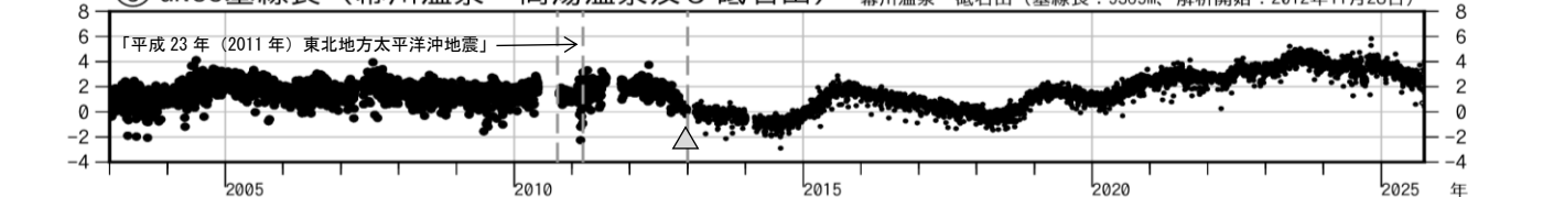
図2 吾妻山 中期的な火山活動の経過（2003年1月～2025年9月）
