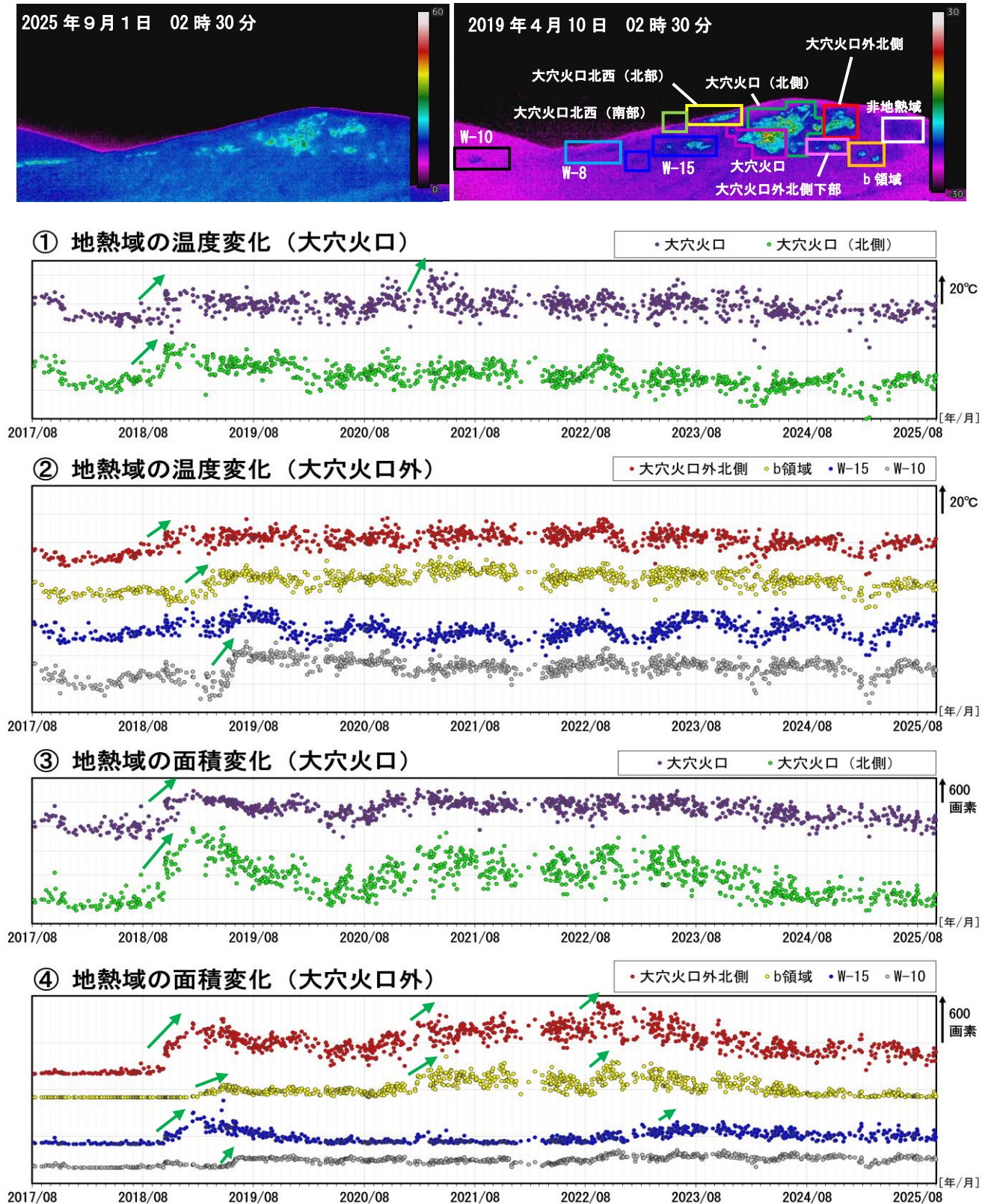
図5 吾妻山 監視カメラによる大穴火口周辺の地熱域の経過（2017年8月～2025年9月）
