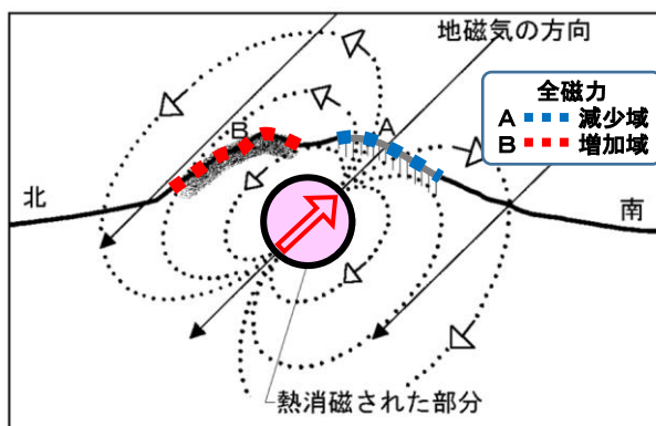
図 7 熱消磁に伴う全磁力変化のモデル
