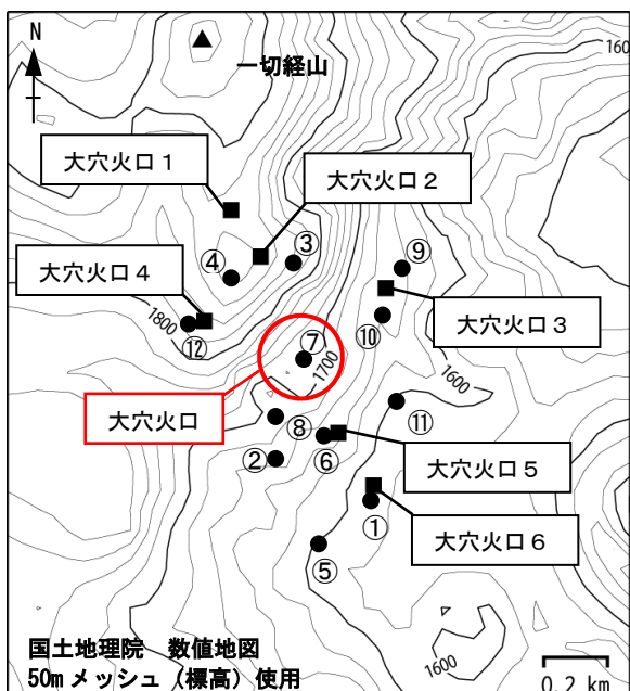
図 10 吾妻山 全磁力観測点配置図
