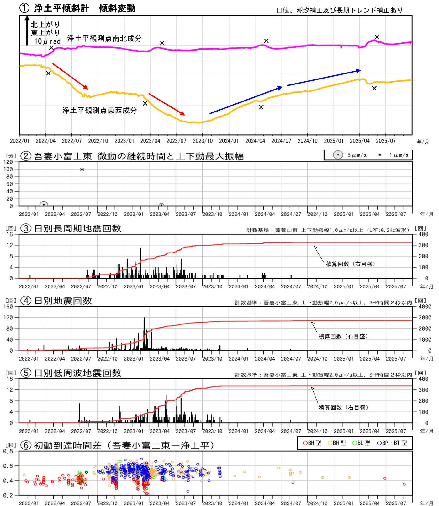
図3 吾妻山 火山活動経過図（2022年1月～2025年9月）
