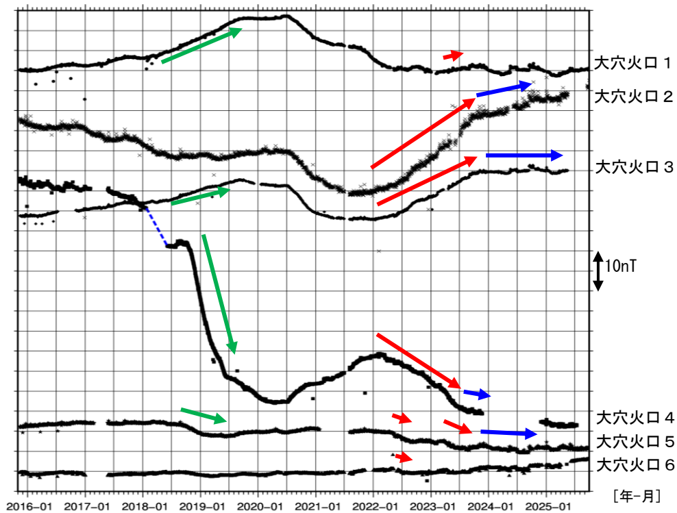
図 6 吾妻山 全磁力連続観測点の全磁力値変化（2015 年 11 月～2025 年 9 月）
