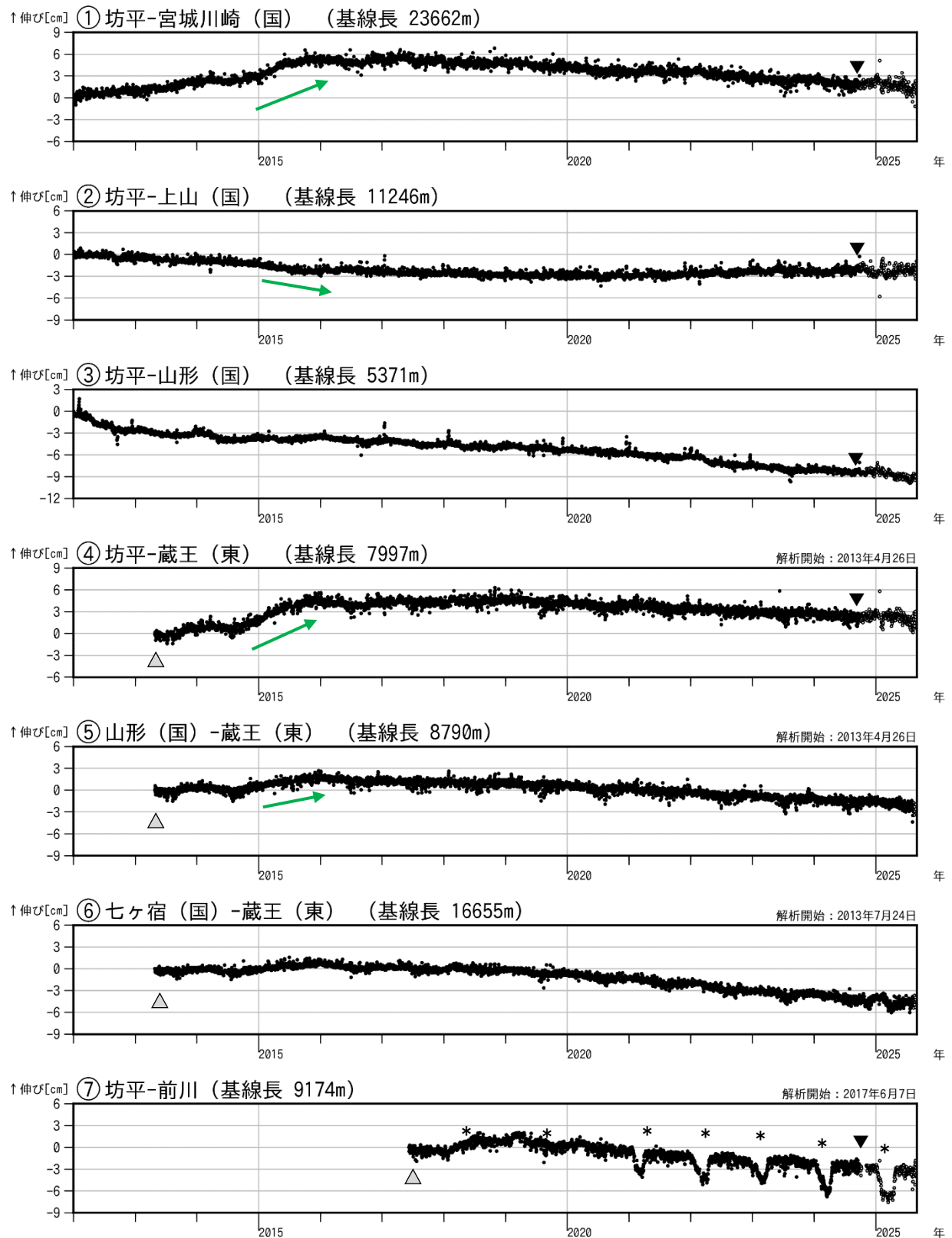
図5 蔵王山 GNSS 基線長変化図 (2012 年 1 月～2025 年 9 月)
