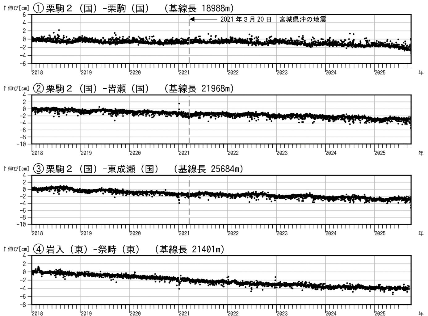
図4 栗駒山 GNSS 基線長変化図（2018年1月～2025年9月）
