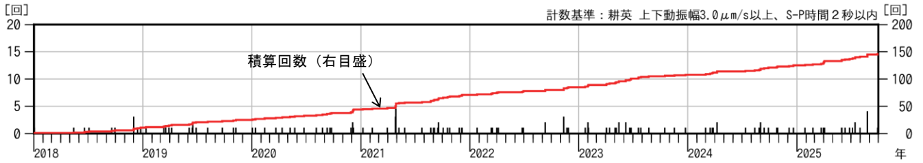
図3 栗駒山 日別地震回数（2018年1月～2025年9月）
