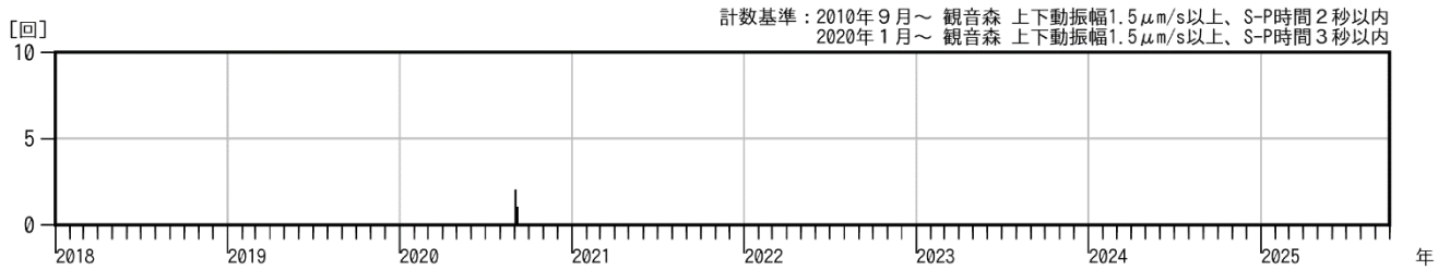
図3 鳥海山 火山性地震の日別回数（2018年1月～2025年9月）
