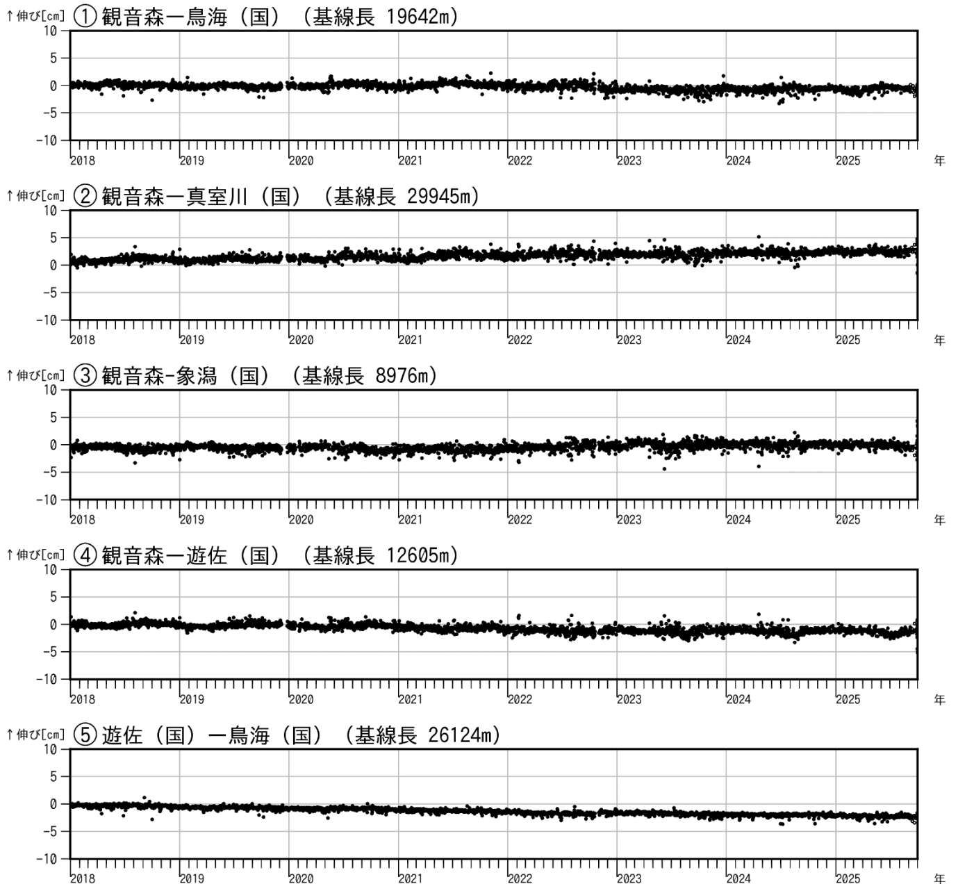
図4 鳥海山 GNSS 基線長変化図（2018年1月～2025年9月）
