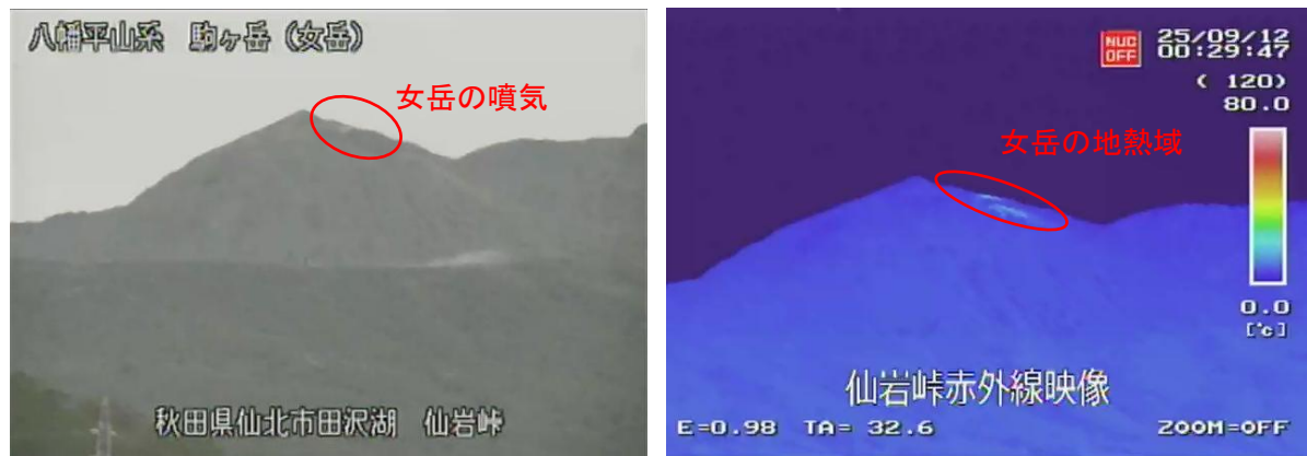
図1 秋田駒ヶ岳 女岳周辺の状況（9月11日）と地表面温度分布の状況（9月12日） ・東北地方整備局が設置している仙岩峠監視カメラ（女岳山頂の南約5km）の可視及び赤外映像です。
