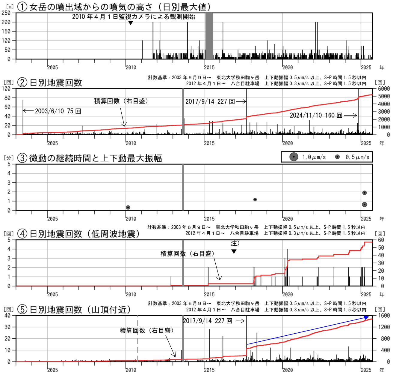
図 2 秋田駒ヶ岳 火山活動経過図（2003 年 6 月～2025 年 9 月）
