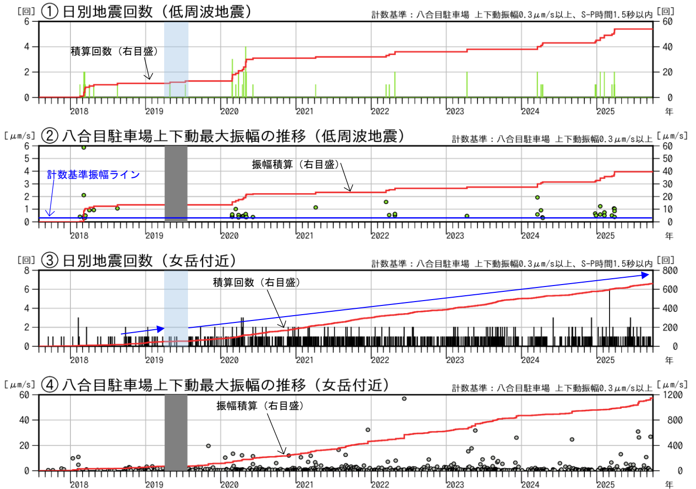
図3 秋田駒ヶ岳 低周波地震及び女岳付近の日別回数と最大振幅（2017年8月～2025年9月）
