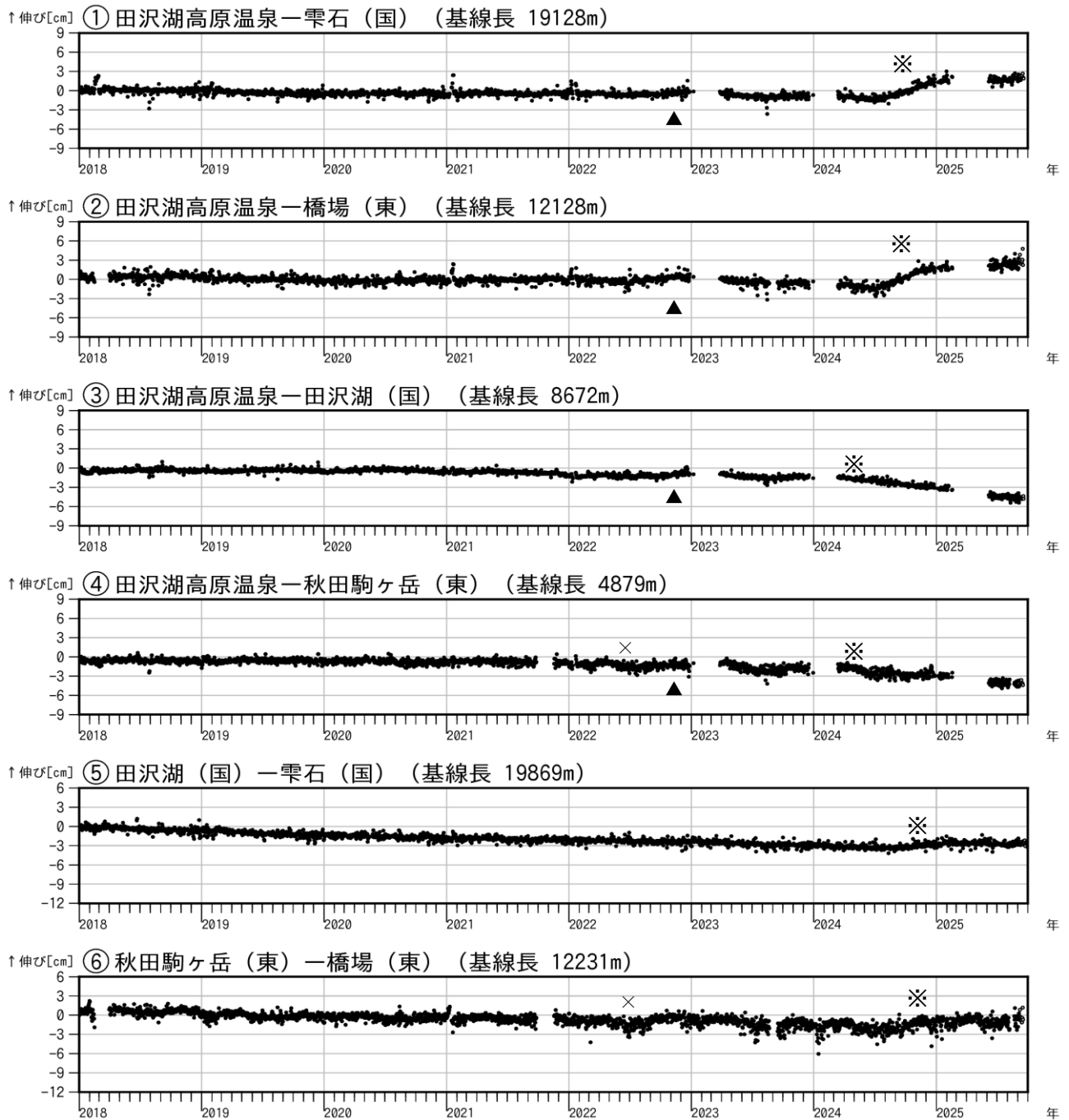
図5 秋田駒ヶ岳 GNSS 基線長変化図（2018年1月～2025年9月）
