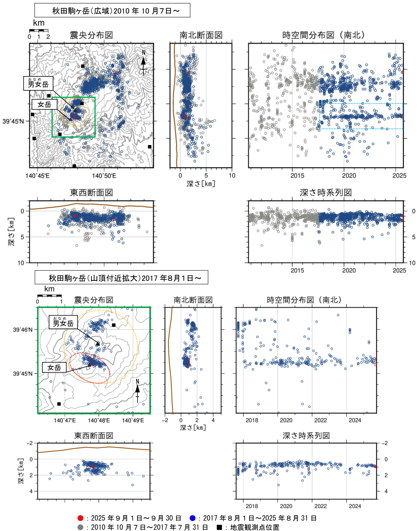
図4 秋田駒ヶ岳 地震活動（2010年10月7日～2025年9月）
