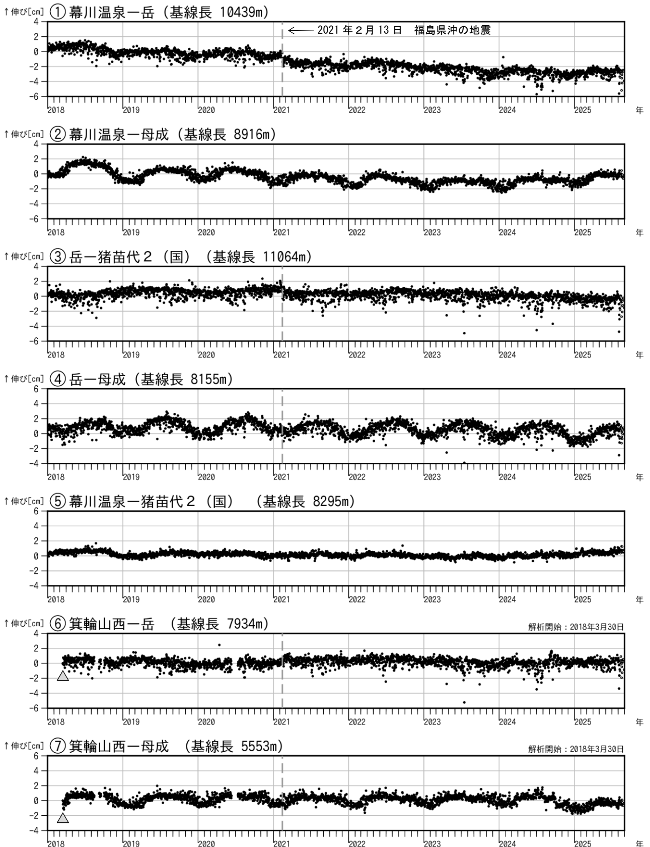
図4 安達太良山 GNSS 基線長変化図（2018年1月～2025年8月）
