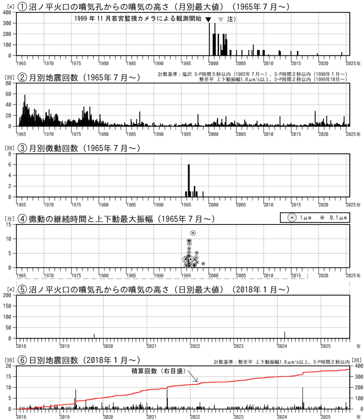
図3 安達太良山 火山活動経過図（1965年7月～2025年8月）
