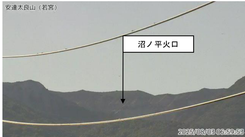
図1 安達太良山 沼ノ平火口周辺の状況（8月3日） ・若宮監視カメラ（沼ノ平火口の西北西約8 km）の映像です。
