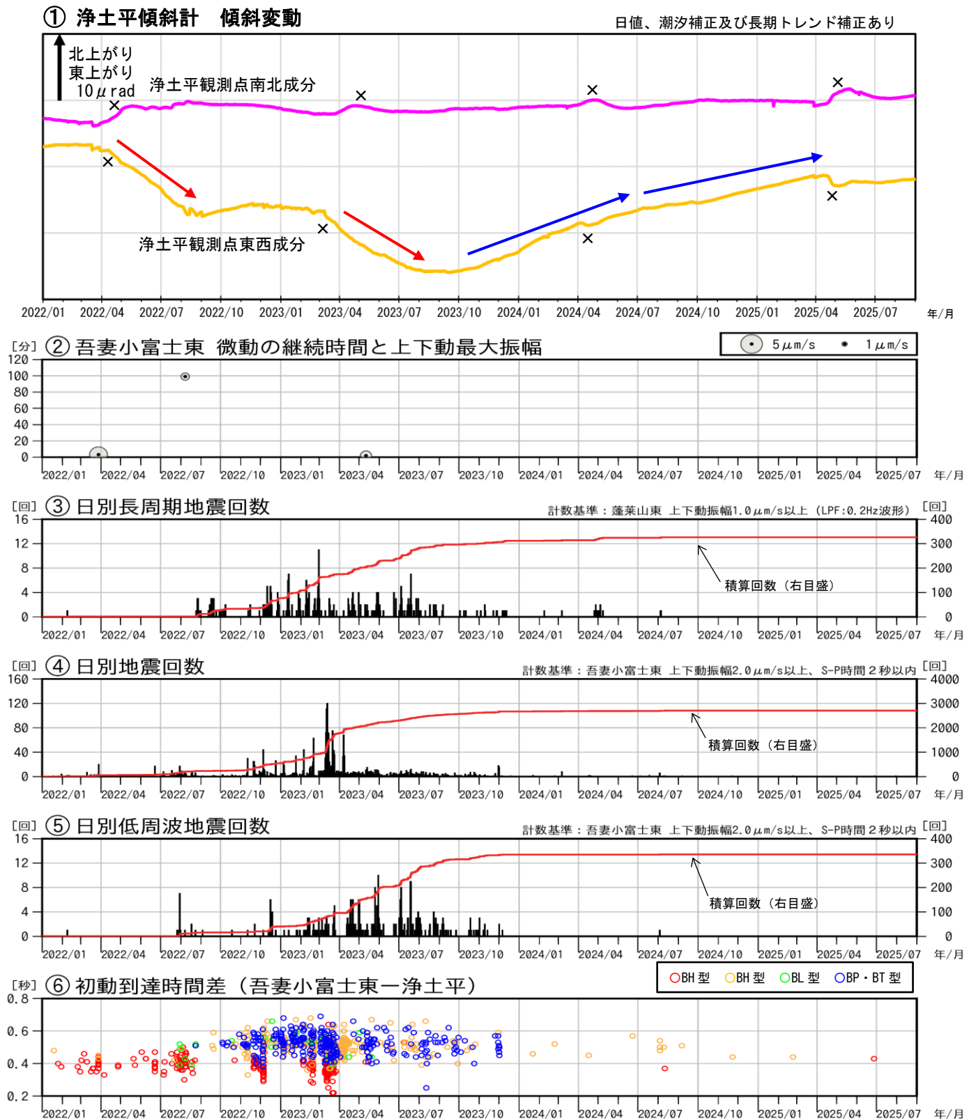
図3 吾妻山 火山活動経過図（2022年1月～2025年8月）
