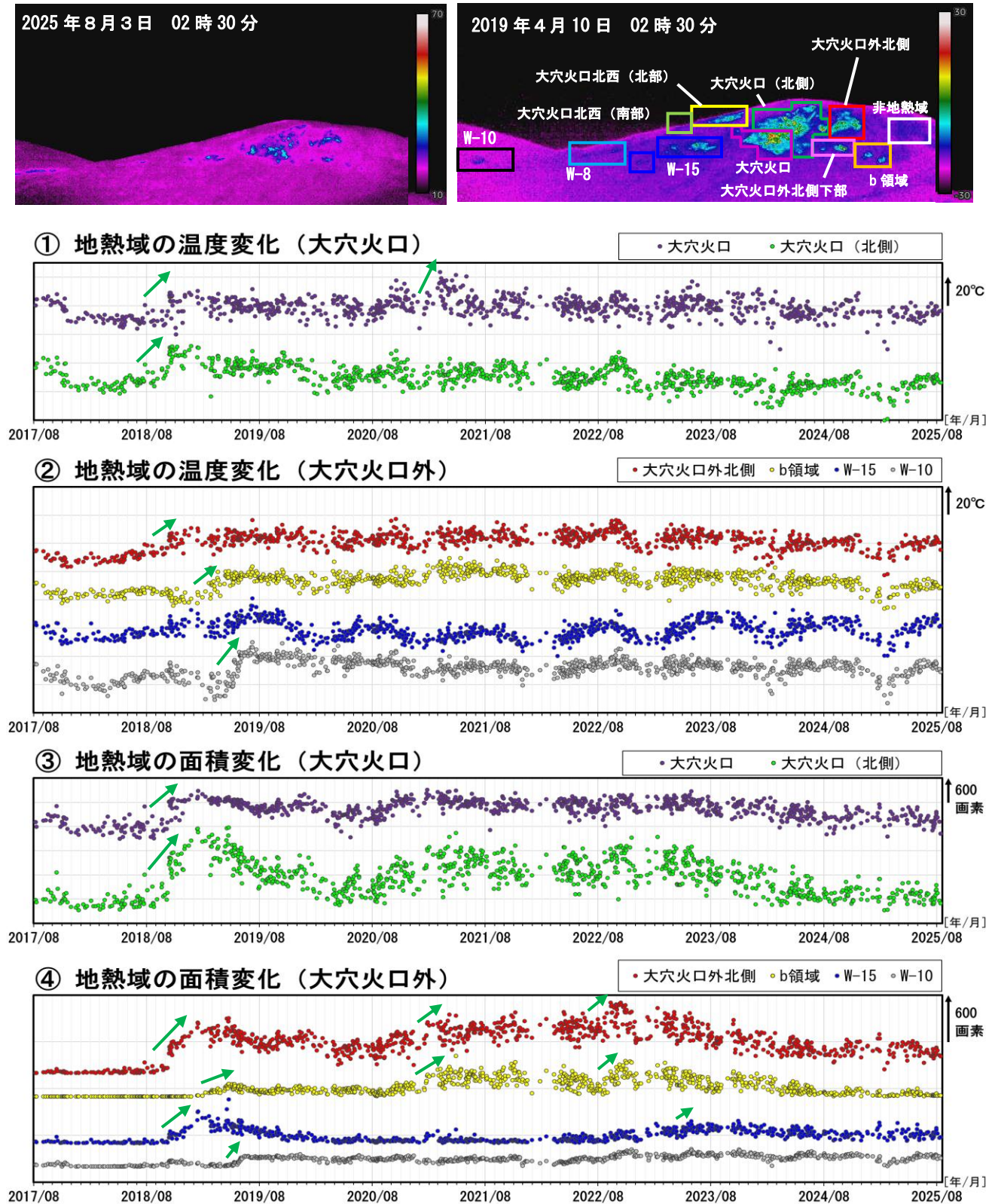
図5 吾妻山 監視カメラによる大穴火口周辺の地熱域の経過（2017年8月～2025年8月）
