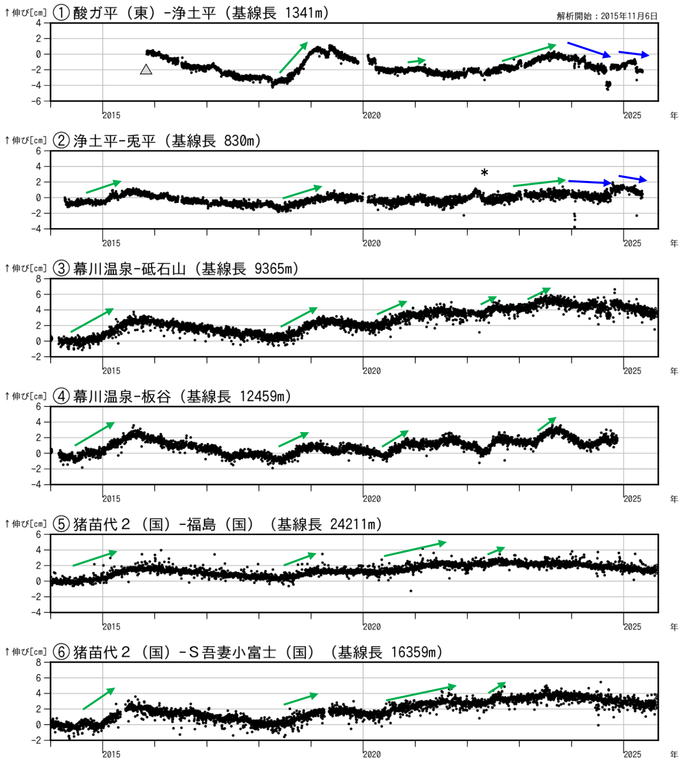
図4 吾妻山 吾妻山浅部・深部の地殻変動（2014年1月～2025年8月）
