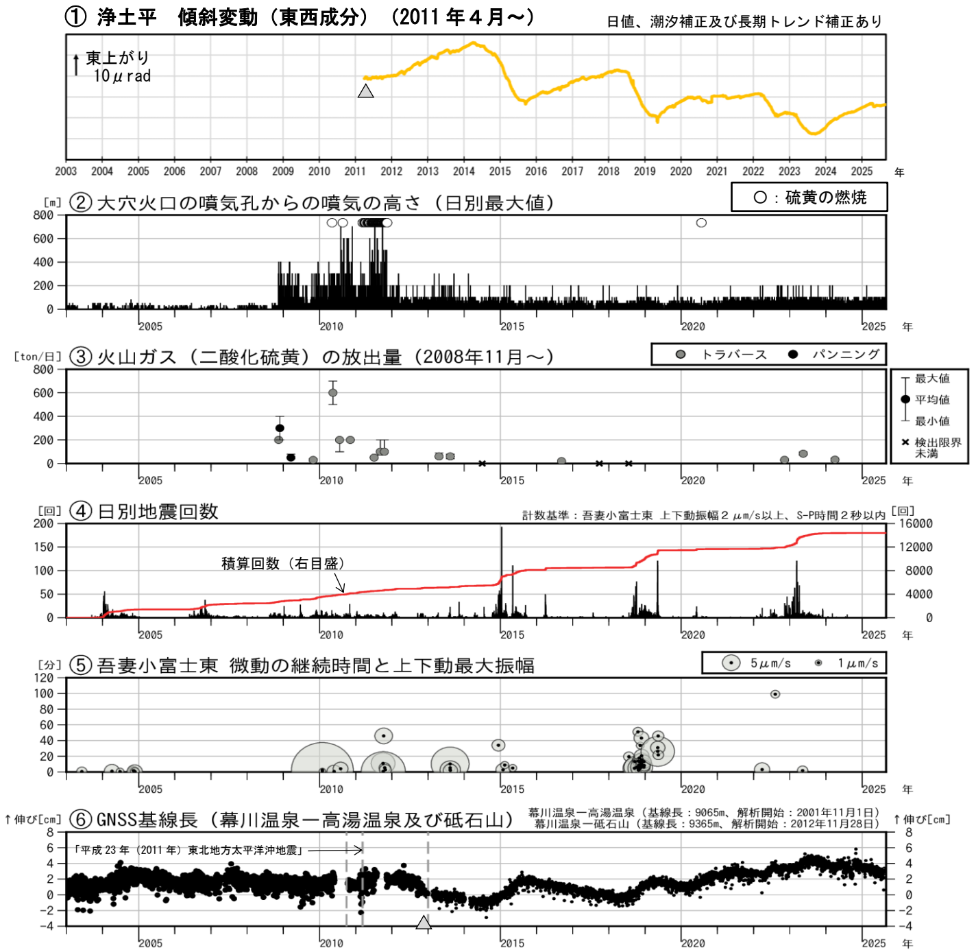
図2 吾妻山 中期的な火山活動の経過（2003年1月～2025年8月）
