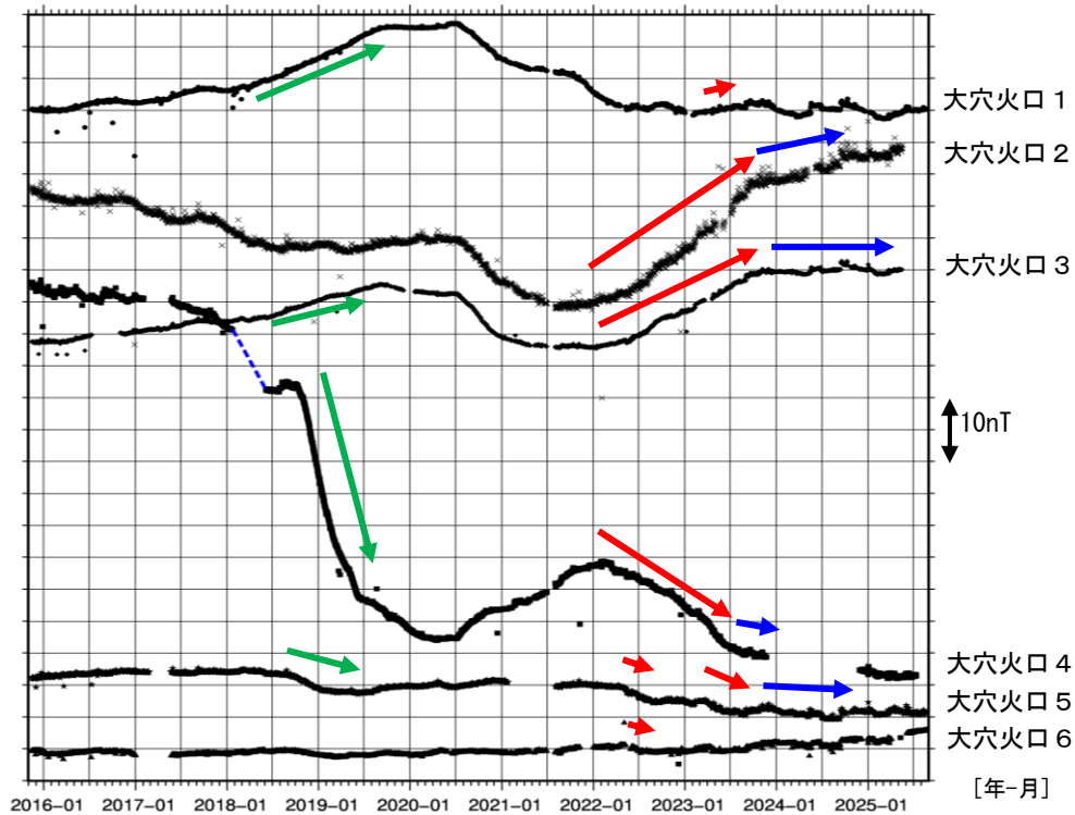
図6 吾妻山 全磁力連続観測点の全磁力値変化（2015年11月～2025年8月）
