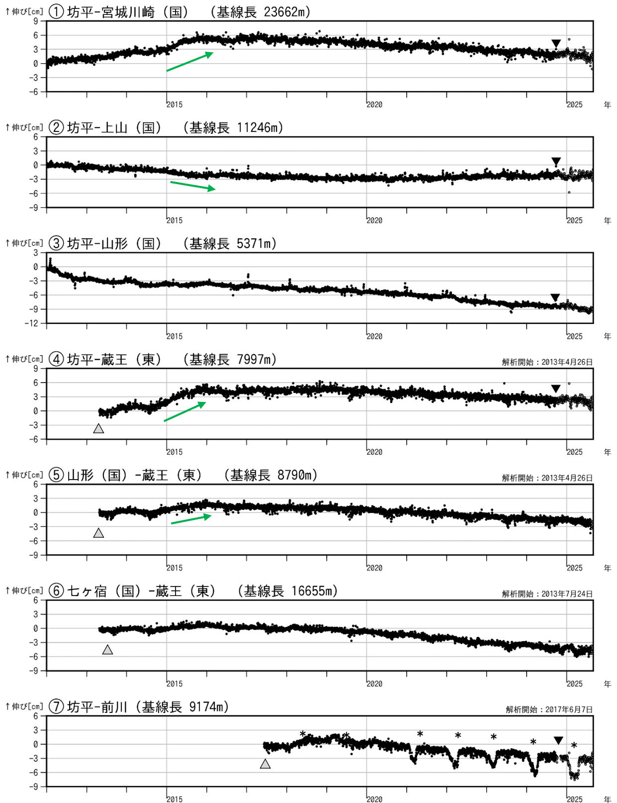
図3 蔵王山 GNSS 基線長変化図（2012年1月～2025年8月）
