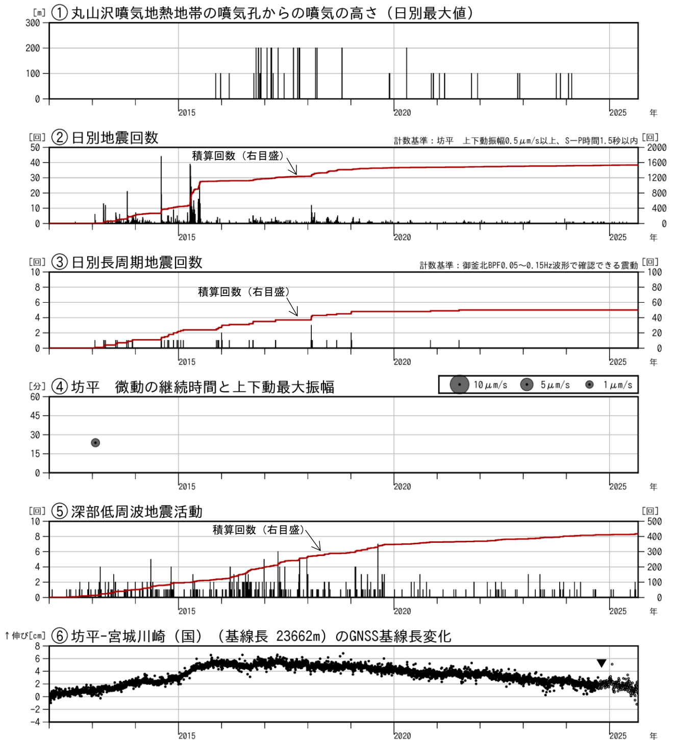
図2 蔵王山 火山活動経過図（2012年1月～2025年8月）
