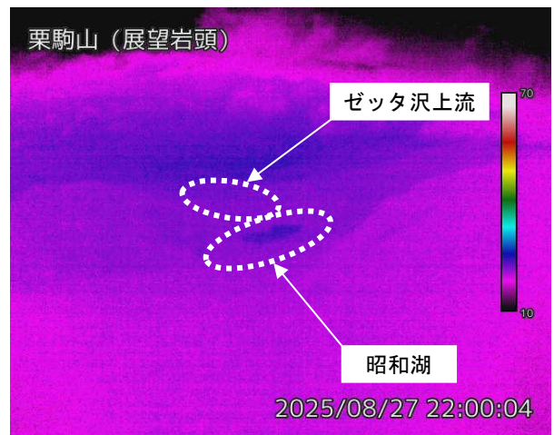
図2 栗駒山 昭和湖及びゼッタ沢上流周辺の状況（8月23日）と地表面温度分布（8月27日） ・展望岩頭監視カメラ（昭和湖の南南西約900m）の映像です。 ※8月26日に実施した改修作業により、地表面温度分布の画角が以前とは異なります。
