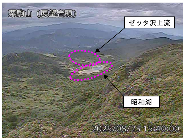
図2 栗駒山 昭和湖及びゼッタ沢上流周辺の状況（8月23日）と地表面温度分布（8月27日） ・展望岩頭監視カメラ（昭和湖の南南西約900m）の映像です。 ※8月26日に実施した改修作業により、地表面温度分布の画角が以前とは異なります。
