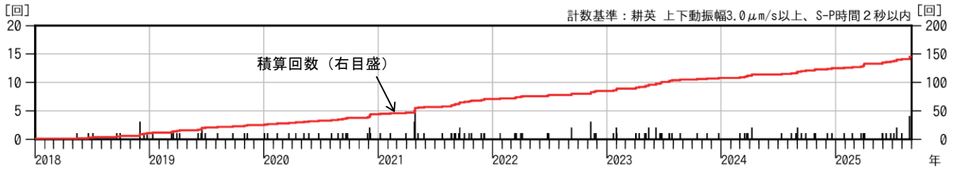
図3 栗駒山 日別地震回数（2018年1月～2025年8月）
