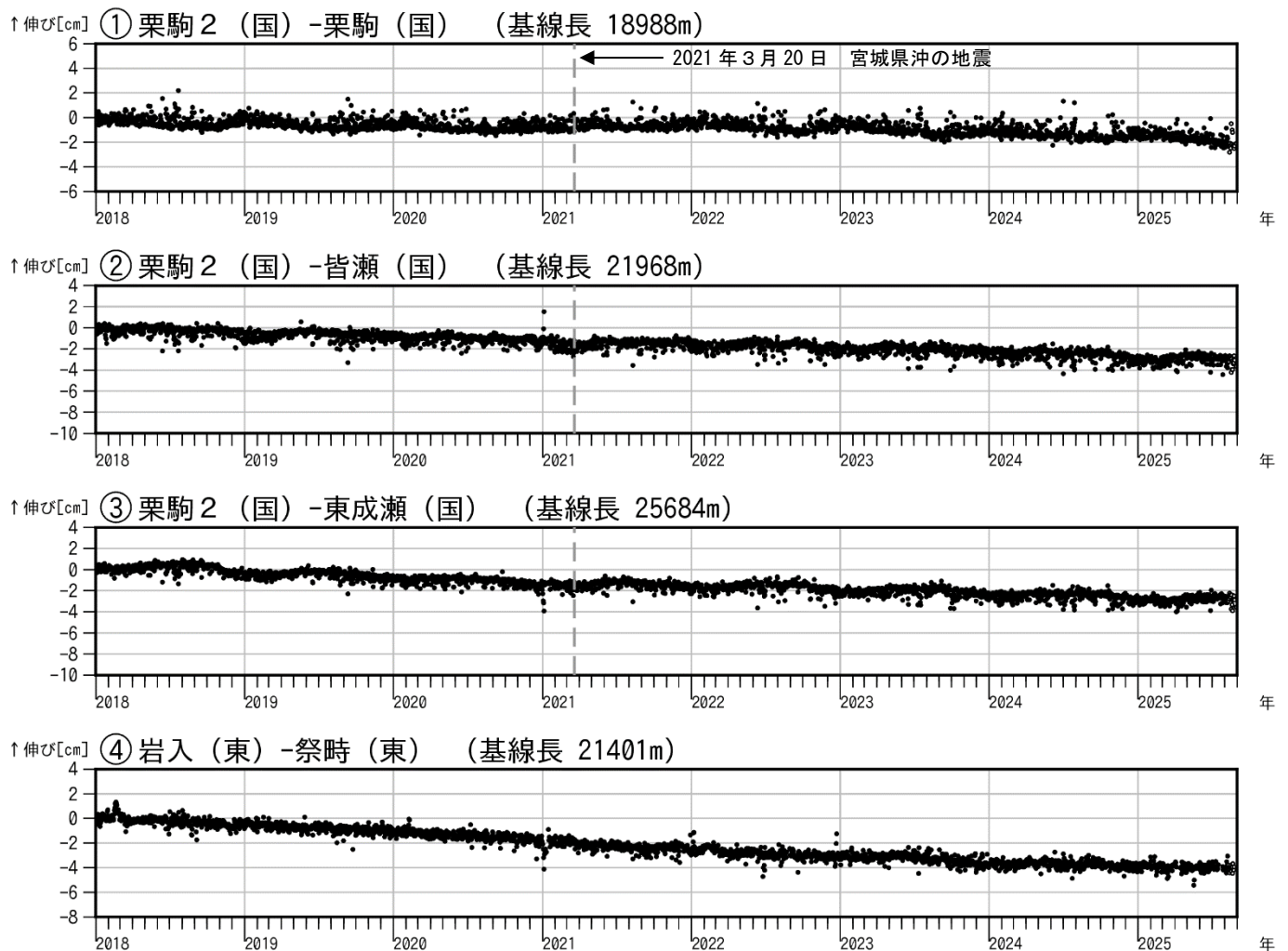
図4 栗駒山 GNSS 基線長変化図（2018年1月～2025年8月）
