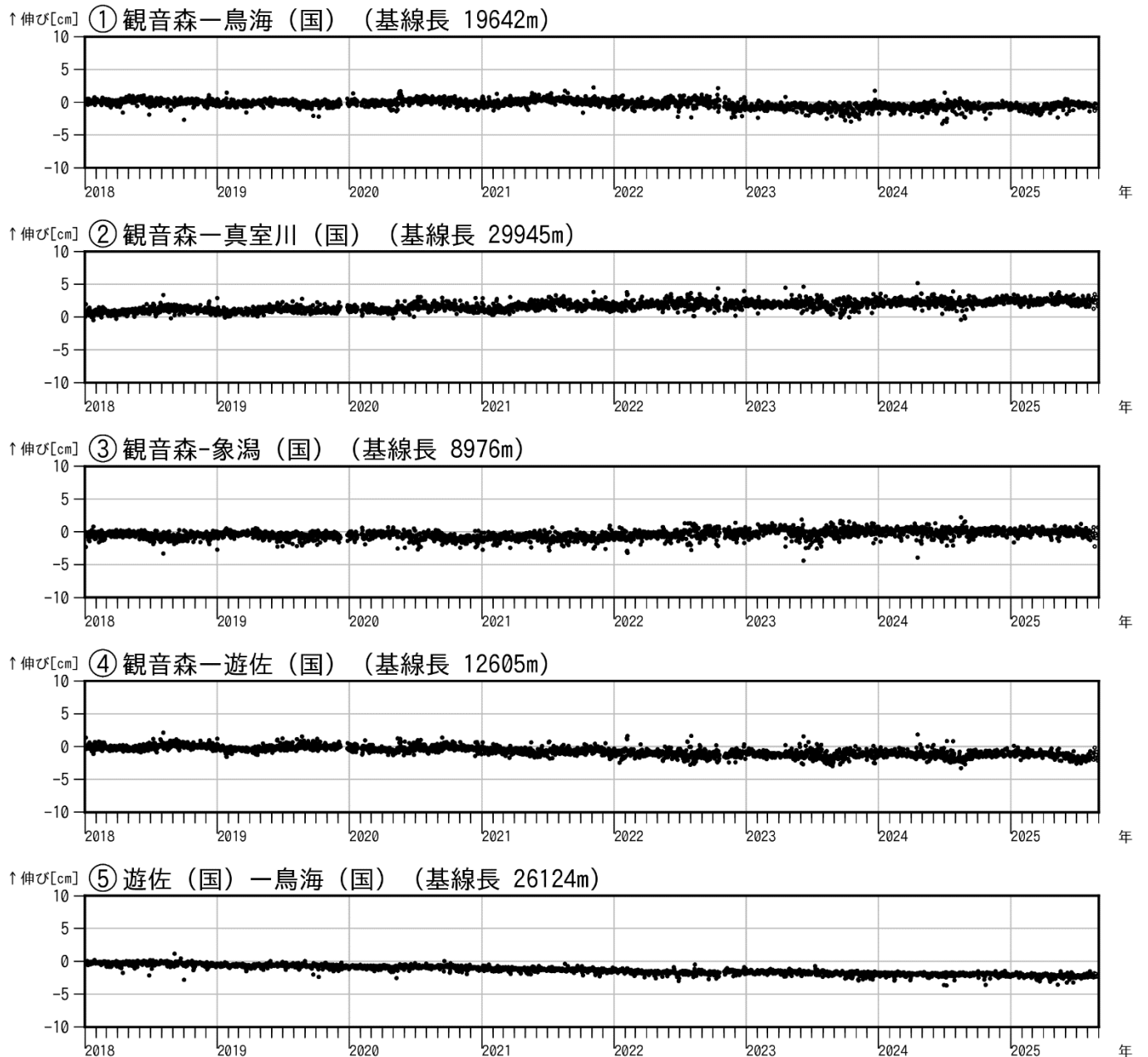
図4 鳥海山 GNSS 基線長変化図（2018年1月～2025年8月）
