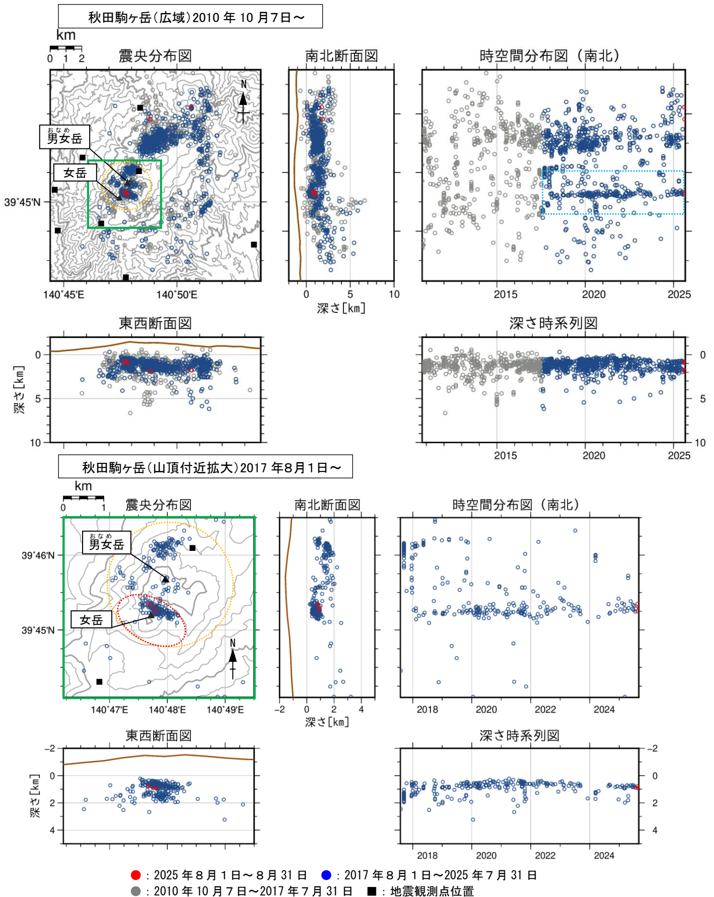
図4 秋田駒ヶ岳 地震活動（2010年10月7日～2025年8月）
