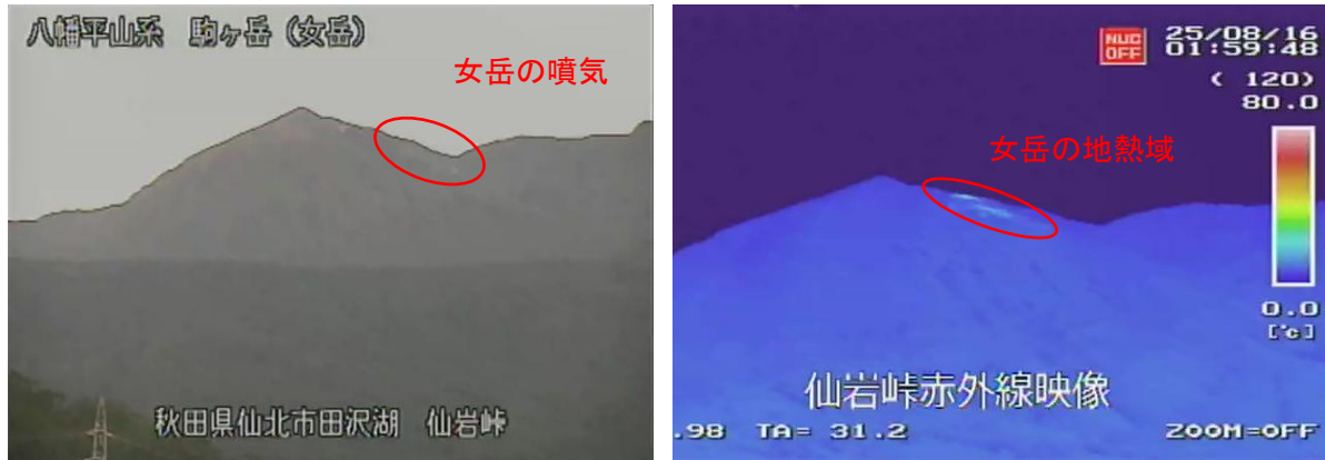
図1 秋田駒ヶ岳 女岳周辺の状況（8月9日）と地表面温度分布の状況（8月16日） ・東北地方整備局が設置している仙岩峠監視カメラ（女岳山頂の南約5km）の可視及び赤外映像です。
