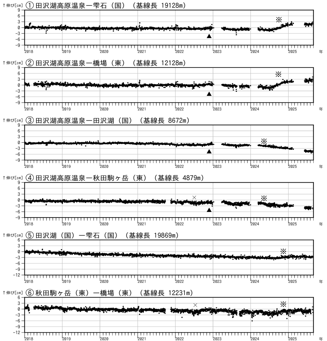
図5 秋田駒ヶ岳 GNSS 基線長変化図（2018年1月～2025年8月）
