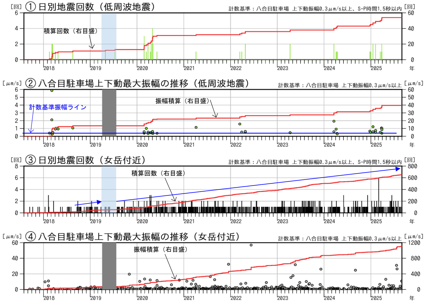
図3 秋田駒ヶ岳 低周波地震及び女岳付近の日別回数と最大振幅（2017年8月～2025年8月）
