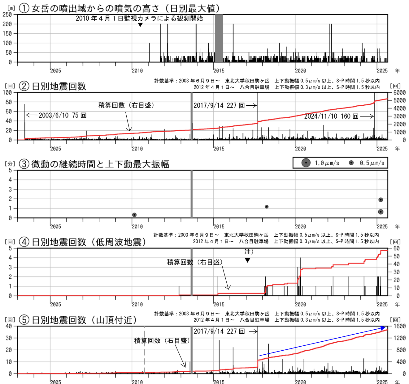
図2 秋田駒ヶ岳 火山活動経過図（2003年6月～2025年8月）
