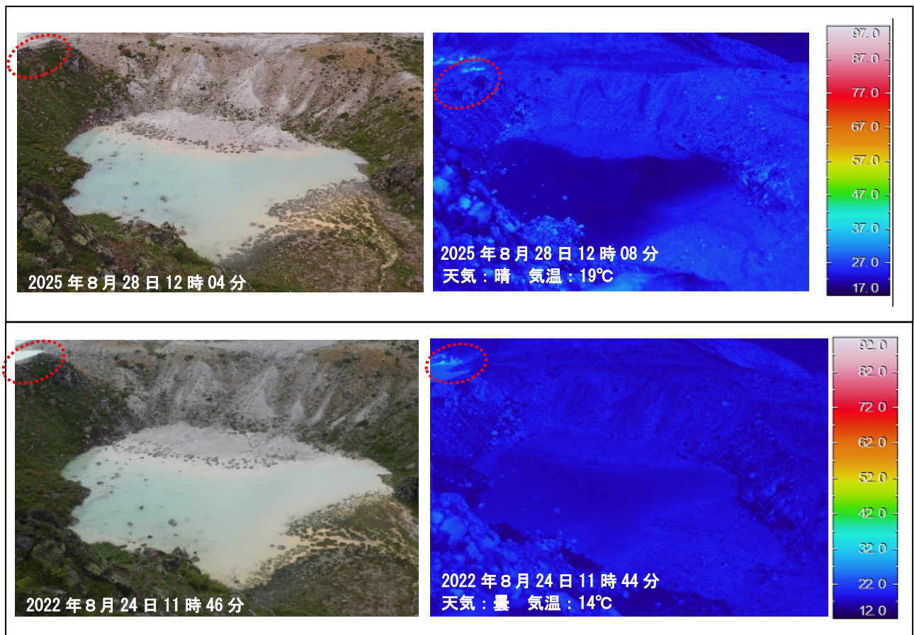
図6 秋田焼山 南から撮影した空沼の状況と地表面温度分布
