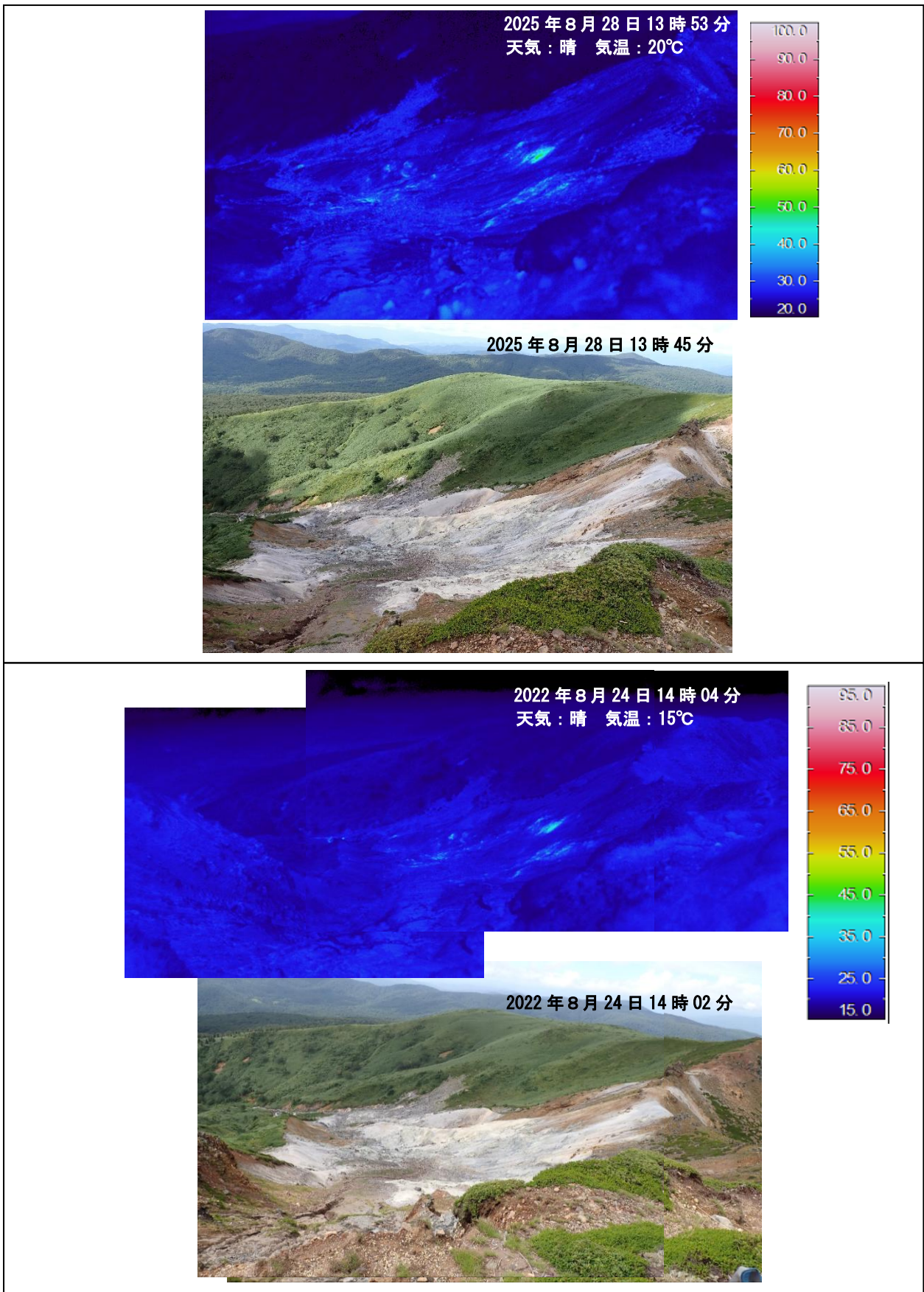
図4 秋田焼山 南東から撮影した叫沢源頭部の状況と地表面温度分布
