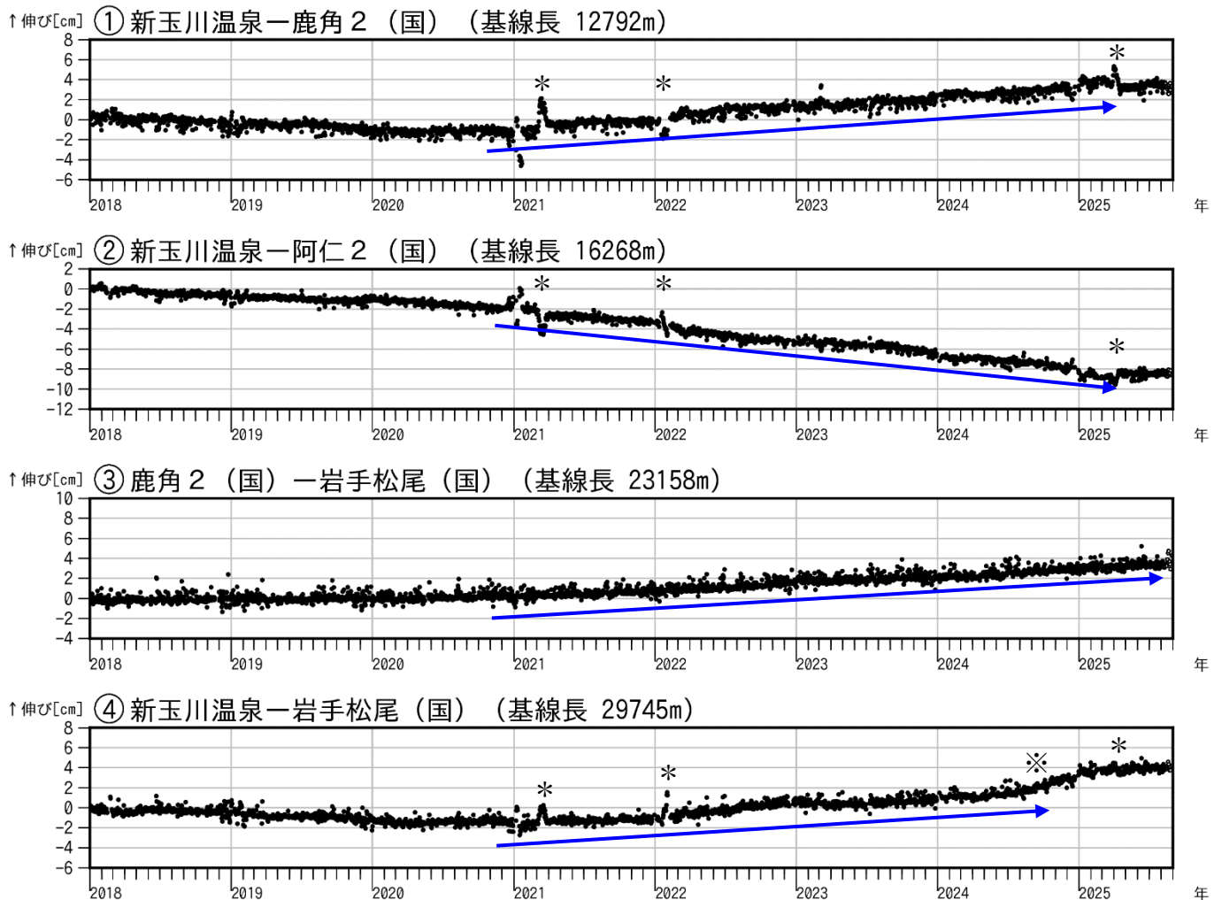
図 8 秋田焼山 GNSS 基線長変化図（2018 年 1 月～2025 年 8 月）
