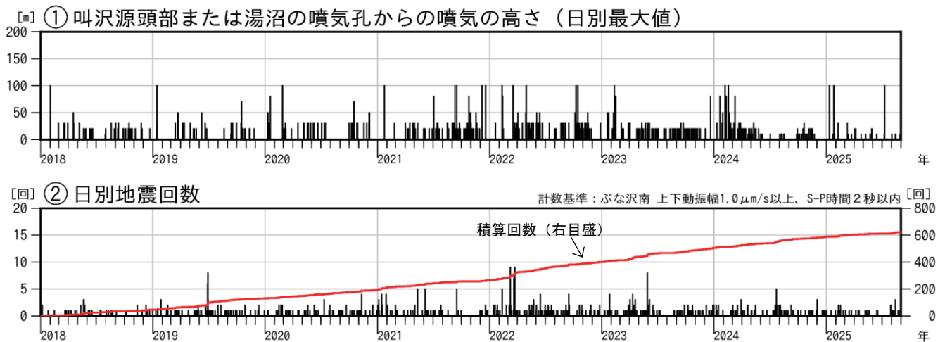
図 7 秋田焼山 火山活動経過図（2018 年 1 月～2025 年 8 月）
