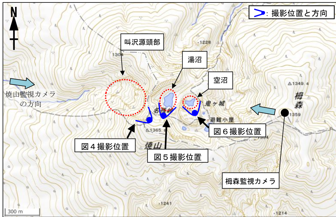
図3 秋田焼山 叫沢源頭部、湯沼及び空沼の写真と地表面温度分布撮影位置
