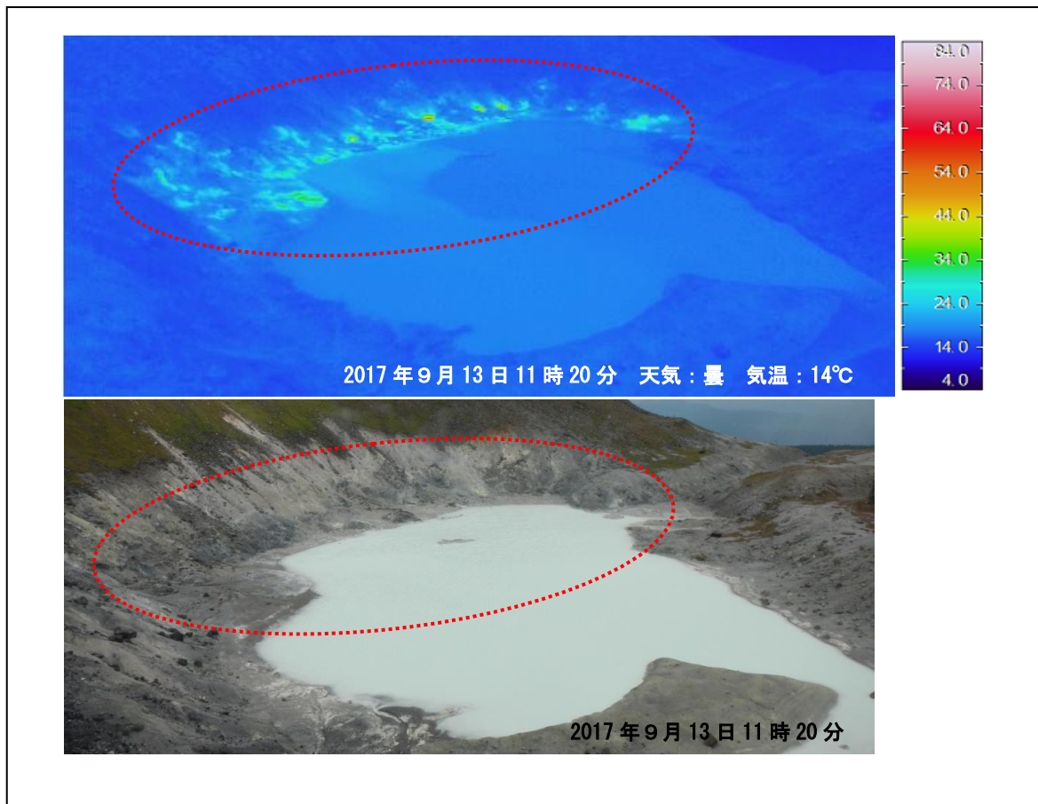
図5 秋田焼山 南から撮影した湯沼の状況と地表面温度分布
