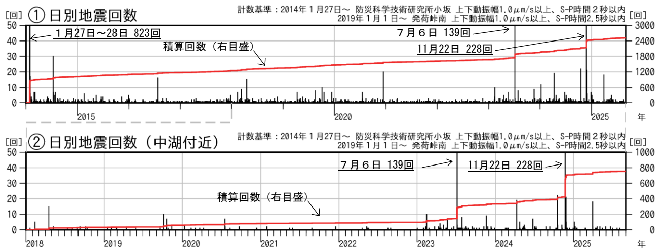
図2 十和田 活動経過図（2014年1月～2025年8月）
