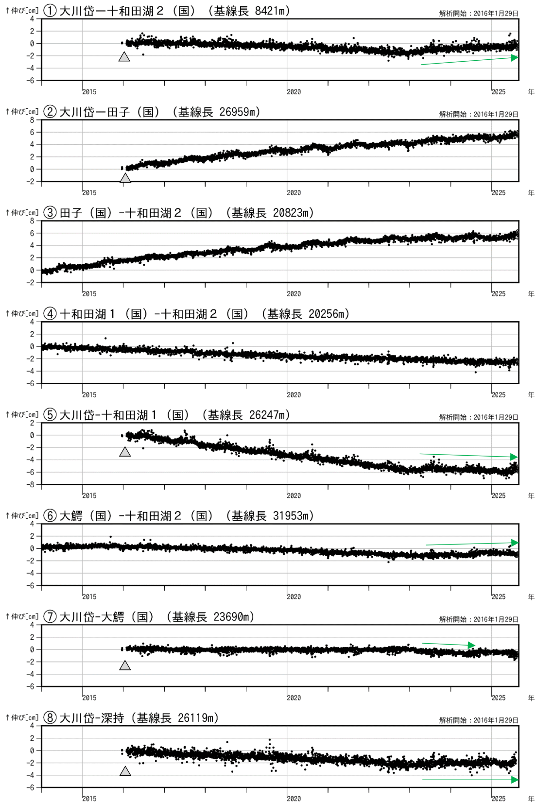
図3 十和田 GNSS 基線長変化図 (2014 年 1 月~2025 年 8 月)
