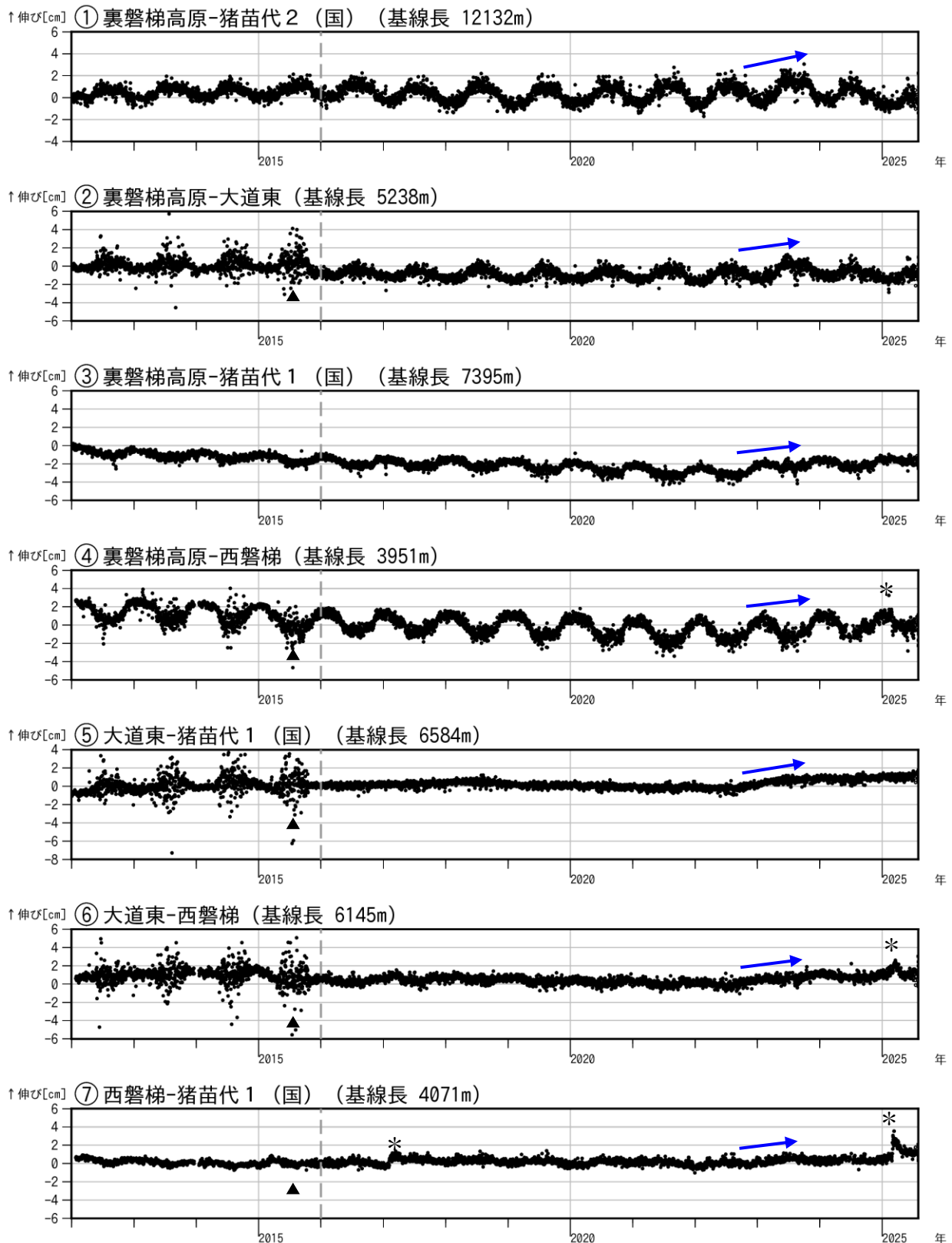
図 6 磐梯山 GNSS 基線長変化図 (2012 年 1 月～2025 年 7 月)
