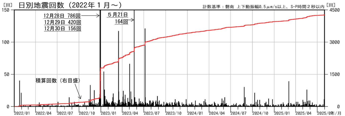
図4 磐梯山 地震回数（2022年1月～2025年7月）
