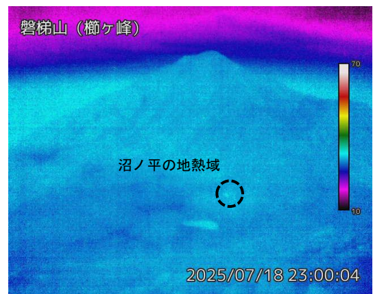
図2 磐梯山 沼ノ平周辺の状況と地表面温度分布（7月18日）
