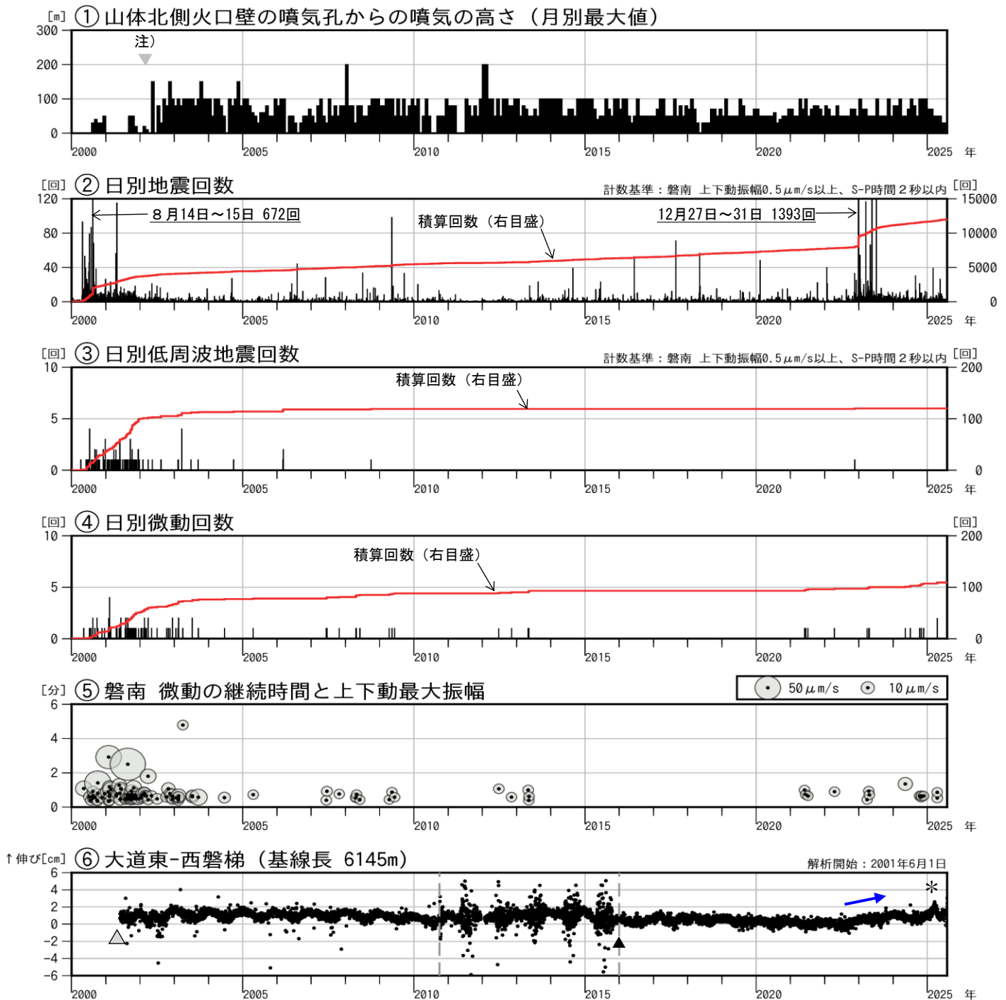
図3 磐梯山 火山活動経過図（2000年1月～2025年7月）
