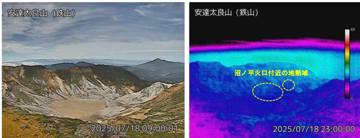
図2 安達太良山 沼ノ平火口周辺の状況と地表面温度分布の状況（7月18日）
