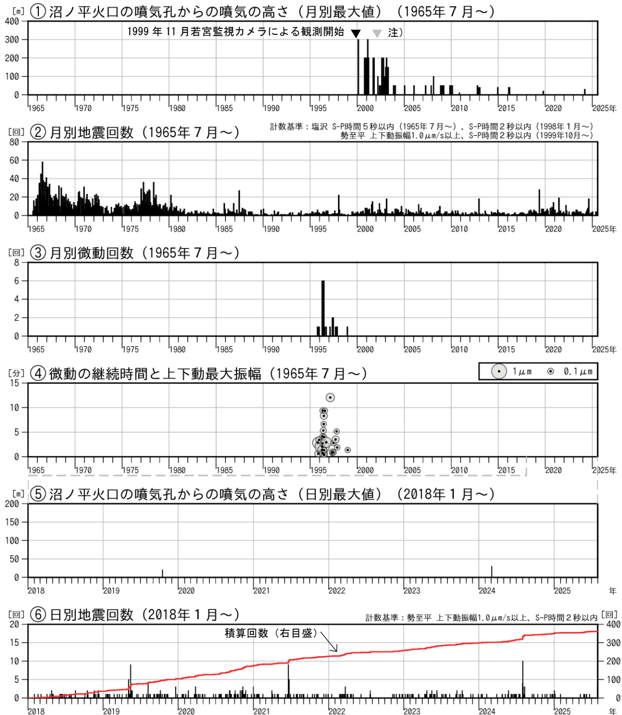
図3 安達太良山 火山活動経過図（1965年7月～2025年7月）
