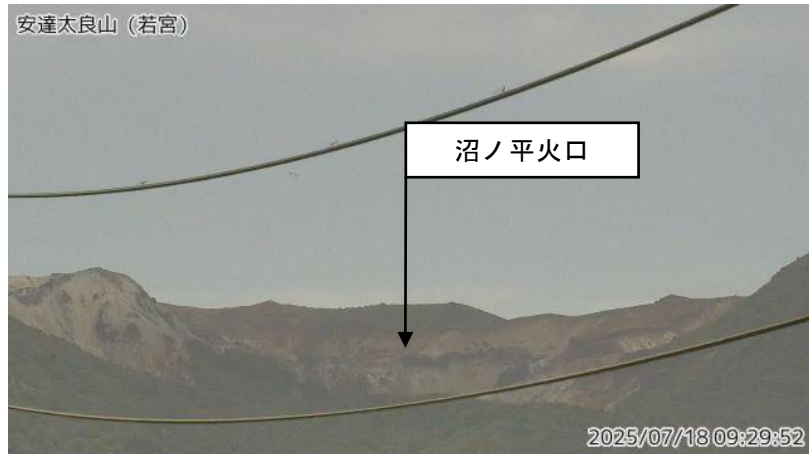
図1 安達太良山 沼ノ平火口周辺の状況（7月18日）
