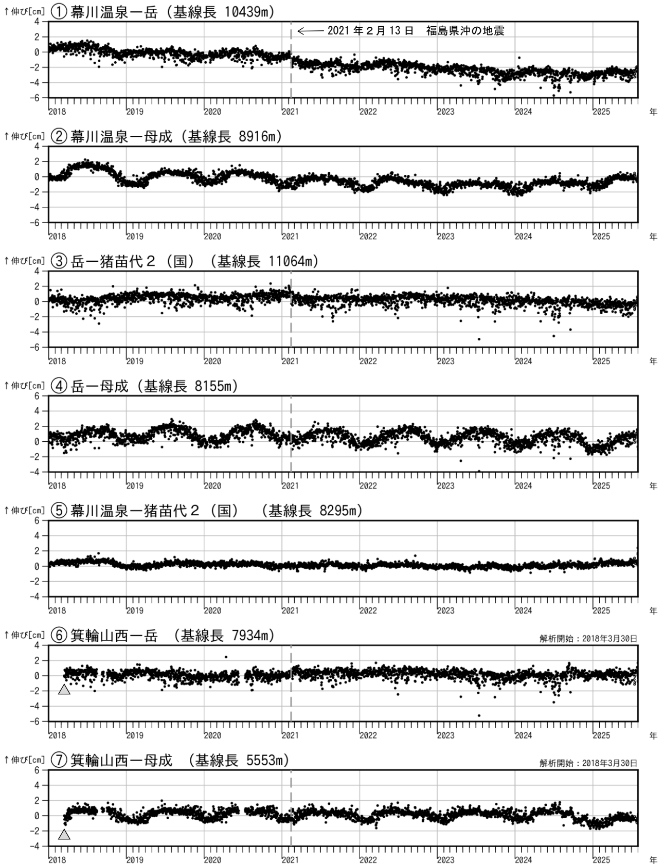
図4 安達太良山 GNSS 基線長変化図（2018年1月～2025年7月）
