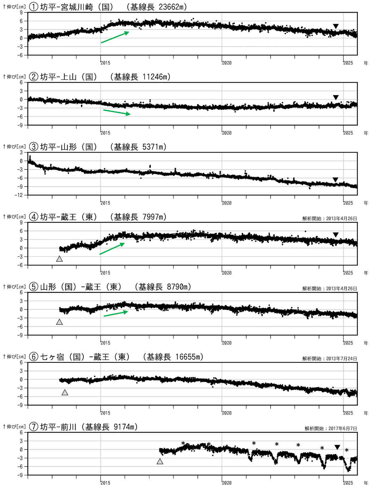
図3 蔵王山 GNSS 基線長変化図 (2012 年 1 月～2025 年 7 月)
