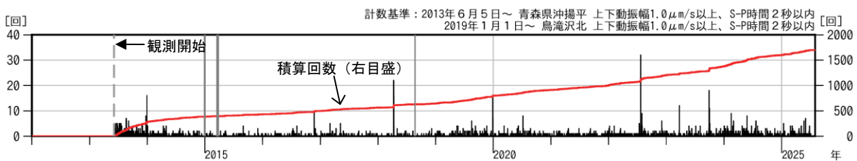
図2 八甲田山 日別地震回数（2013年6月～2025年7月）
