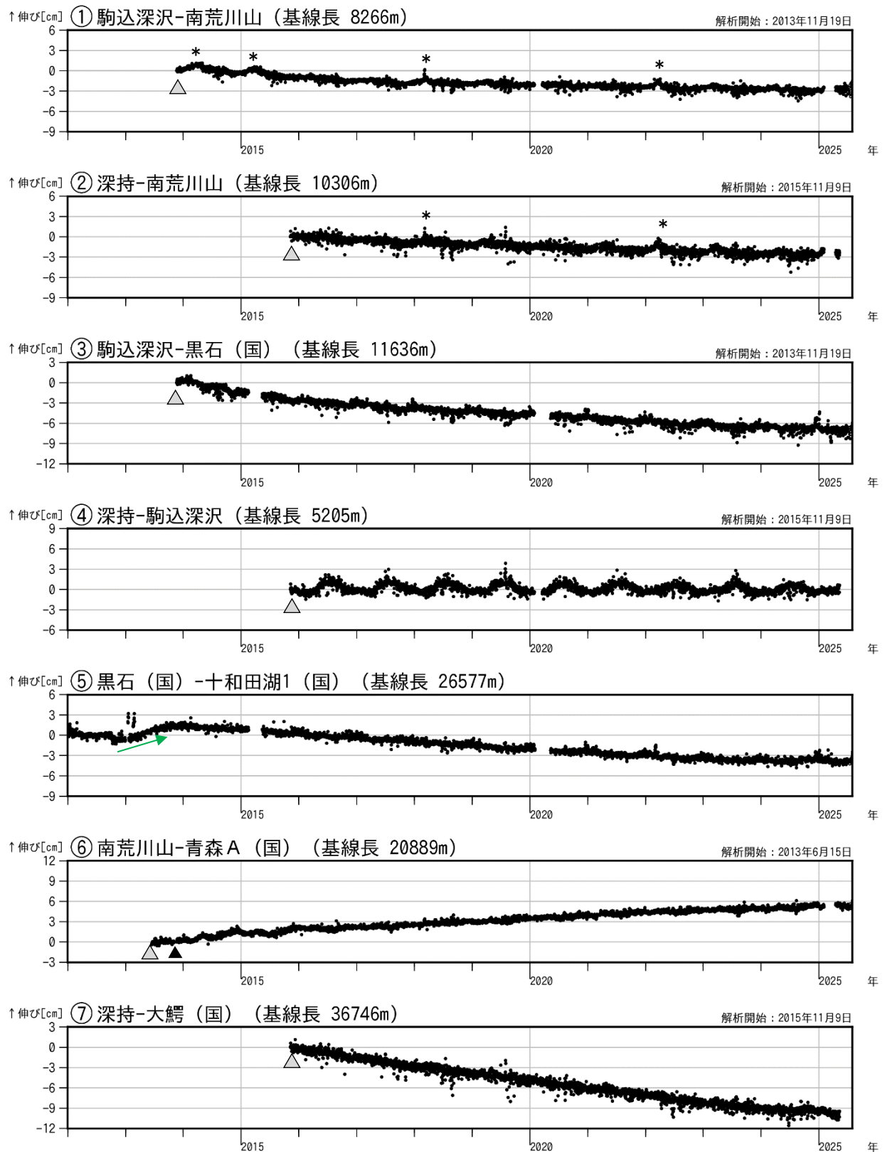
図3 八甲田山 GNSS 基線長変化図（2012年1月～2025年7月）
