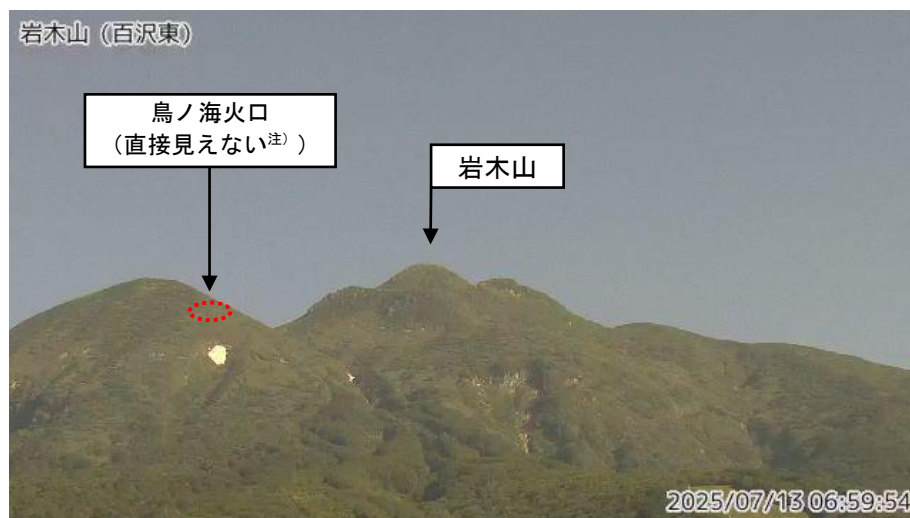
図1 岩木山 山頂部の状況（7月13日）
