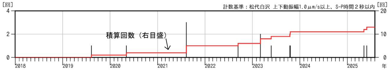
図2 岩木山 日別地震回数（2018年1月～2025年7月）
