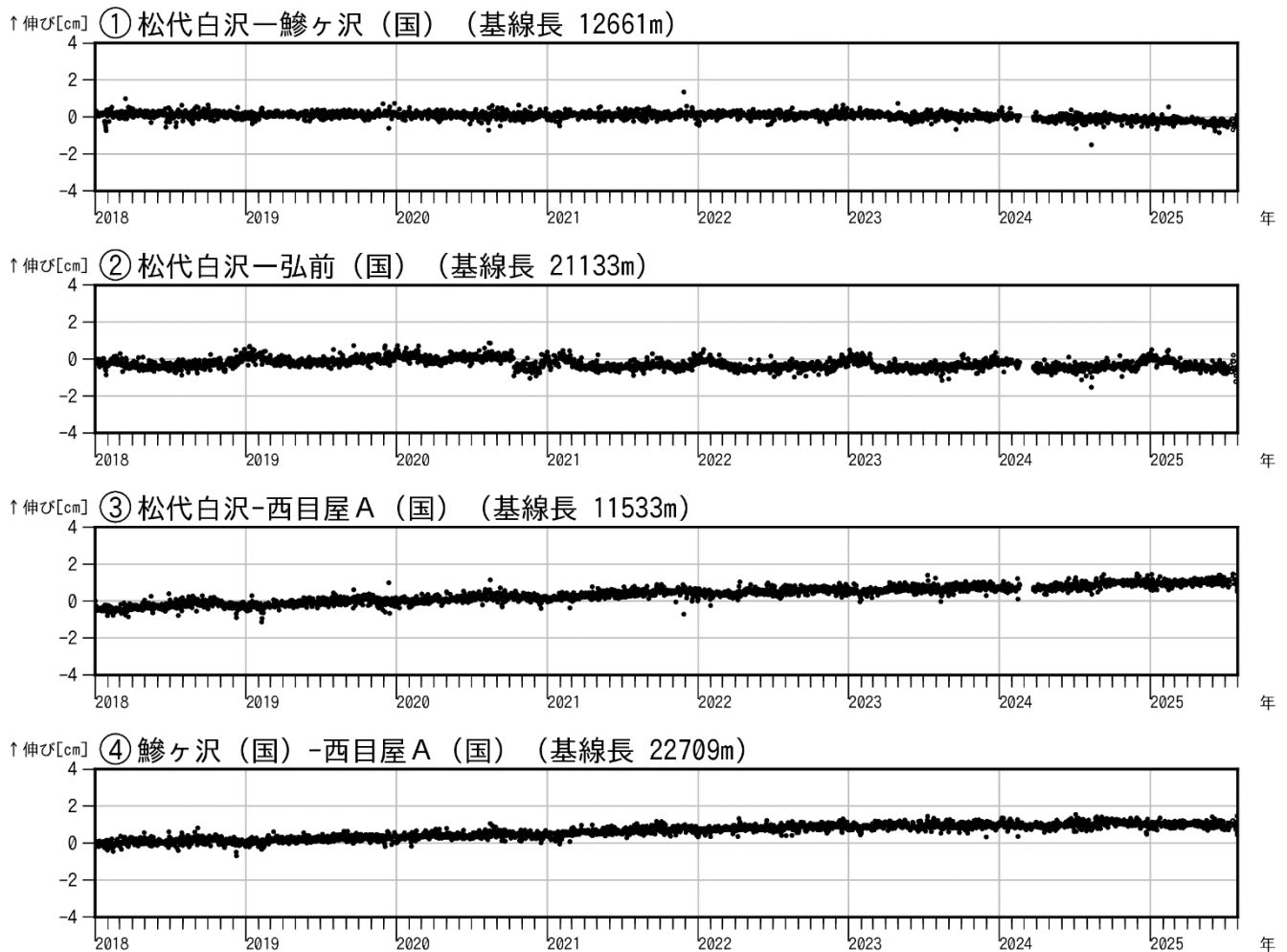
図3 岩木山 GNSS 基線長変化図（2018年1月～2025年7月）
