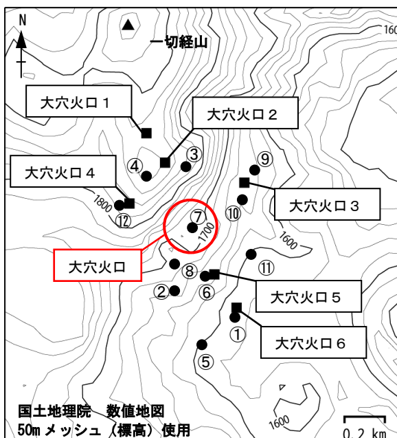
図10 吾妻山 全磁力観測点配置図
