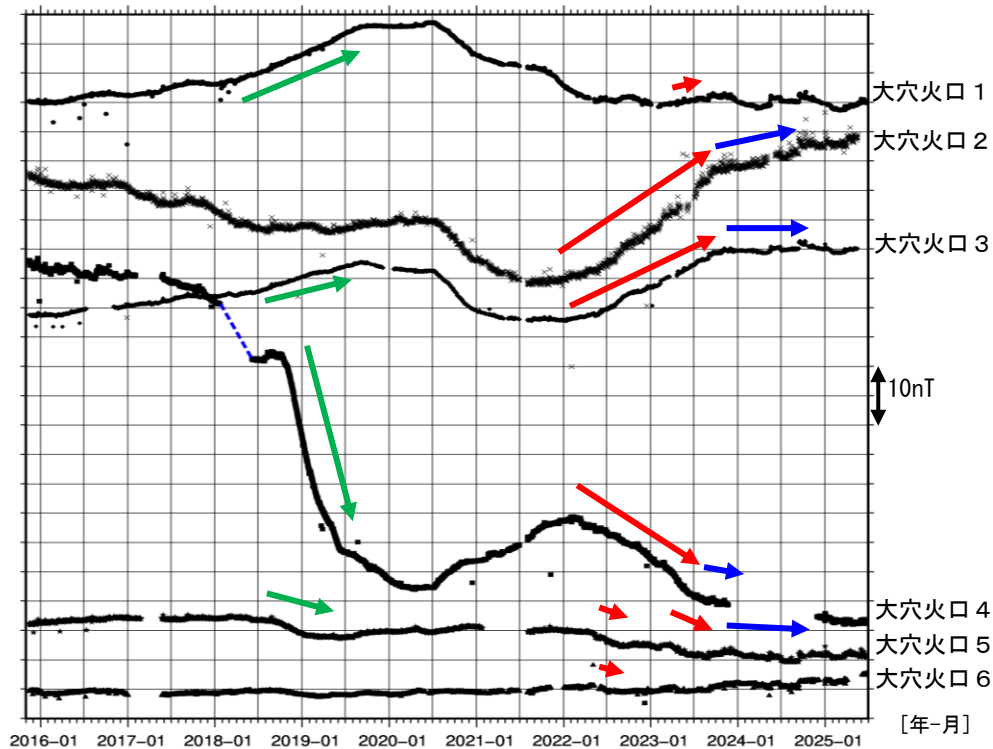
図6 吾妻山 全磁力連続観測点の全磁力値変化（2015年11月～2025年6月）
