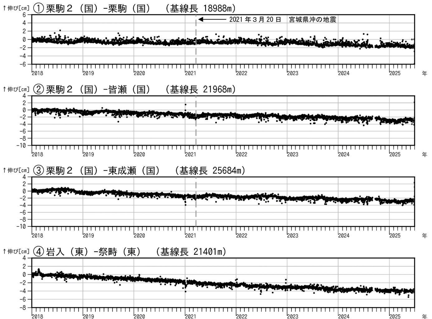
図3 栗駒山 GNSS 基線長変化図（2018年1月～2025年6月）
