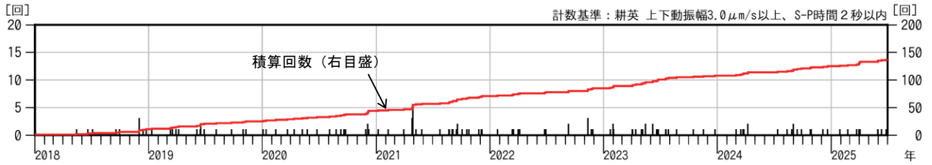
図2 栗駒山 日別地震回数（2018年1月～2025年6月）
