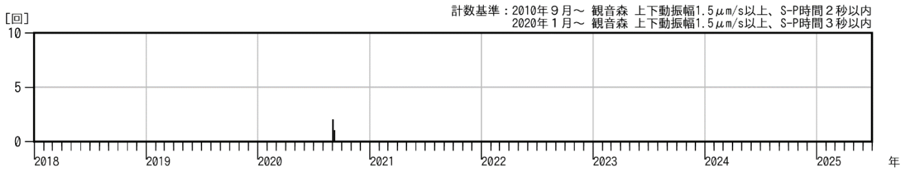
図3 鳥海山 火山性地震の日別回数（2018年1月～2025年6月）
