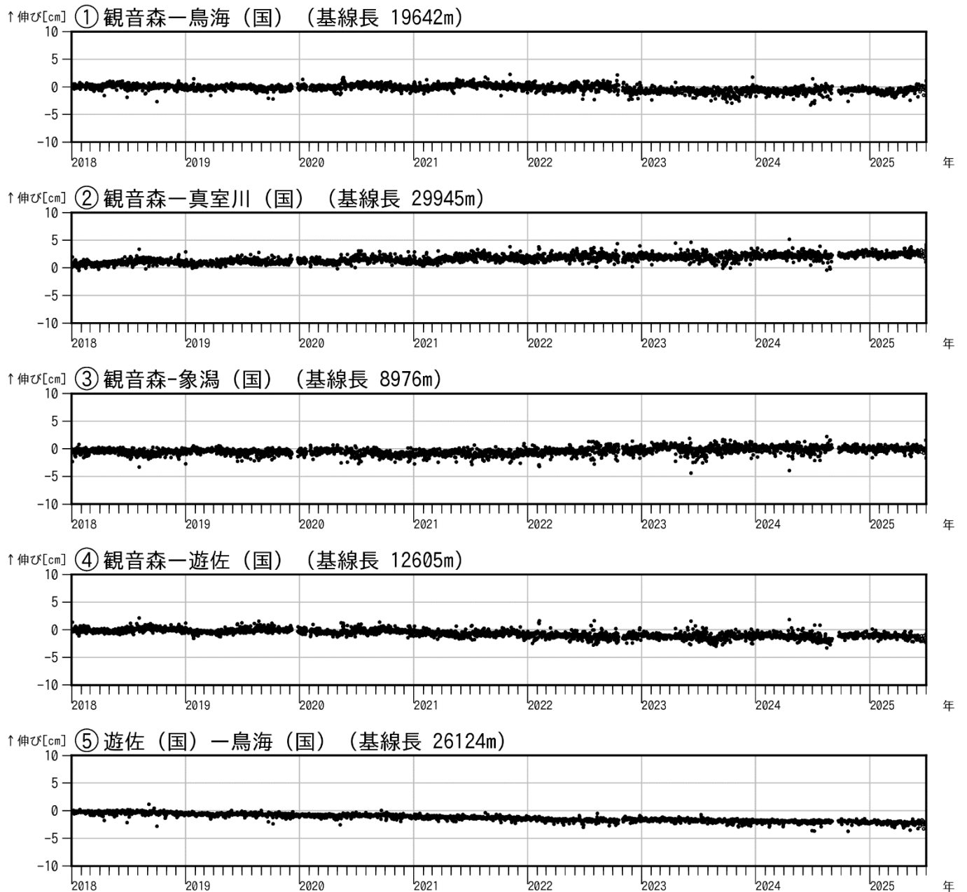
図4 鳥海山 GNSS 基線長変化図（2018年1月～2025年6月）
