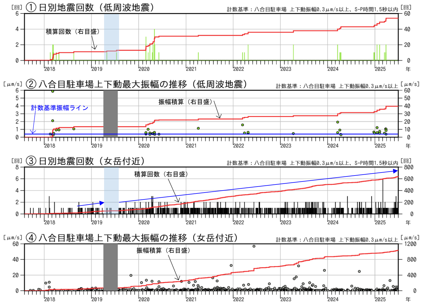
図3 秋田駒ヶ岳 低周波地震及び女岳付近の日別回数と最大振幅（2017年8月～2025年6月）
