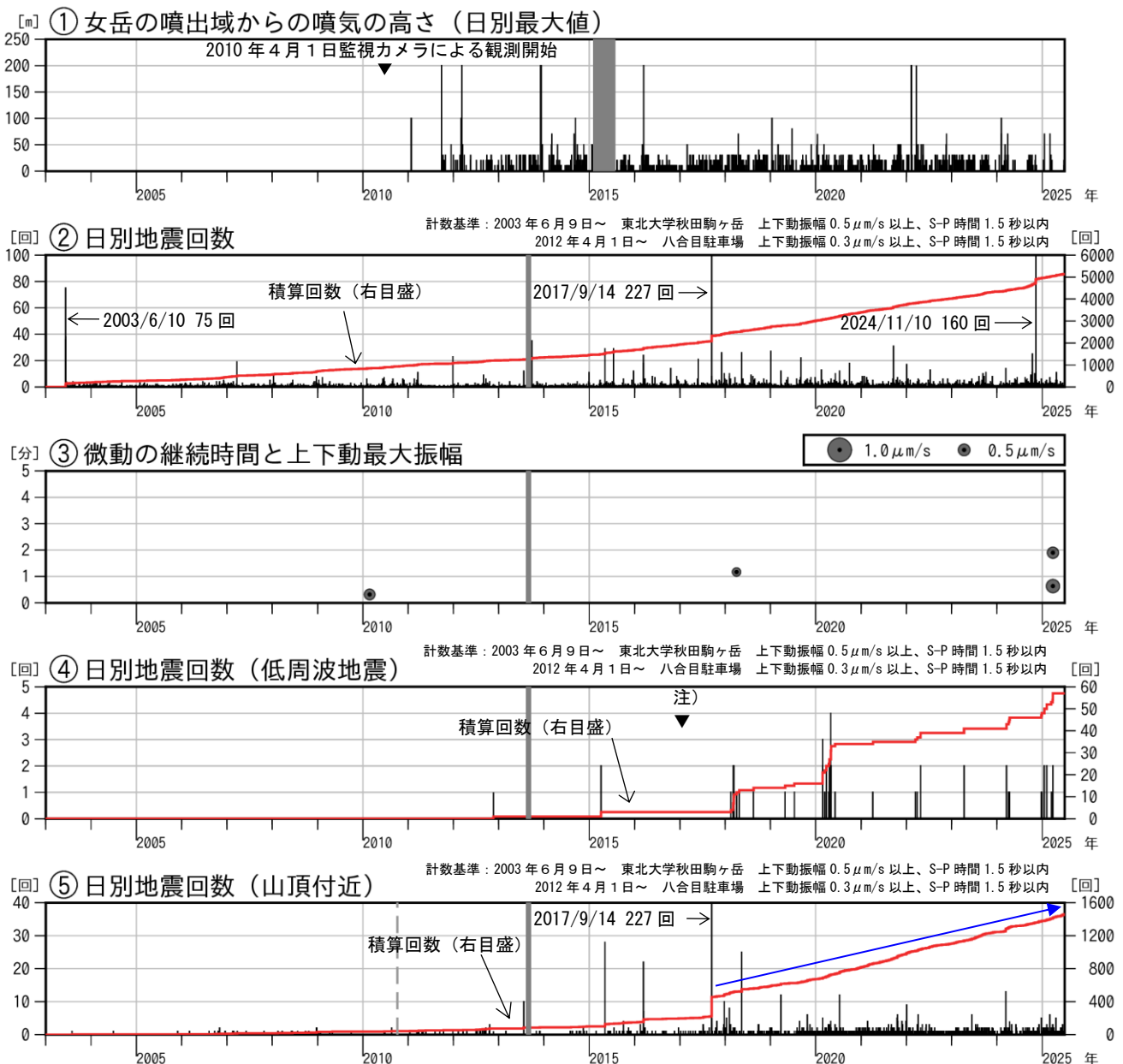
図 2 秋田駒ヶ岳 火山活動経過図（2003 年 6 月～2025 年 6 月）
