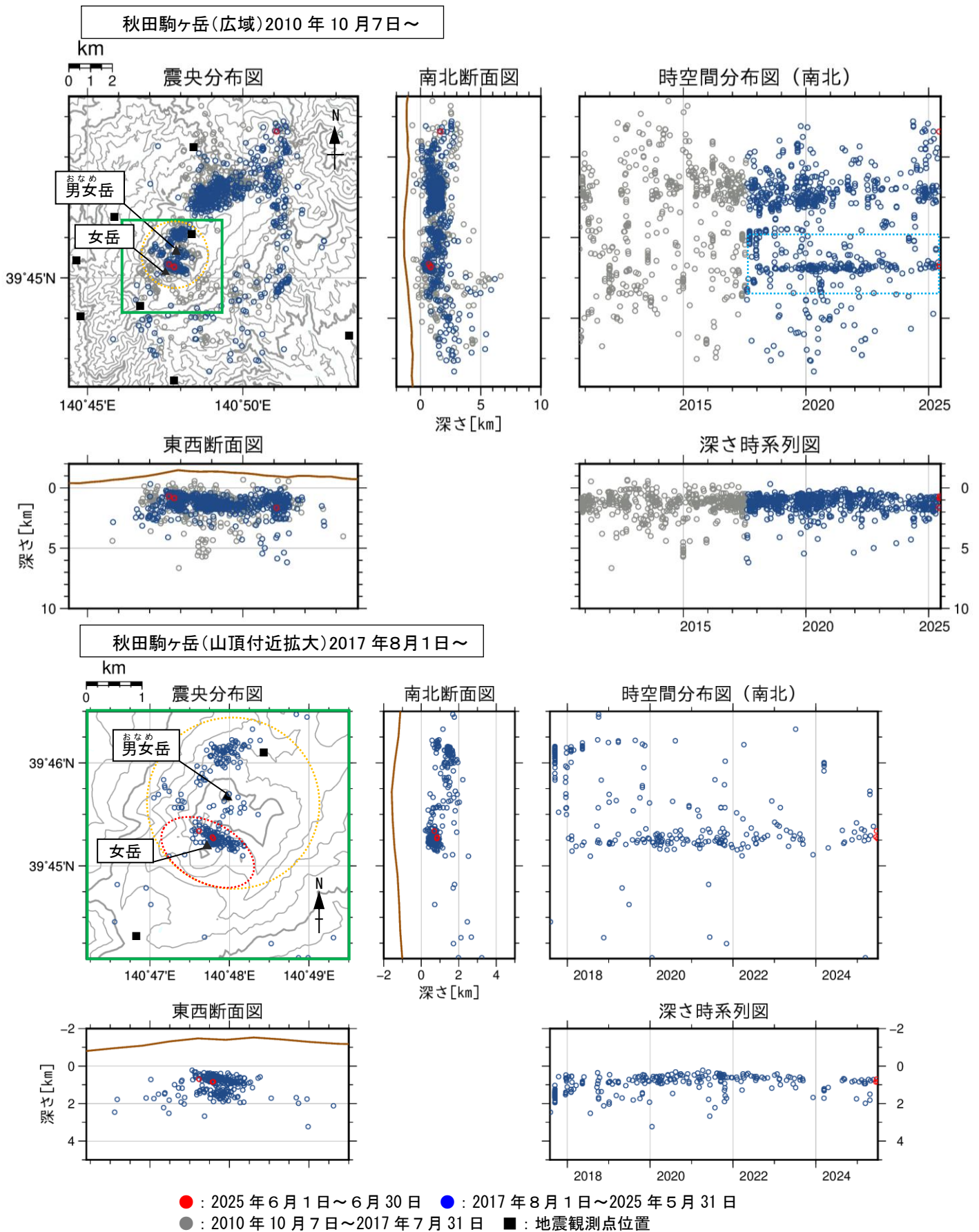
図4 秋田駒ヶ岳 地震活動（2010年10月7日～2025年6月）
