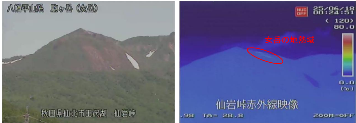
図1 秋田駒ヶ岳 女岳周辺の状況（6月13日）と地表面温度分布の状況（6月18日）
