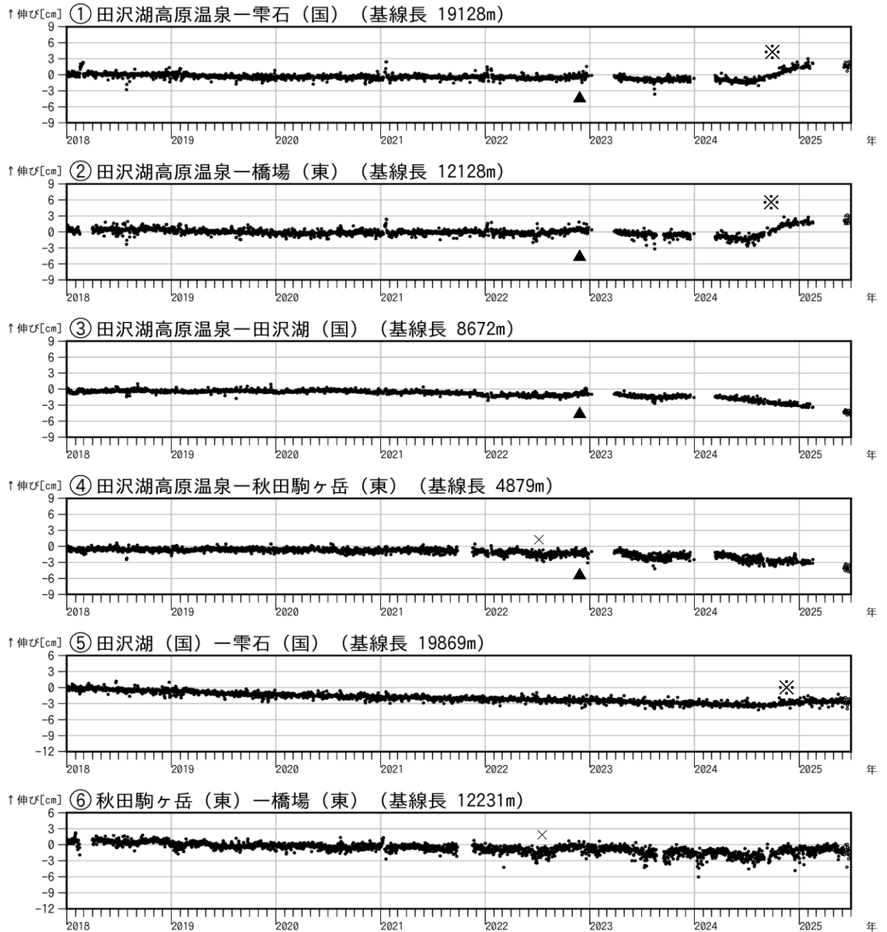
図5 秋田駒ヶ岳 GNSS 基線長変化図（2018年1月～2025年6月）
