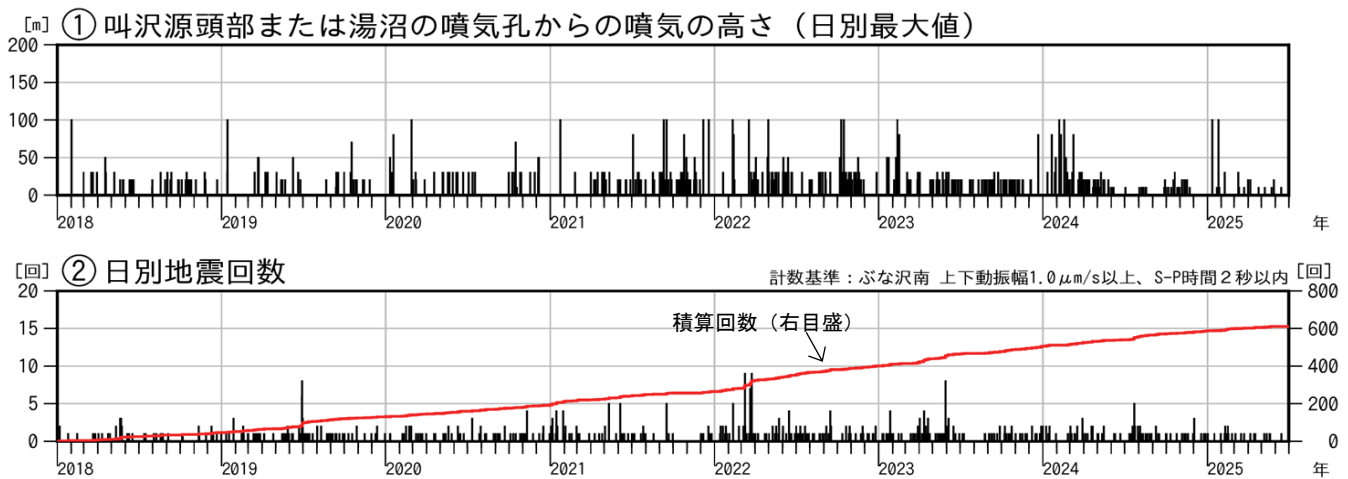
図3 秋田焼山 火山活動経過図（2018年1月～2025年6月）
