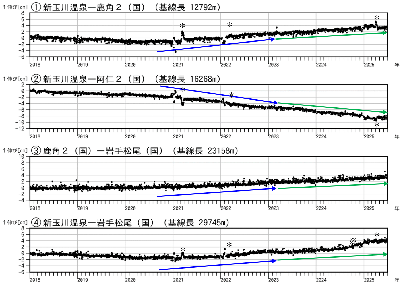
図4 秋田焼山 GNSS 基線長変化図（2018年1月～2025年6月）
