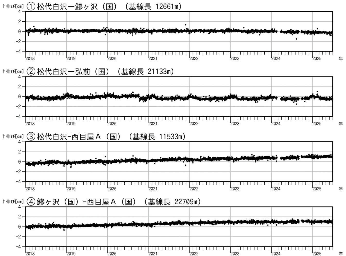
図3 岩木山 GNSS 基線長変化図（2018年1月～2025年6月）
