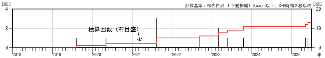
図2 岩木山 日別地震回数（2018年1月～2025年6月）
