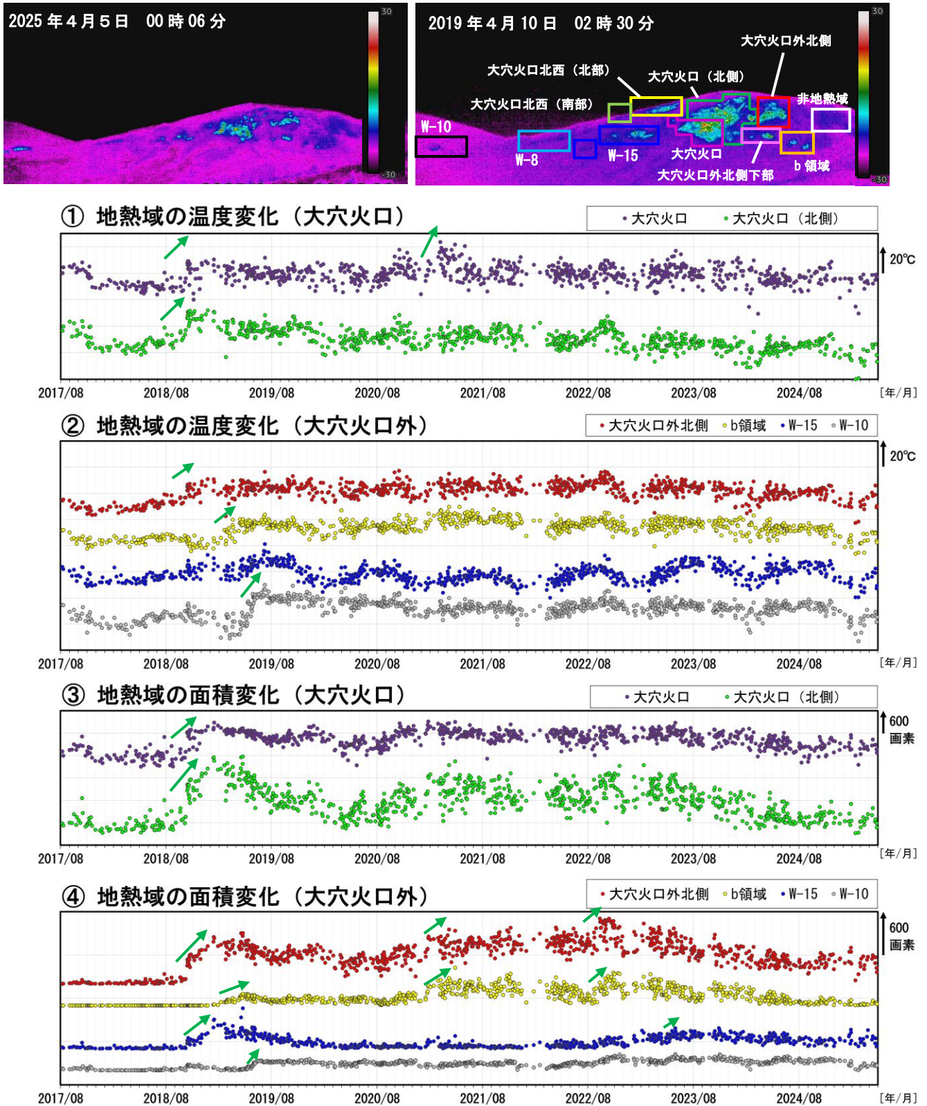
図5 吾妻山 監視カメラによる大穴火口周辺の地熱域の経過（2017年8月～2025年4月）
