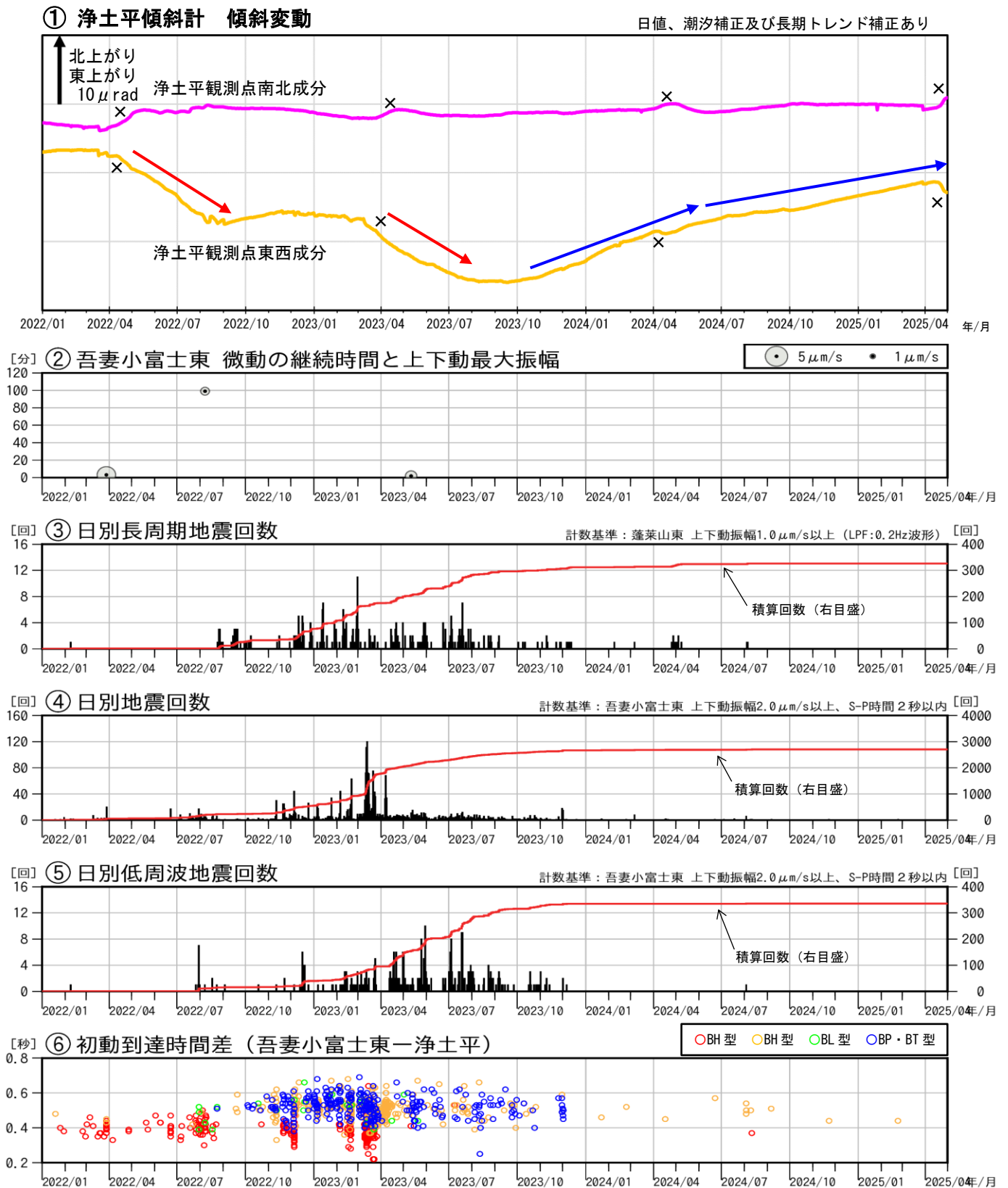
図3 吾妻山 火山活動経過図（2022年1月～2025年4月）
