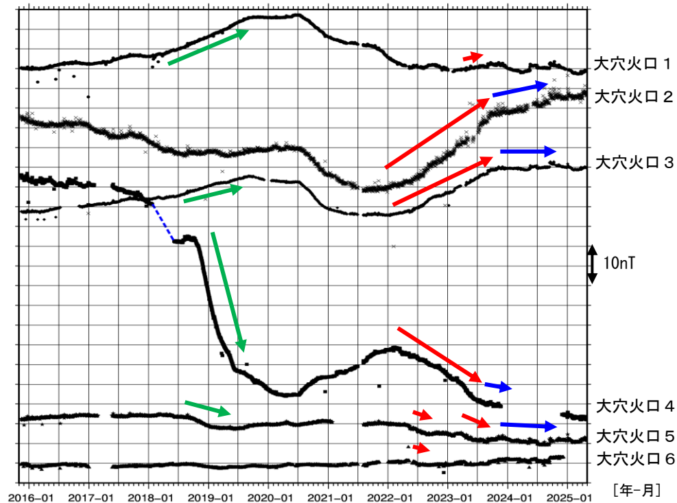
図7 吾妻山 全磁力連続観測点の全磁力値変化（2015年11月～2025年4月）
