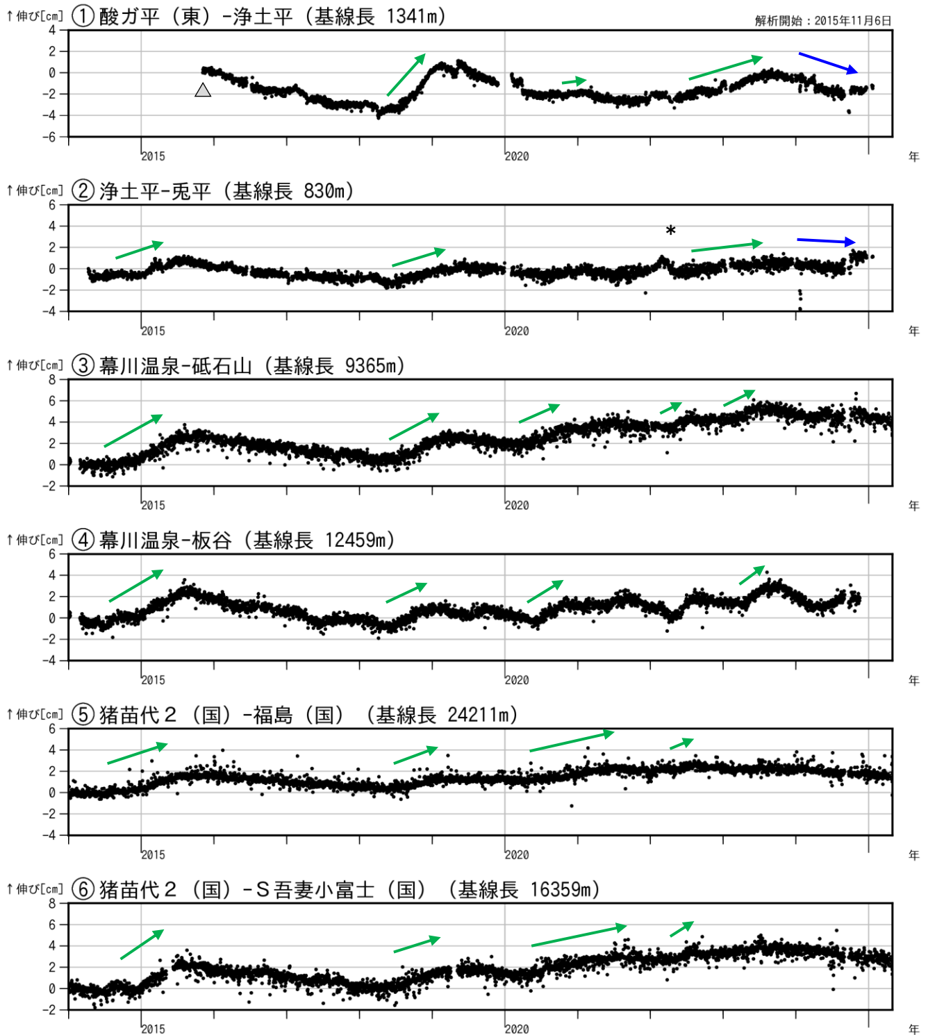
図4 吾妻山 吾妻山浅部・深部の地殻変動（2014年1月～2025年4月）
