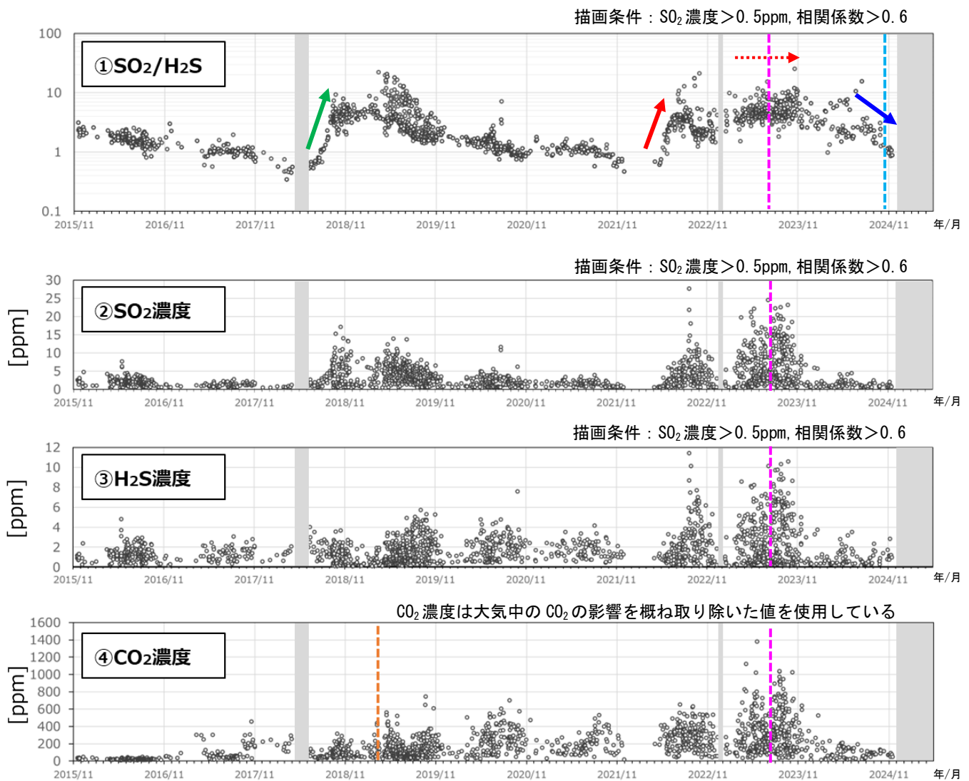
図6 吾妻山 火山ガス観測装置による観測（2015年11月～2025年4月）
