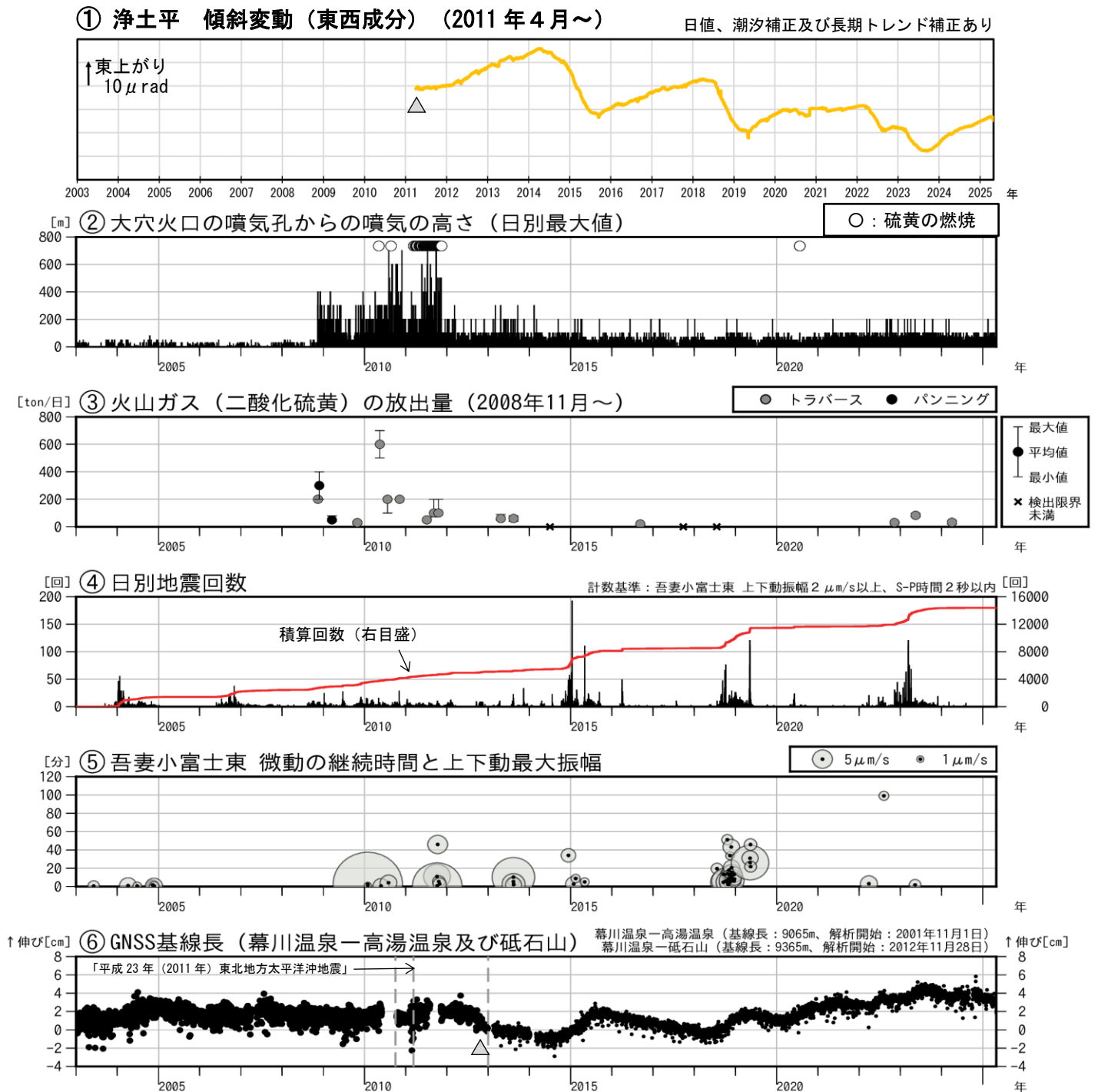
図2 吾妻山 中期的な火山活動の経過（2003年1月～2025年4月）
