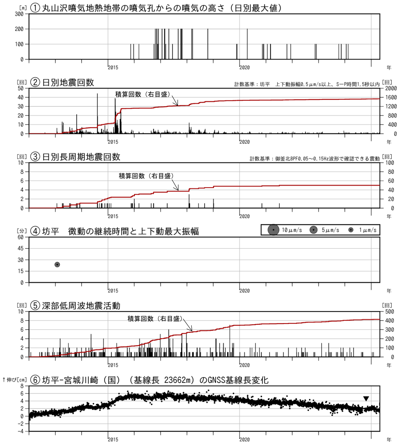
図2 蔵王山 火山活動経過図（2012年1月～2025年4月）
