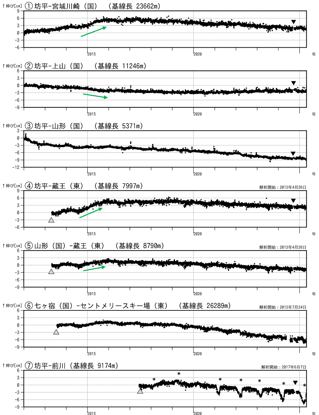
図3 蔵王山 GNSS 基線長変化図 (2012 年 1 月～2025 年 4 月)
