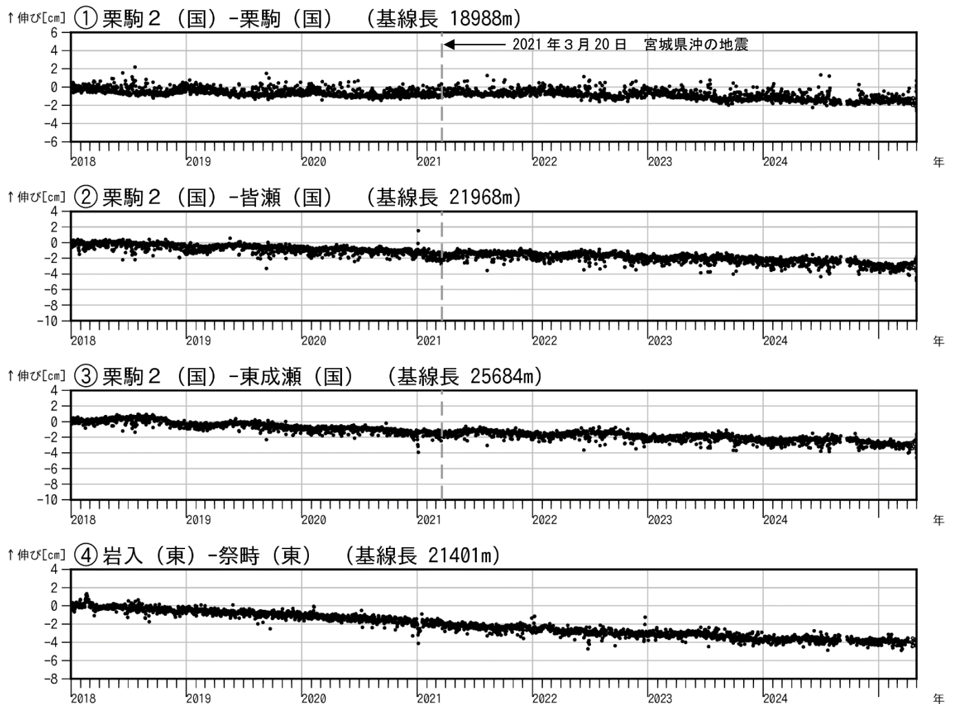
図3 栗駒山 GNSS 基線長変化図（2018年1月～2025年4月）
