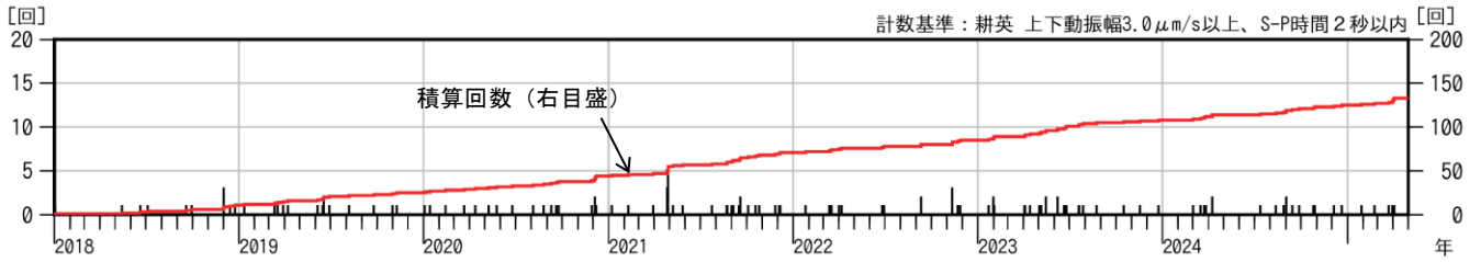
図2 栗駒山 日別地震回数（2018年1月～2025年4月）
