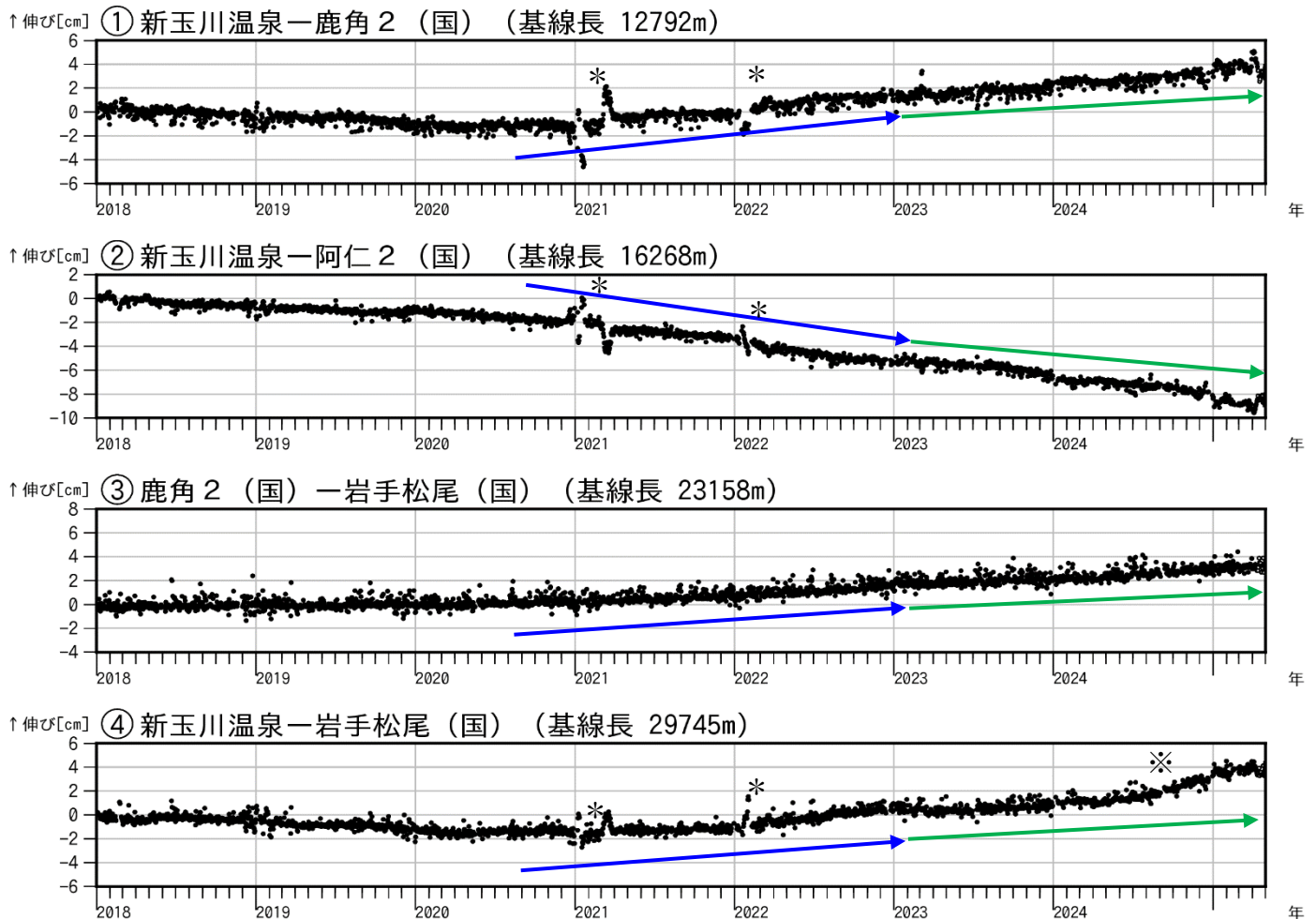
図4 秋田焼山 GNSS 基線長変化図（2018年1月～2025年4月）
