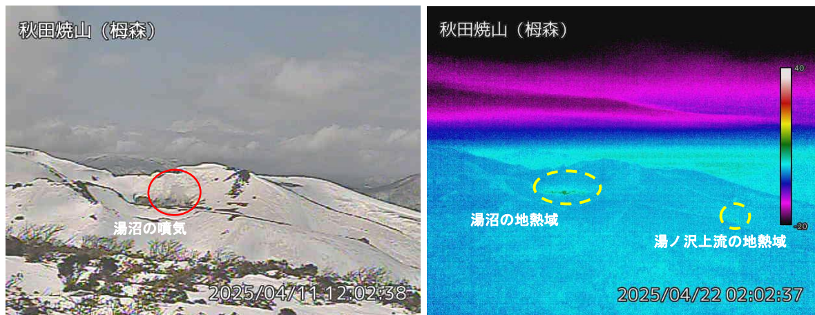
図2 秋田焼山 湯沼と湯ノ沢上流の状況（4月11日）と地表面温度分布（4月22日）
