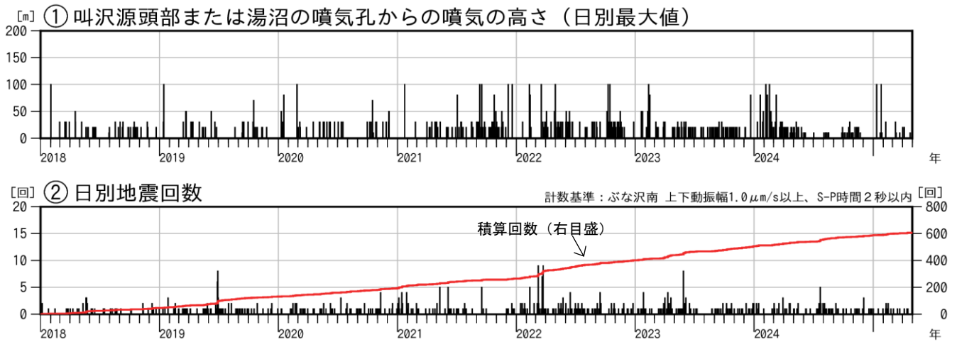
図3 秋田焼山 火山活動経過図（2018年1月～2025年4月）
