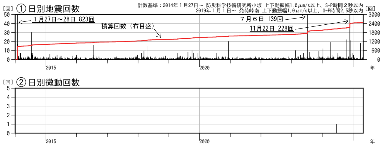
図2 十和田 活動経過図（2014年1月～2025年4月）
