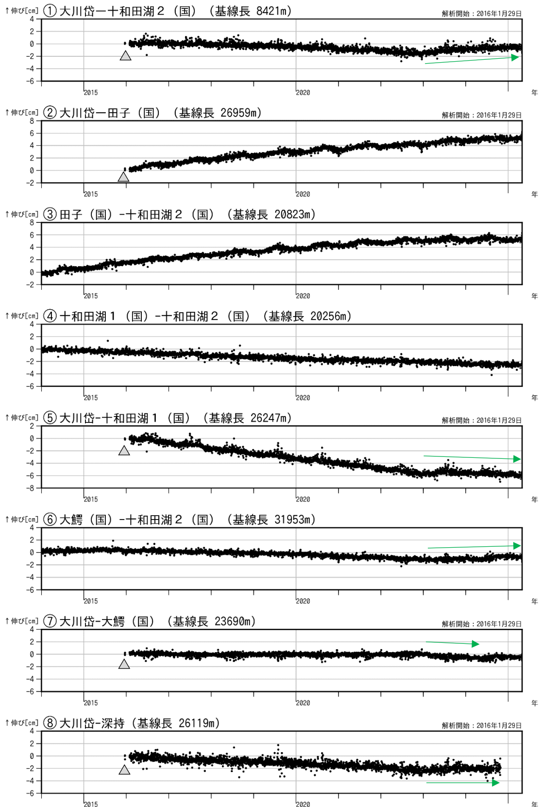
図3 十和田 GNSS 基線長変化図（2014年1月～2025年4月）
