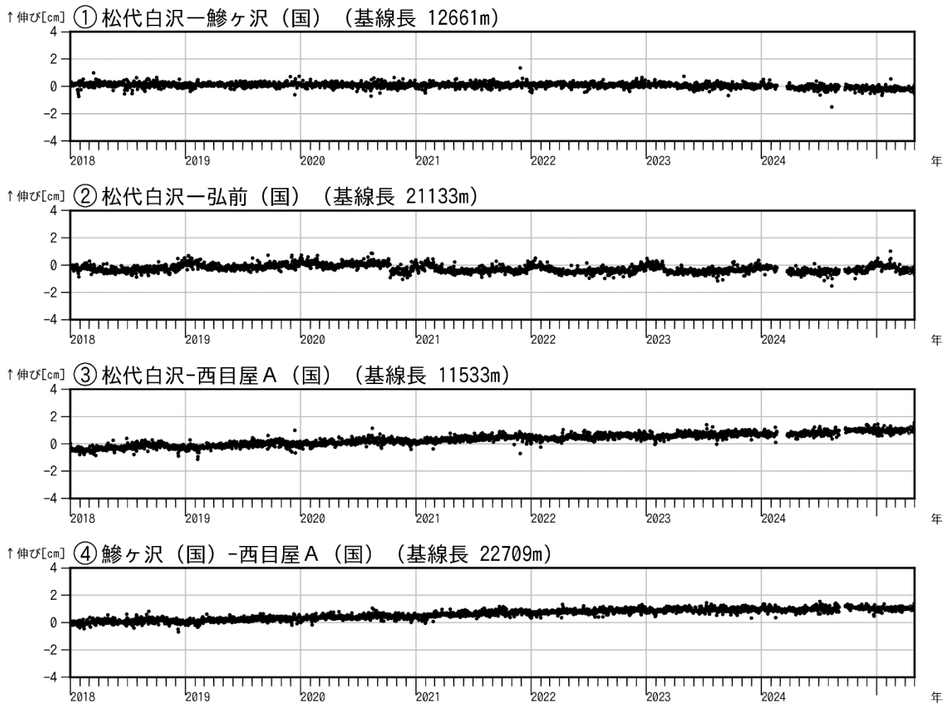
図3 岩木山 GNSS 基線長変化図（2018年1月～2025年4月）
