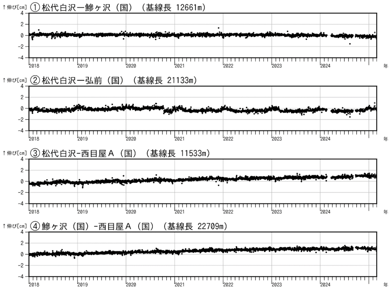
図3 岩木山 GNSS 基線長変化図（2018年1月～2025年2月）
