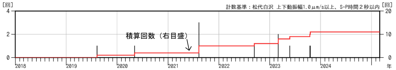
図2 岩木山 日別地震回数（2018年1月～2025年2月）
