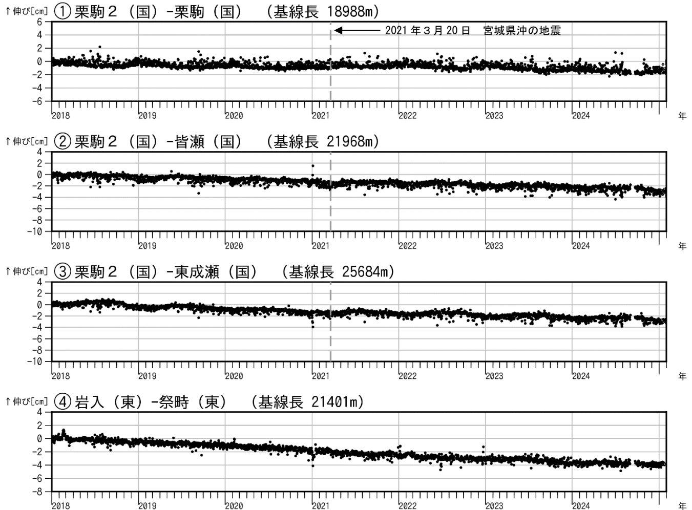
図3 栗駒山 GNSS 基線長変化図（2018年1月～2025年1月）
