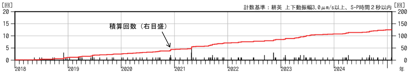
図2 栗駒山 日別地震回数（2018年1月～2025年1月）
